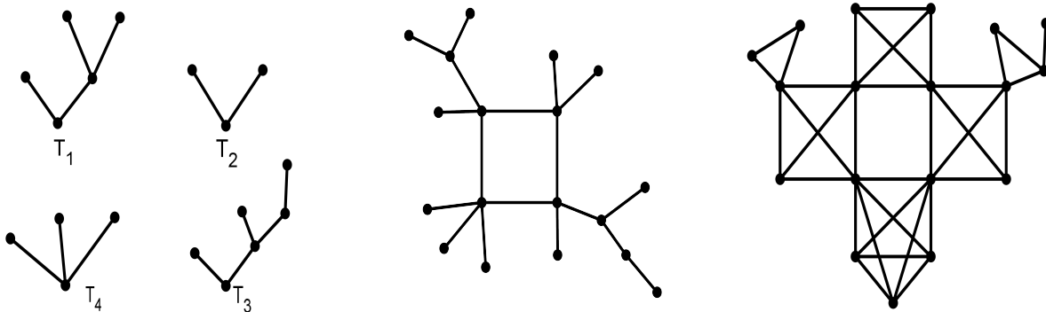
Figura 1: Los árboles T_1, T_2, T_3, T_4 , el grafo C_4(T_1, T_2, T_3, T_4) y su grafo de línea \mathcal{L}(C_4(T_1, T_2, T_3, T_4)) .
