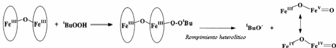
Figura 10. Esquema propuesto para la formación de especies activas entre d -FePcS y TBHP
