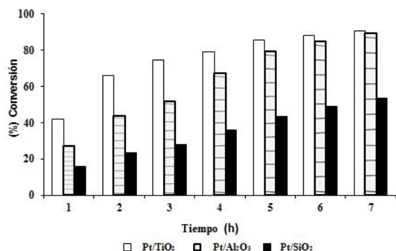
Figura 2. Nivel de conversión vs. tiempo en la hidrogenación de m -dinitrobenzono a 343 K y 0.82 MPa con catalizadores de platino soportado.
