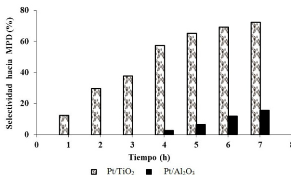
Figura 3. Nivel de selectividad hacia m -feniléndiamina en los catalizadores Pt/TiO 2 y Pt/Al 2 O 3 en el transcurso de la reacción.
