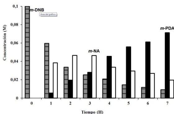
Figura 4. Concentraciones de reactivos y productos en el transcurso de la reacción con el catalizador Pt/TiO 2 .
