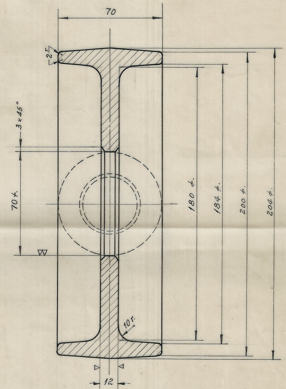
SECCION: A-A
