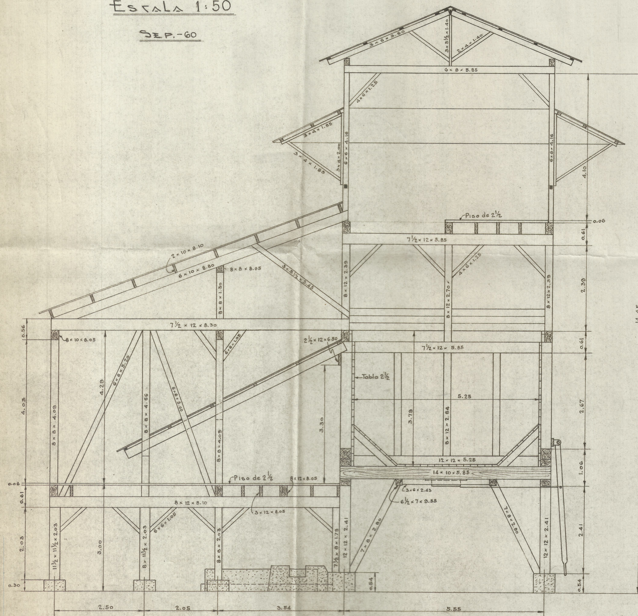
CORTE E-E
