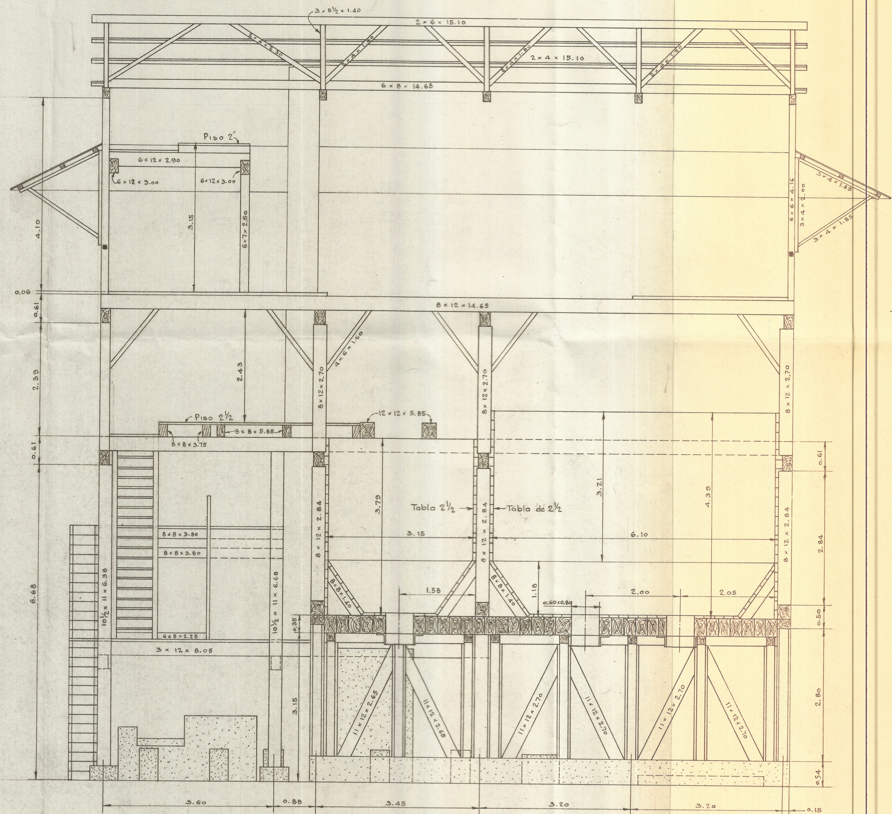
CORTE F-F
