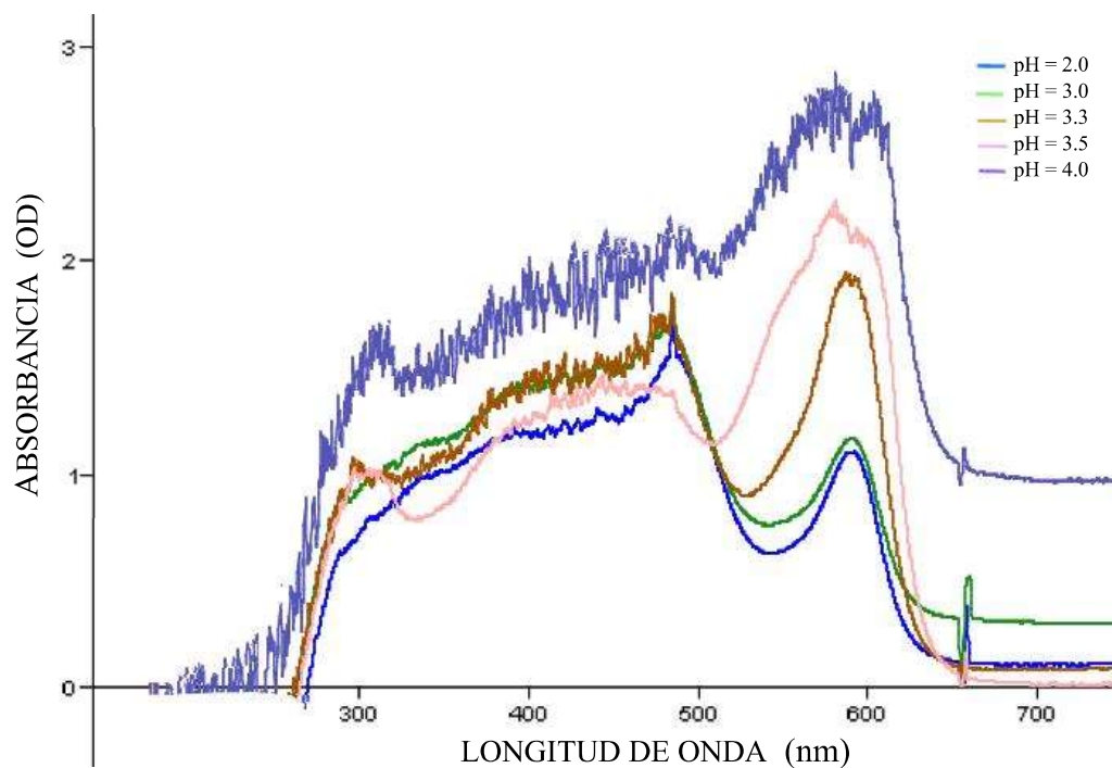
Figura 11. Espectros de absorbancia UV-Vis de soluciones buffer en el intervalo de pH 3.0–4.0 a 15 °C.
