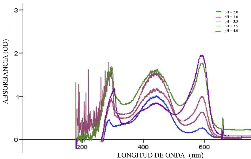
Figura 12. Espectros de absorbancia UV-Vis de soluciones buffer en el intervalo de pH 2.0–4.0 a 30 °C.
