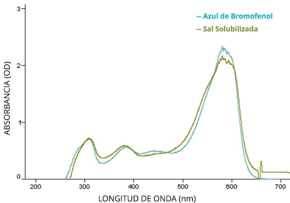
Figura 9. Espectros de absorbancia UV-Vis del indicador más la sal solubilizada luego de presurización.
