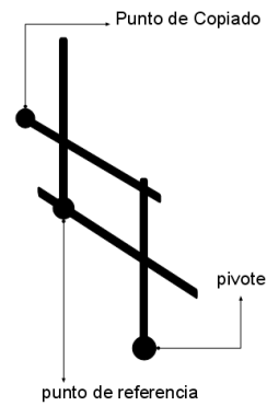
Figura 15. Pantógrafo
