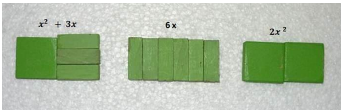
Fig.10. Representaciones de 2x^2 con Algebloks.
