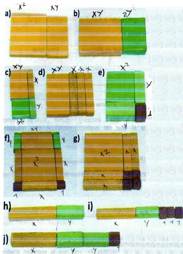
Fig.42 Desarrollo de la técnica \tau_{1d}
