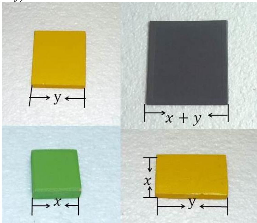
Fig.5 Bloques Algebloks: Dos dimensiones.
