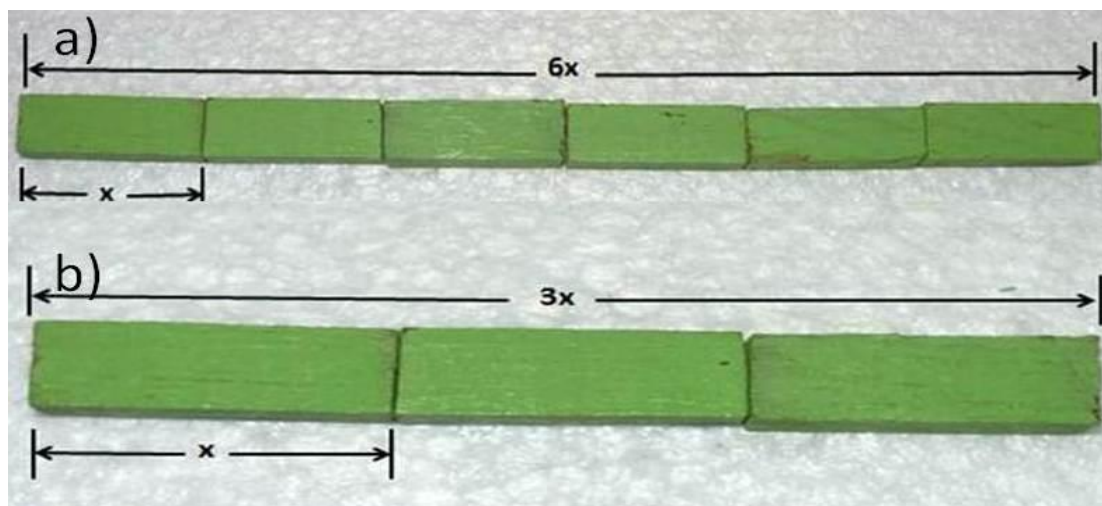
Fig.12. Distancias 6x y 3x .
