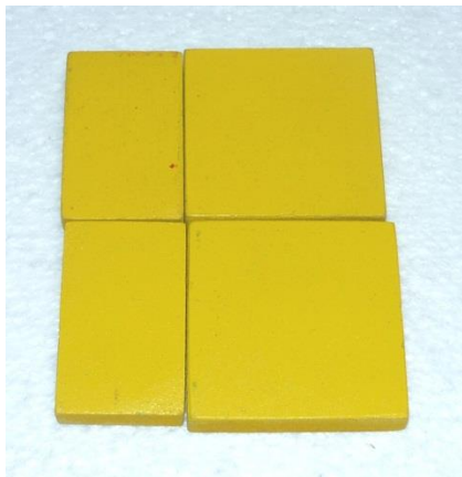
Fig.17 Superficie con Algebloks.
