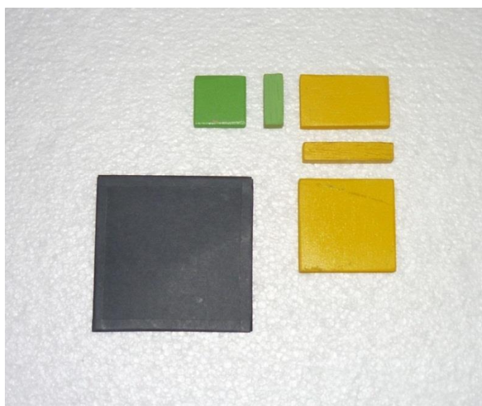
Fig.6 Bloques Algebloks: Una y dos dimensiones.
