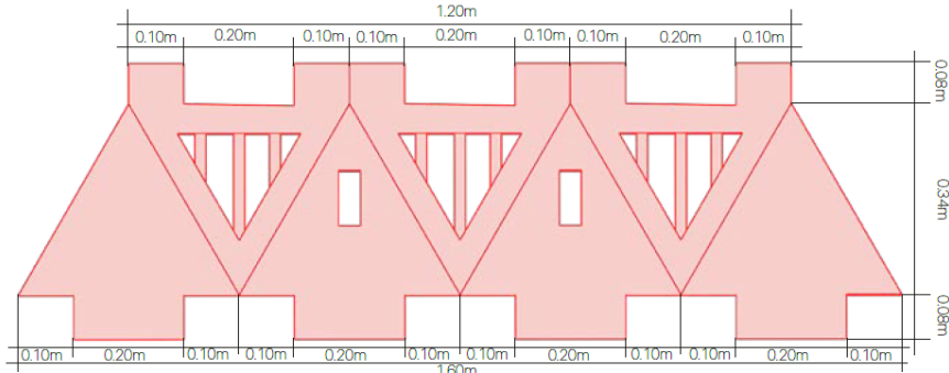
PLANTA EXTREMO "B" ESC 10
