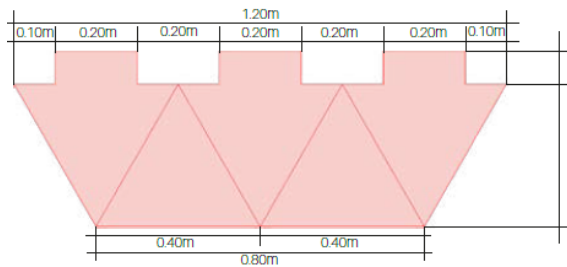
PLANTA EXTREMO "D" ESC 10
