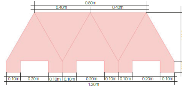
PLANTA EXTREMO "A" ESC 10
