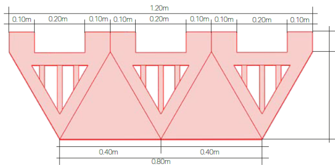
PLANTA EXTREMO "D" ESC 10
