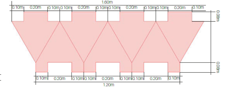
PLANTA EXTREMO "C" ESC 10
