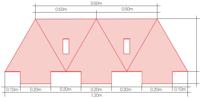
PLANTA EXTREMO "A" ESC 10
