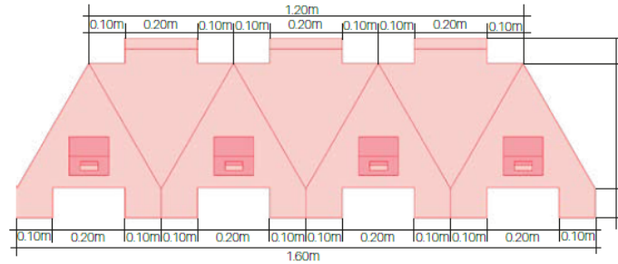
VISTA POSTERIOR EXTREMO "B" ESC 10
