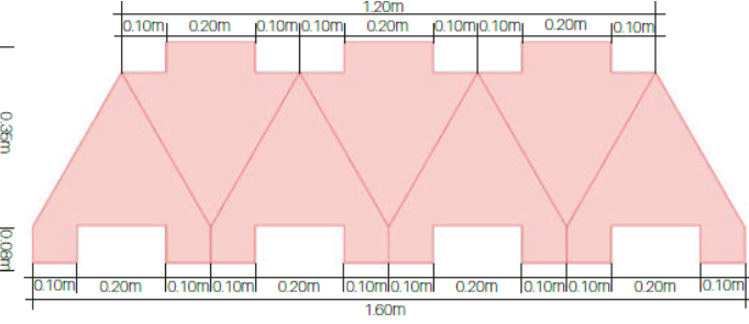
PLANTA EXTREMO "B" ESC 10
