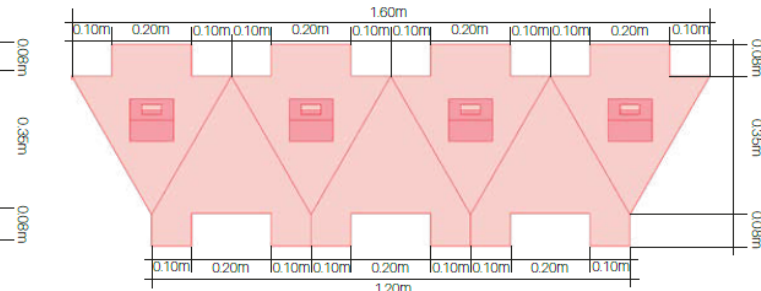
VISTA POSTERIOR EXTREMO "C" ESC 10
