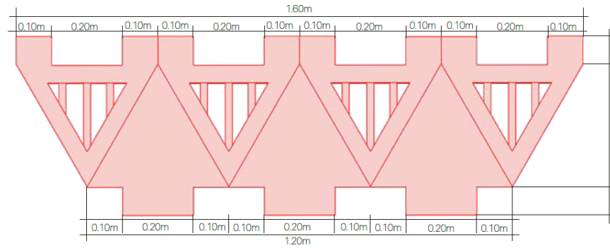
PLANTA EXTREMO "C" ESC 10
