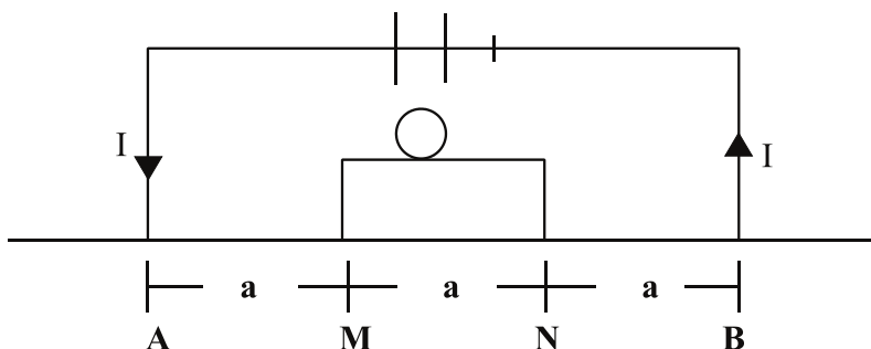
Figura 3. Configuración de un dispositivo de cuatro electrodos para estudios de prospección arqueológica.
