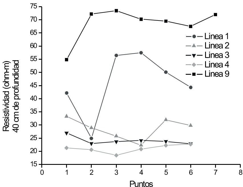
Figura 57. Resistividad en el suelo enterrado a 40 cm. de profundidad.
