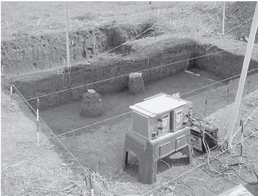
Figura 4. Dispositivo de geoelectrica (Resistivímetro) para mediciones en campo.
