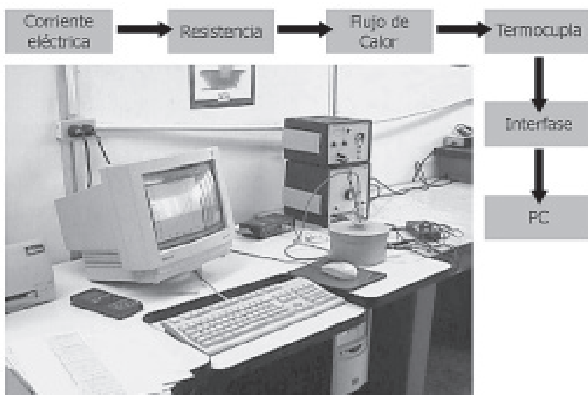
Figura 39. Montaje para evaluar la conductividad térmica del suelo.
