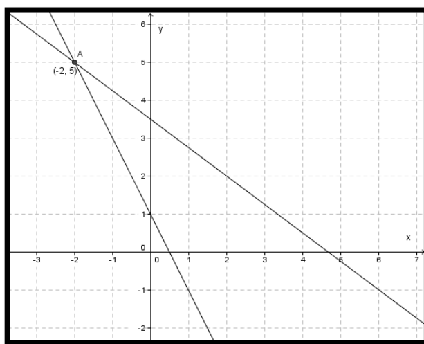
Figura 1. Representación cartesiana de dos rectas que se cortan en un mismo punto.
