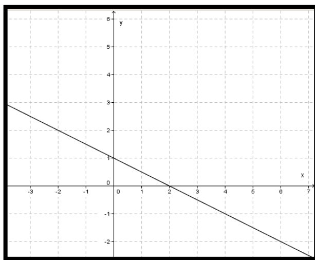
Figura 2. Representación cartesiana de dos rectas que coinciden en todos sus puntos.
