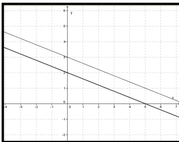
Figura 3. Representación cartesiana de dos rectas paralelas.
