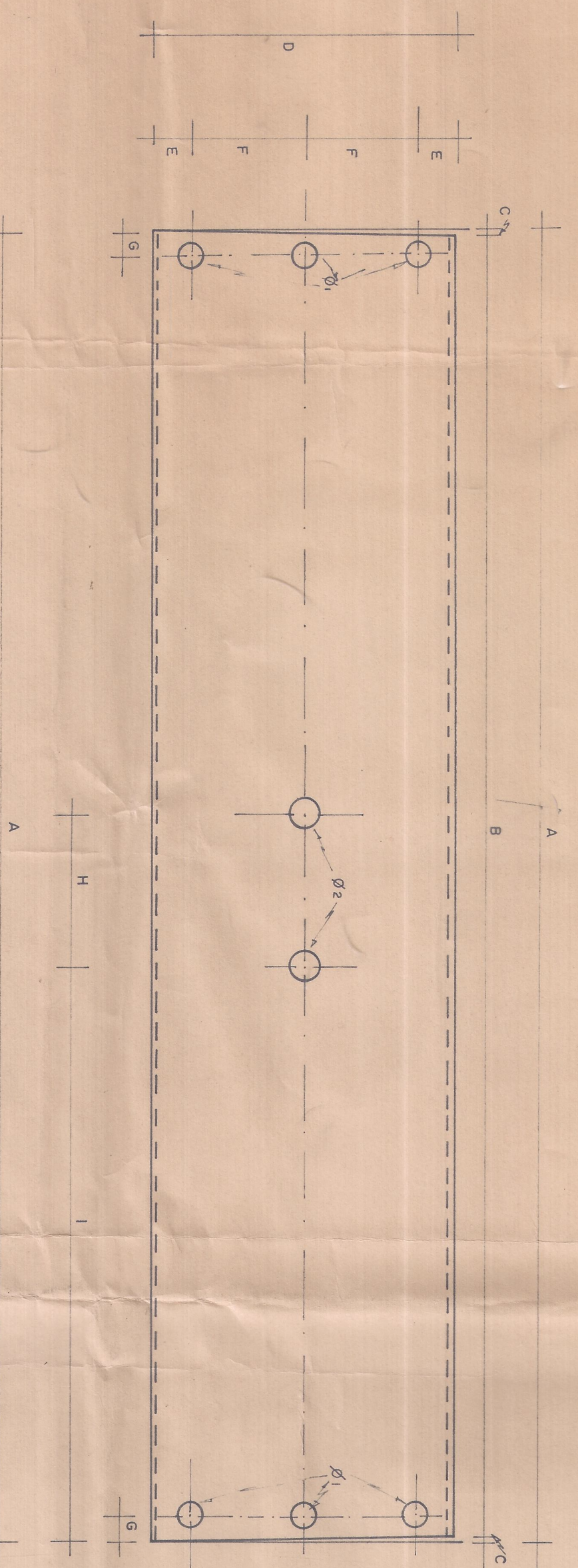
SECCION DE SEPARACION PARA I-II-III y IV ALUMINIO SEMI-DURO de 2 Mm. CANTIDAD = 2 X SECCION VER TABLA N° 2
