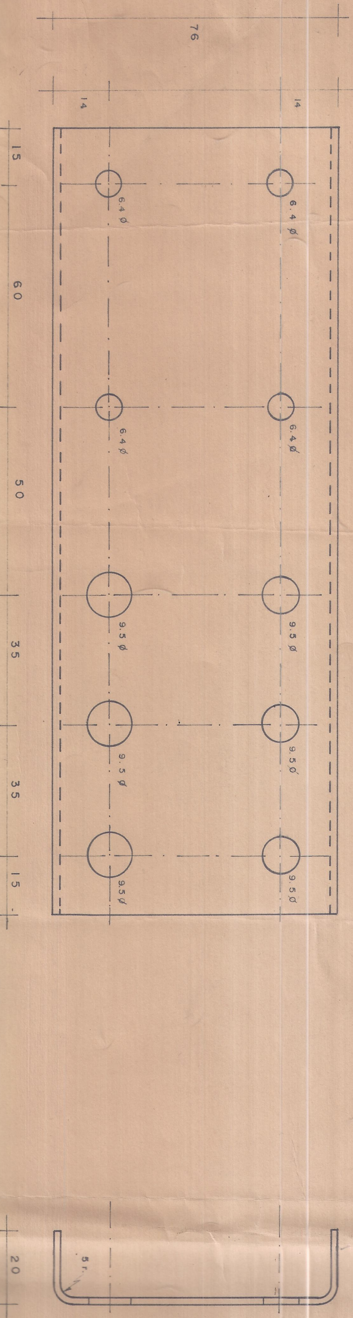
SECCION DE SEPARACION PARA V y VI ALUMINIO SEMI-DURO de 2 Mm. CANTIDAD = 2 X SECCION
