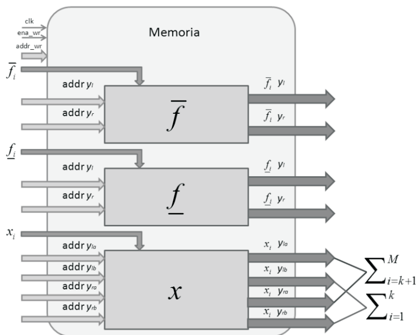
Figura 9. Configuración de la memoria.
