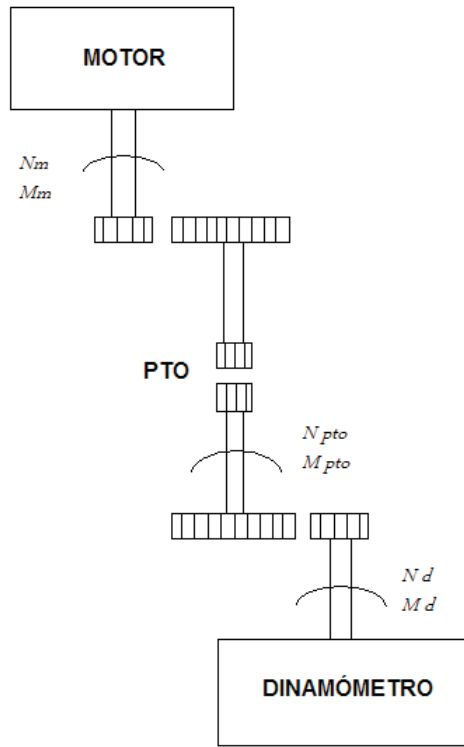
Figura 1. Esquema del sistema de transmisión
