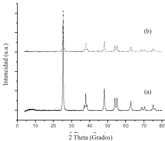
Figura 3. Análisis DRX de compuestos (a) \text{TiO}_2 (b) \text{TiO}_2 -Au
