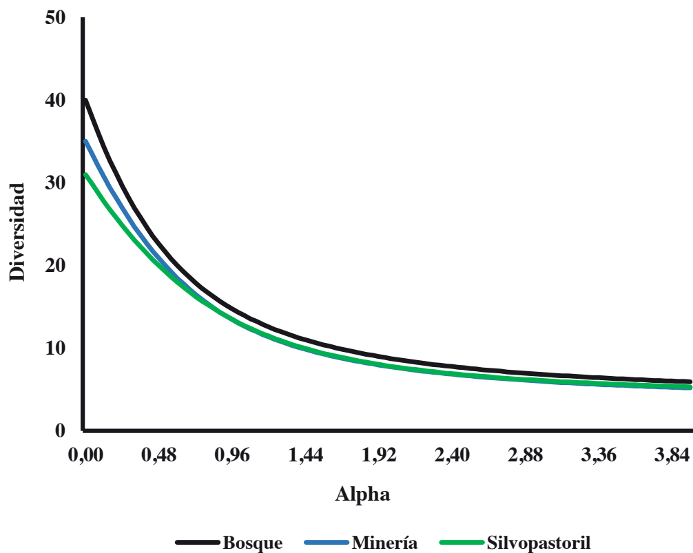
Figura 3. Perfiles de diversidad de Renyi para las tres zonas de estudio en el río Purnio.
