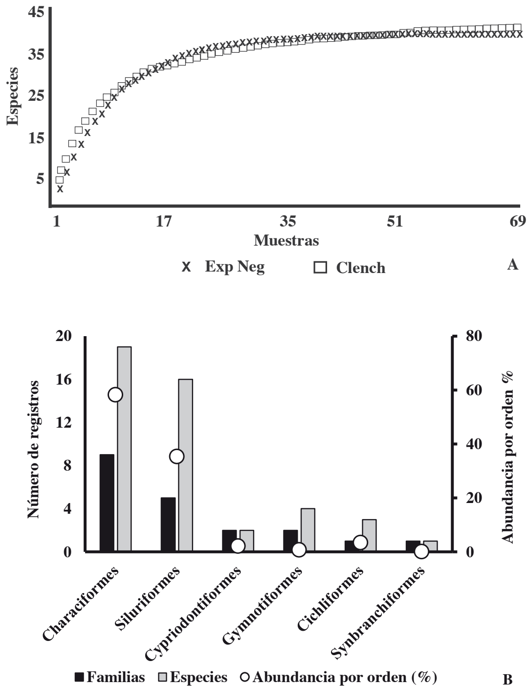
Figura 1. A. Curvas de acumulación de especies ajustadas de acuerdo a los modelos exponencial negativo y Clench. B. Número de familias y especies de peces de cada orden registradas en la zona de estudio y proporción de contribución a la abundancia.
