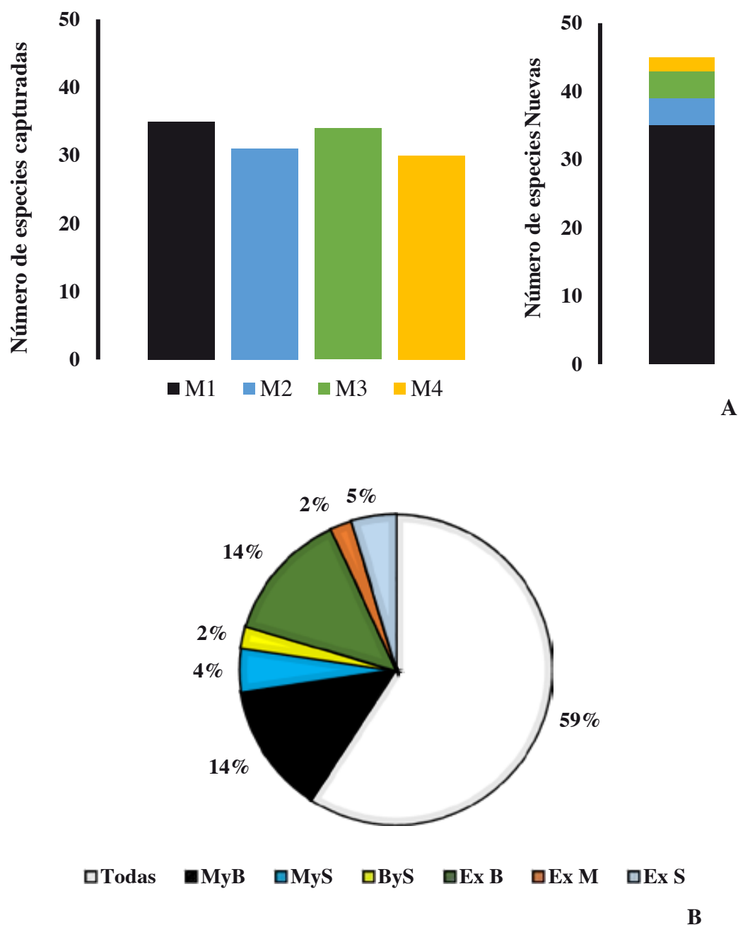
Figura 2. A. Especies capturadas por muestreo y especies nuevas adicionadas durante cada uno de los eventos de muestreo: M1: muestreo 1, M2: muestreo 2, M3: muestreo 3, M4: muestreo 4. B. Proporción de especies exclusivas y compartidas considerando las diferentes zonas de estudio. MyB: minería y bosque, MyS: minería y silvopastoril, ByS: bosque y silvopastoril, Ex B: exclusivas Bosque, Ex M: exclusivas minería, Ex S: exclusivas silvopastoril.
