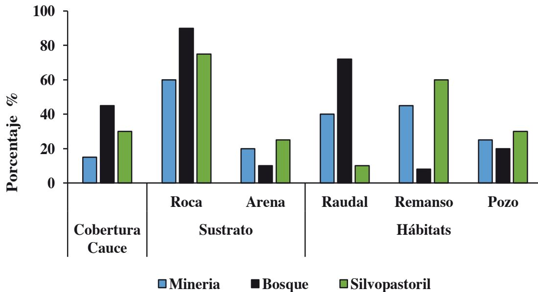
Figura 5. Porcentaje de Cobertura del cauce, composición del sustrato y tipo de hábitat considerando la velocidad y profundidad del agua en las tres zonas de estudio del río Purnio.
