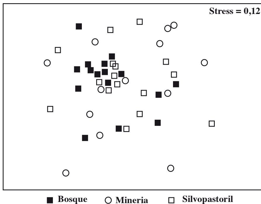
Figura 4. Ordenamiento no métrico multidimensional del ensamble íctico en el río Purnio considerando las tres zonas de estudio.
