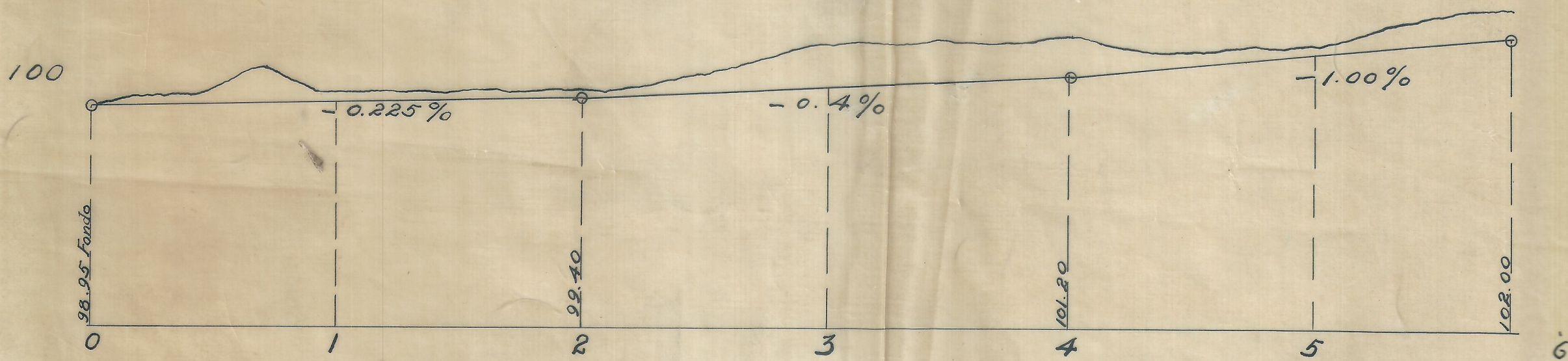
SECCION DEL CANAL Esc. 1/25
