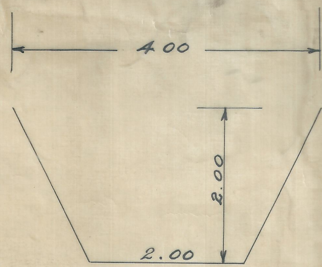
SECCION DEL CANAL Esc. 1/25
