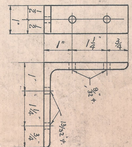
DETALLE N°: 9 CANTIDAD: 2 MATERIAL: Ang. de 3" x 3" x 1/8" x 1
