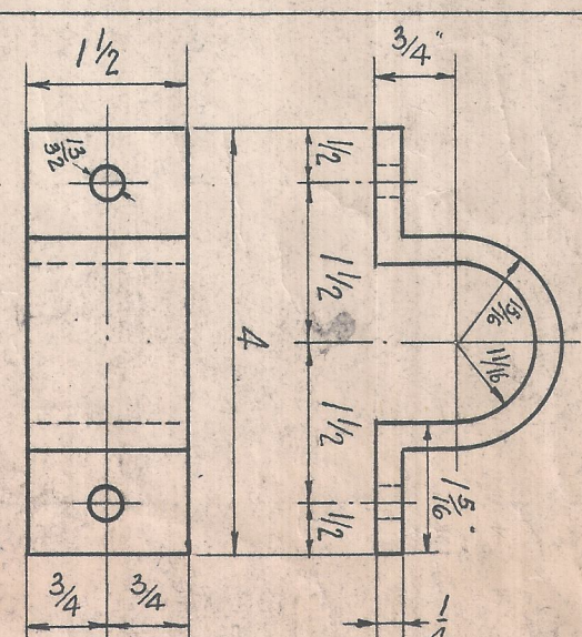
DETALLE N°: 11 CANTIDAD: 4 MATERIAL: Plat 1/4 x 1 1/2 x 6 5/16
