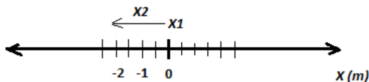
Figura 6. Vectores posición en una dimensión.
