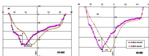
Figura 4. Resultados obtenidos del desplazamiento de la sección del cauce esperados con el modelo BVANE (Odgaard, 1996), para dos de las secciones utilizadas en el diseño: KD+650 y KD+880.
