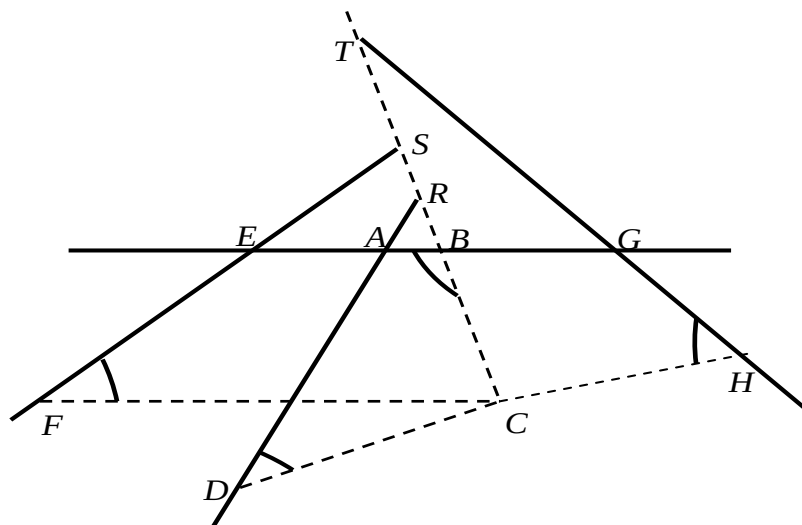
FIGURA 2.4 EL PROBLEMA DE PAPPUS
