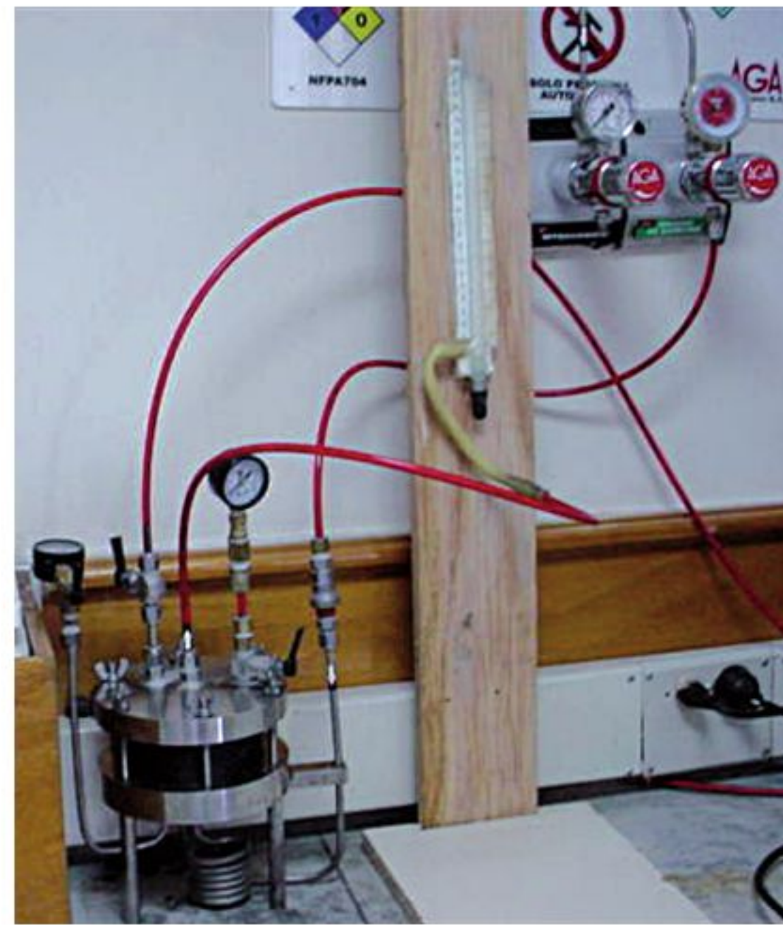
Fig. 2.1. Celda de permeabilidad y conexiones del suministro de gas
