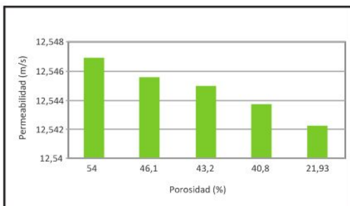
Figuras 4.8 y 4.9. Permeabilidad al CO 2 de diferentes coques a la misma granulometría (>6,3 mm) vs. la porosidad por (MEB) y por (ISO)
