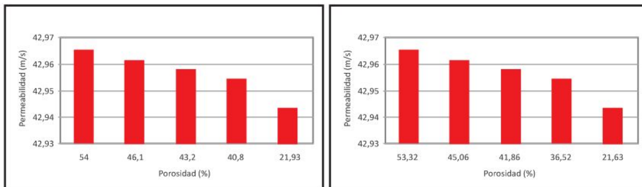
Figuras 4.6 y 4.7. Permeabilidad al N 2 de diferentes coques a la misma granulometría (>6,3 mm) vs. la porosidad por (MEB) y por (ISO)
