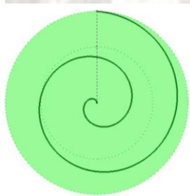
Figura 31. Espiral Arquimédica.
