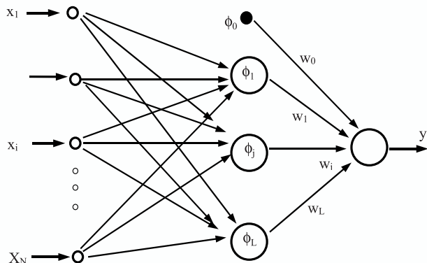
Fig. 6.5 Arquitectura de una red RBF
