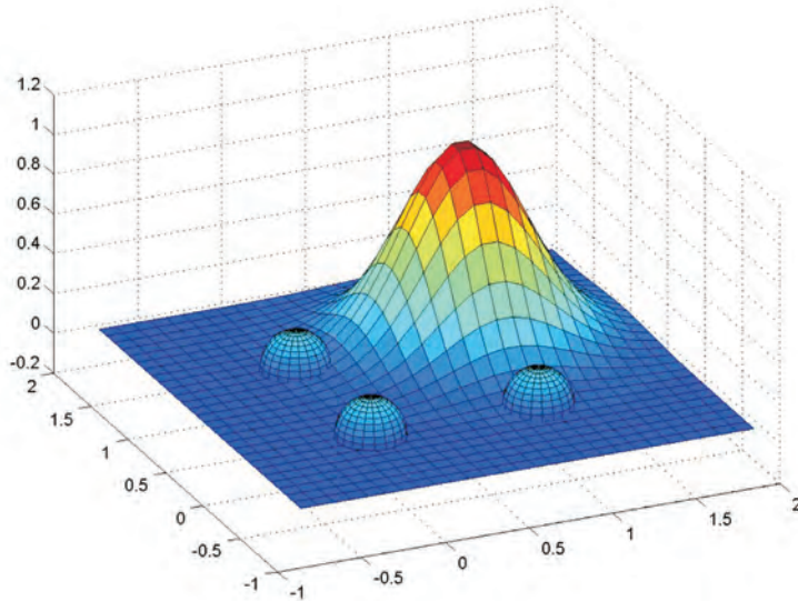
Fig. 6.11 Solución de la función AND con una red tipo RBF
