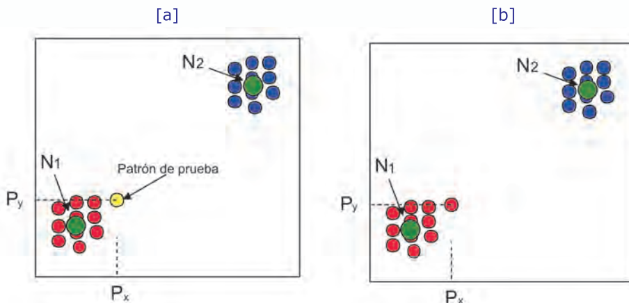
Fig. 5.11 Principio de Funcionamiento del Mapa de Kohonen
