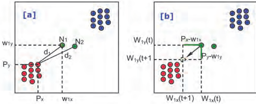
Fig. 5.6 Ilustración del algoritmo de entrenamiento de los SOM
