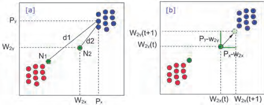
Figura 5.7 Ilustración del algoritmo de entrenamiento de los SOM
