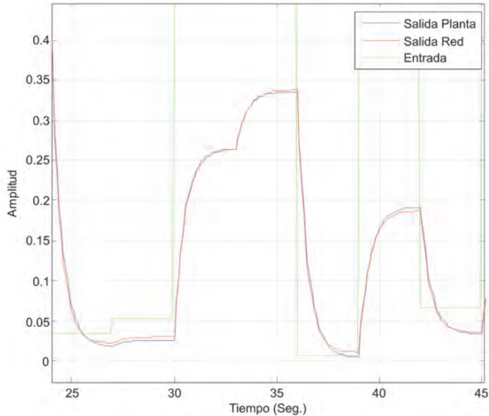
Fig. 6.23 Validación del modelo obtenido
