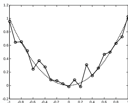
Fig. 3.5 Sobre-entrenamiento en una Red Neuronal Artificial
