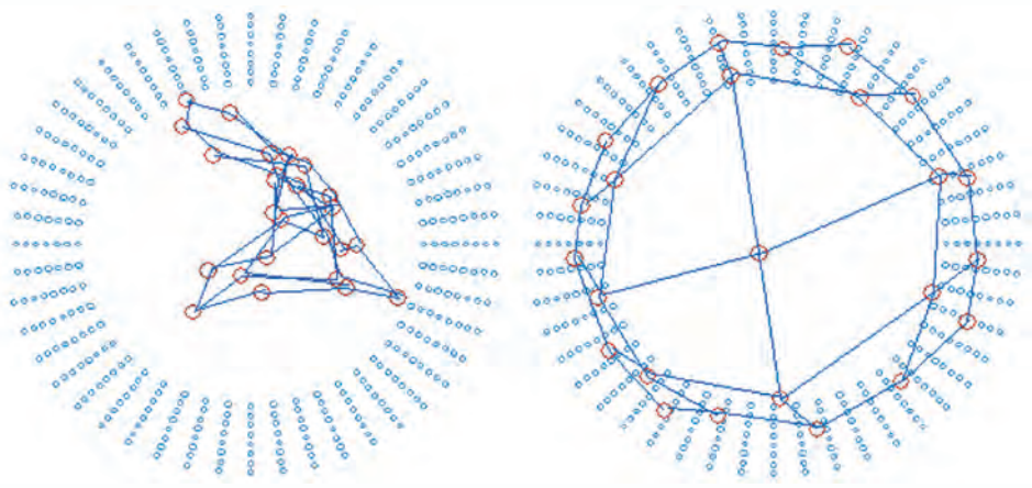
Fig. 5.10 Capacidad de auto-organización de los Mapas de Kohonen (Caso Toroide)
