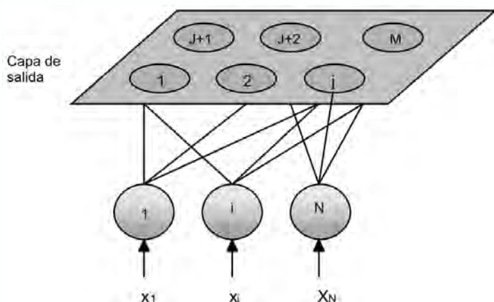
Fig. 5.3 Arquitectura de una red en dos dimensiones
