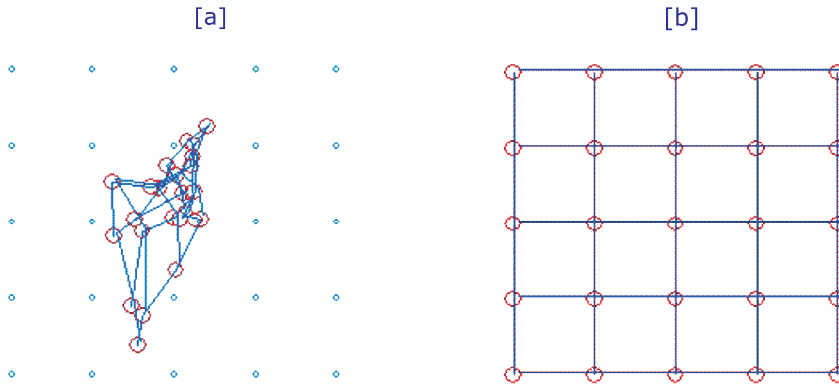
Fig. 5.9 Capacidad de auto-organización de los Mapas de Kohonen (Caso Cuadrícula)
