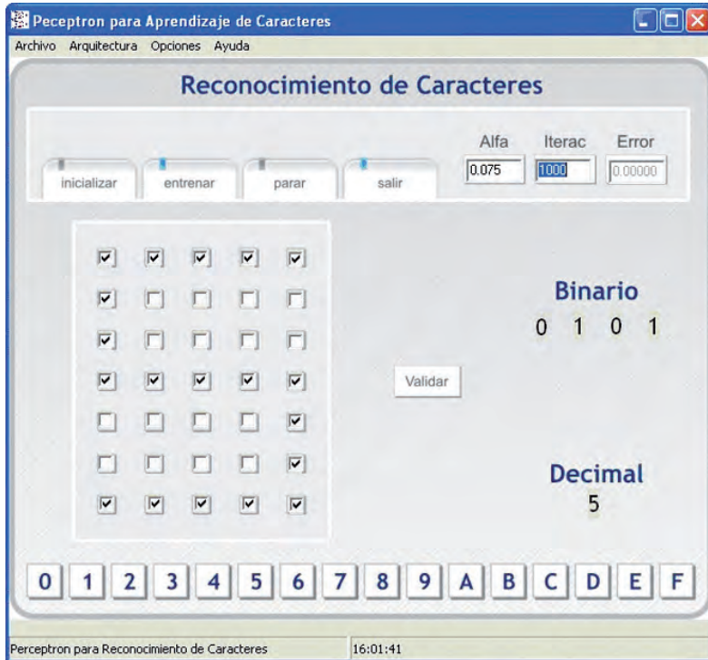
Fig. 2.23 Interfaz de Usuario del Módulo de Reconocimiento de Caracteres de UVSRNA
