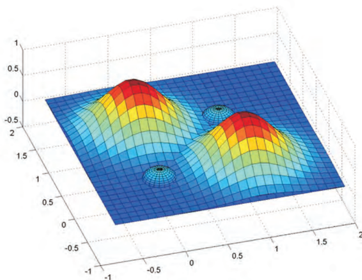
Fig. 6.13 Solución de la función XOR con una red tipo RBF
