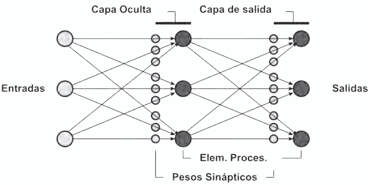
Figura 2.9 Estructura de una Red Neuronal Multicapa
