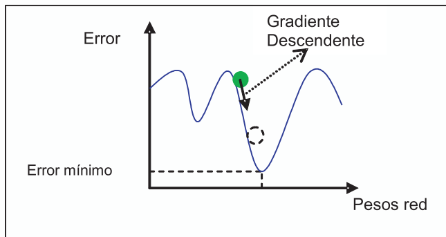
Fig. 2.7 Gradiente Descendente
