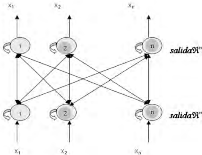
Fig. 4.2 Memoria Autoasociativa
