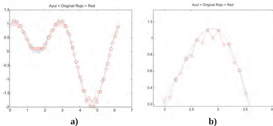
Fig. 6.18 a) Interpolación cuando la desviación estándar es baja b) Acercamiento para visualizar el sobre-entrenamiento
