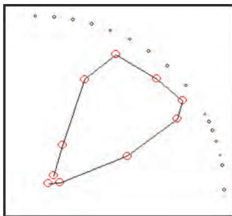
Fig. 5.18 Avance del Entrenamiento con 10 iteraciones
