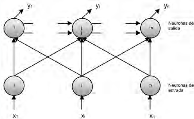
Fig. 5.2 Arquitectura de una red simple de Kohonen
