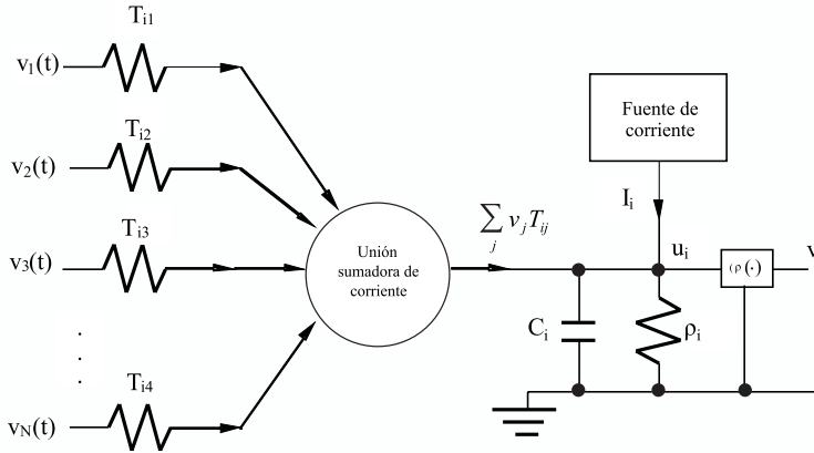
Fig. 4.5 Modelo Continuo de Hopfield de una Neurona
