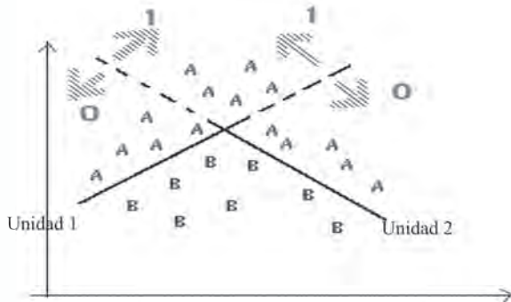
Fig. 2.8 Regiones de separación lineal que genera un Perceptron
