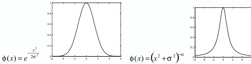
Fig. 6.4 Funciones Base Radial
