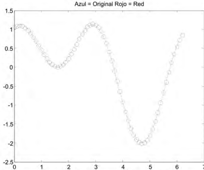
Fig. 6.16 Patrones de entrenamiento y Salida de validación de la Red (des=1)
