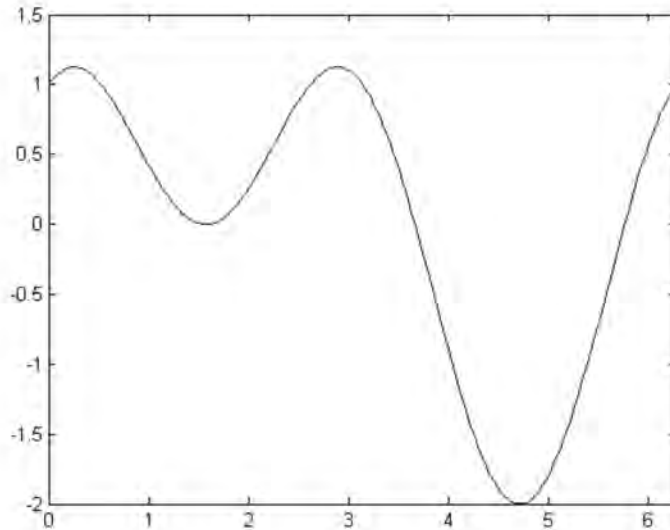
Fig. 6.15 Función a Aproximar con la red tipo RBF
