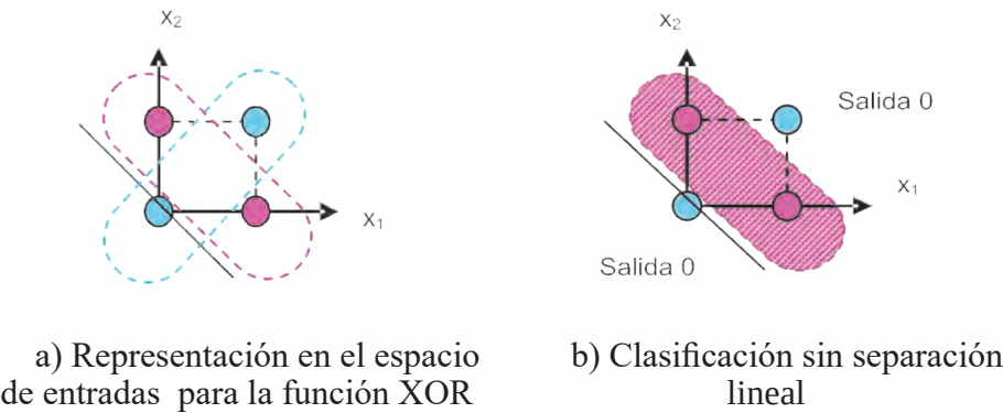
Fig. 2.10 Solución de la XOR con un Perceptron
