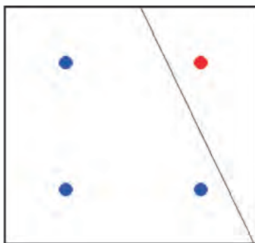
Fig. 6.9 Solución de la función AND con un Perceptron
