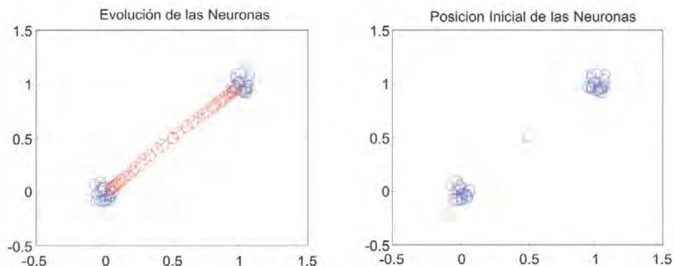
Fig. 5.12 Clasificación de Patrones usando un Mapa de Kohonen
