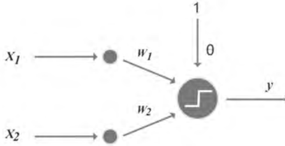
Fig. 2.2 Perceptron para trabajar puntos en dos dimensiones
