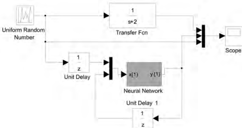
Fig. 6.22 Esquema en Simulink para validar el modelo
