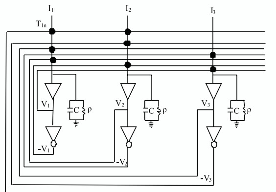
Fig. 4.4 Modelo Continuo de Hopfield
