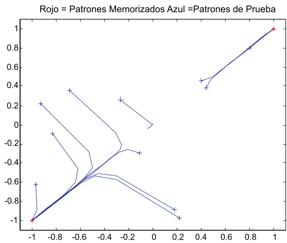
Fig. 4.8 Visualización de la evolución de la salida de la red ante diferentes patrones de entrada
