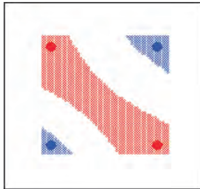
Fig. 6.12 Solución de la función XOR con una red tipo MLP
