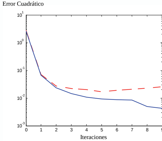
Fig. 3.7 Regularización por Parada Temprana
