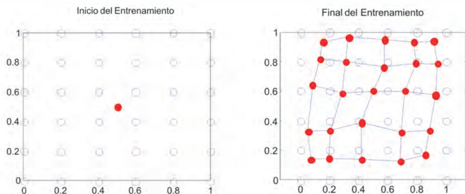
Fig. 5.14 Resultado del proceso de aprendizaje
