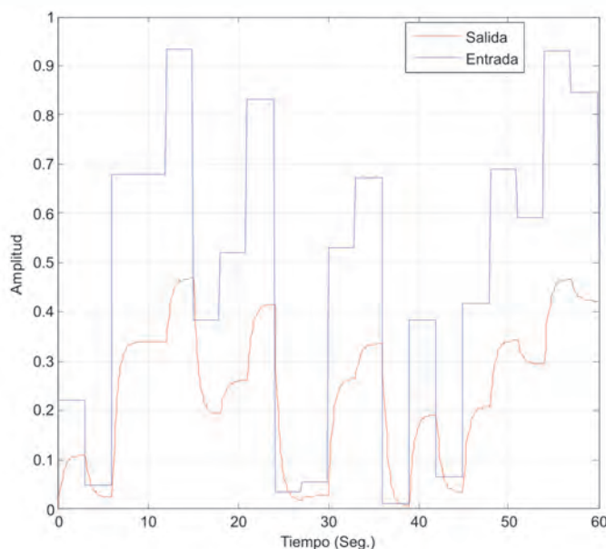
Fig. 6.20 Una posible entrada y su salida obtenida en la Simulación
