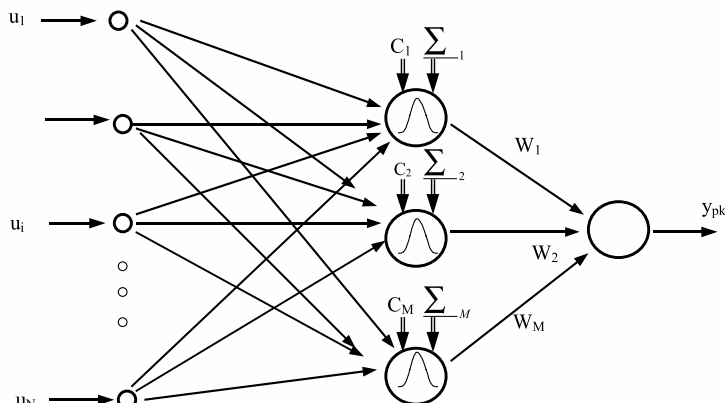
Fig. 6.7 Arquitectura de una red RBF
