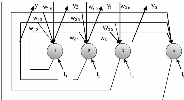
Fig. 4.3 Modelo discreto de Hopfield
