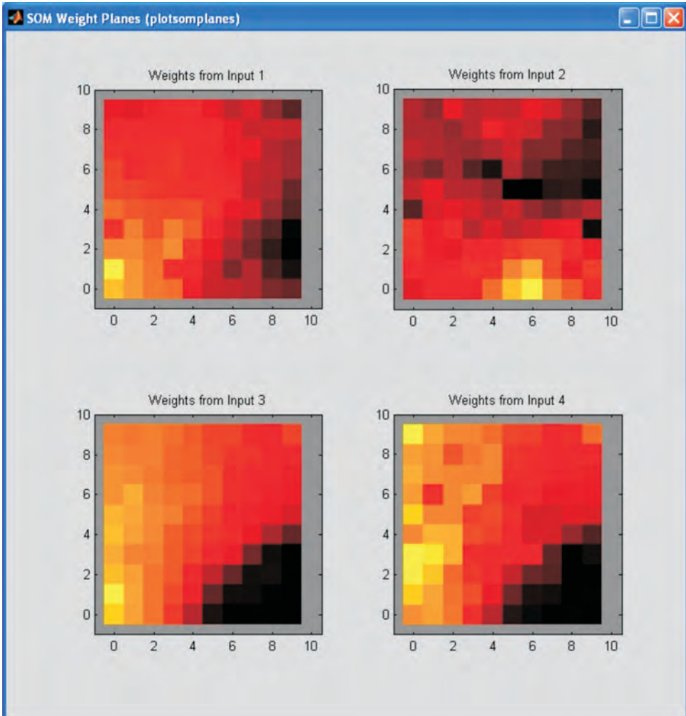
Fig. 5.24 Análisis de planos para las diferentes entradas de la red neuronal
