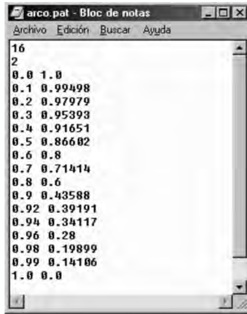
Fig. 5.16 Archivos de patrones.
