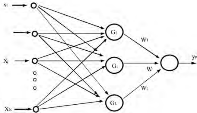
Fig. 6.3 Red de regularización
