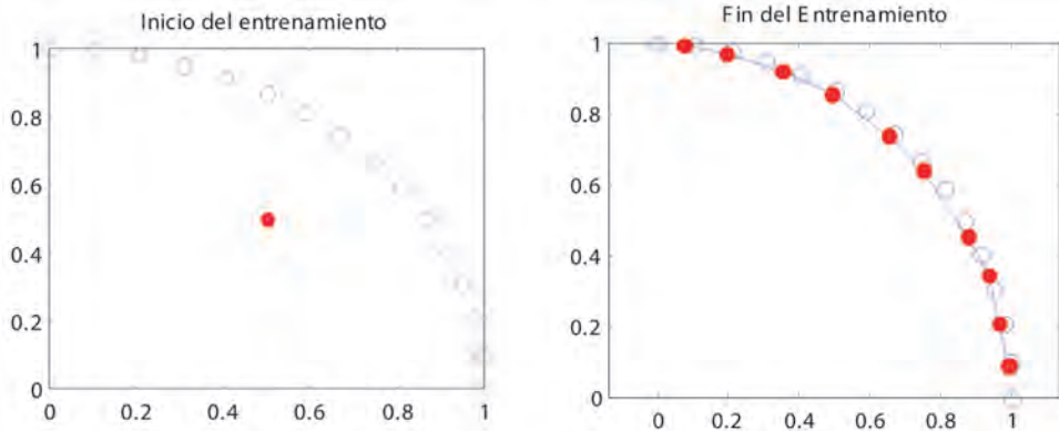
Fig. 5.13 Resultado del proceso de aprendizaje
