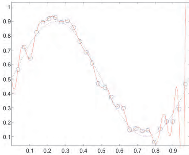
Fig. 6.14 Interpolación exacta realizada con una función de Gauss
