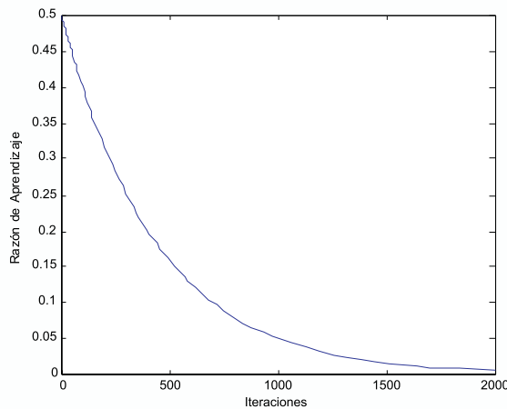
Fig. 5.5 Variación de la Razón de Aprendizaje \alpha(t)
