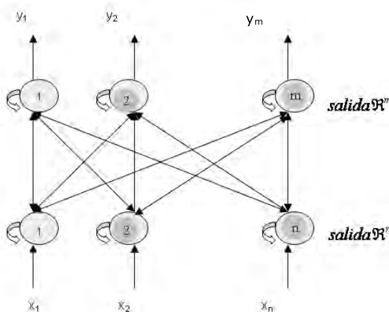
Figura 4.1 Memoria Asociativa Bidireccional
