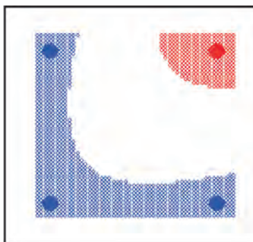
Fig. 6.10 Solución de la función AND con una red tipo MLP
