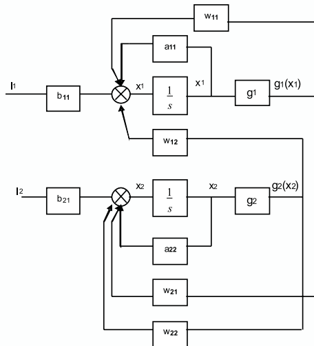
Fig. 4.6 Representación en Espacio de Estado del Modelo Continuo de Hopfield para una Red de dos Neuronas
