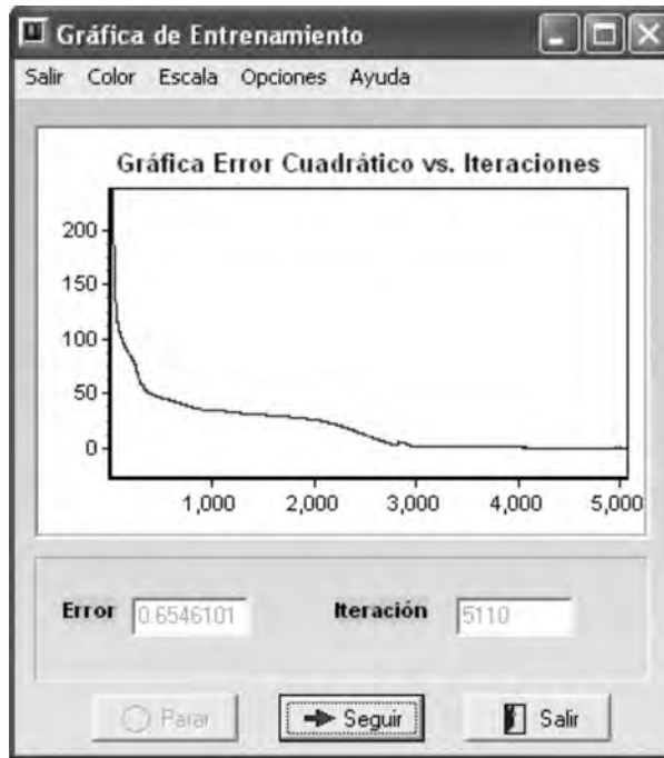
Fig. 3.30 Curva del error cuando \alpha = 0.005 \beta = 0.1
