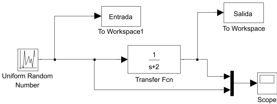
Fig. 6.19 Esquema en Simulink del experimento
