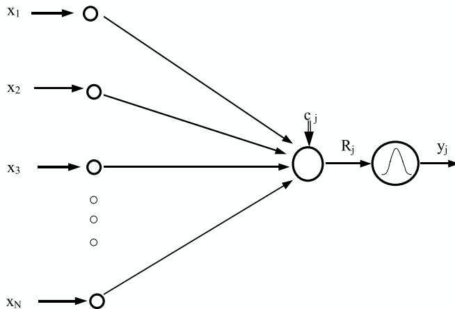
Fig. 6.6 Elemento de procesamiento de una RBF
