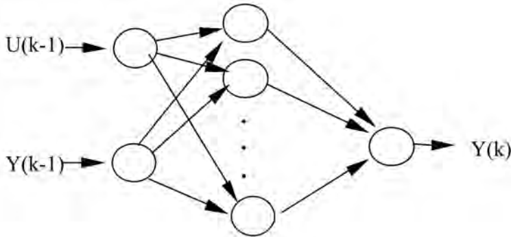
Fig. 6.21 Estructura de la red utilizada para la identificación
