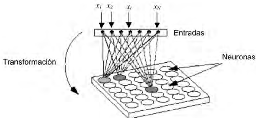
Figura 5.1 Mapa Auto Organizado
