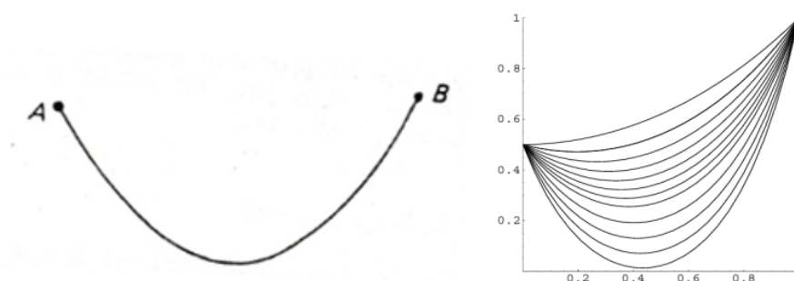
Figura 13. Forma catenaria
