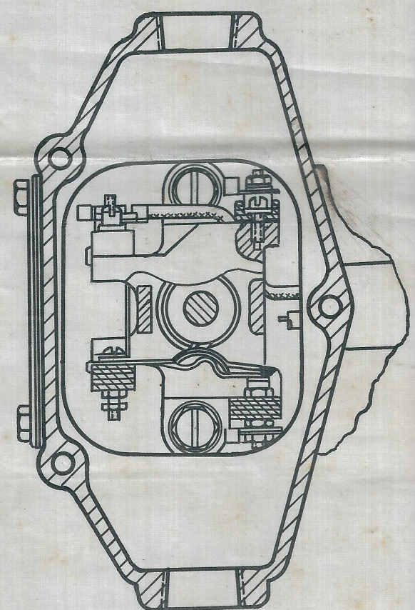
SECCION POR "A"
