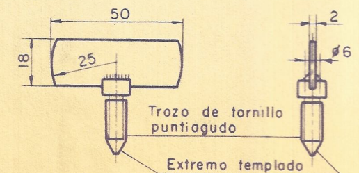
4- TORNILLO DE PRESION Tornillo y lámina de acero
