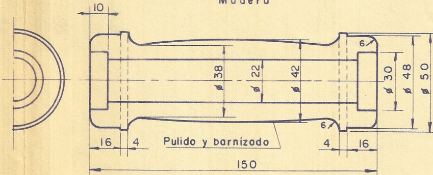
7- MONTAJE CENTRAL Madera
