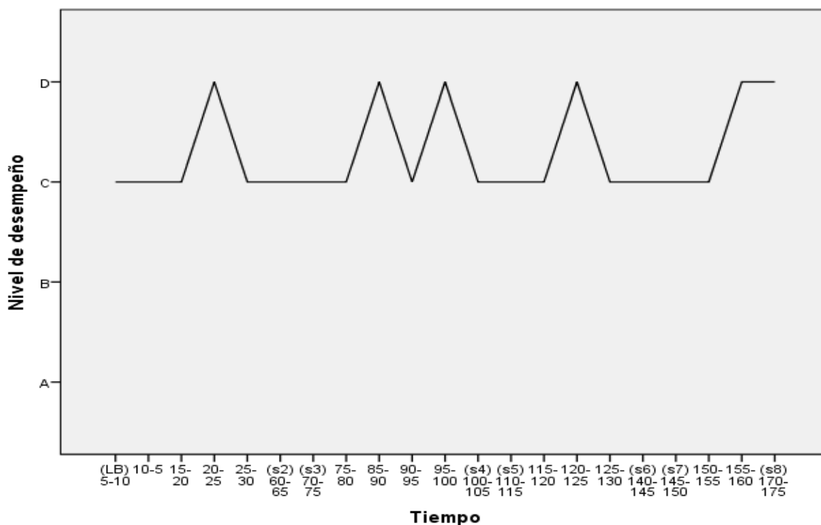
Gráfico 5.3.1. Trayectoria de desarrollo de la habilidad “Pensamiento covariativo” durante las sesiones
