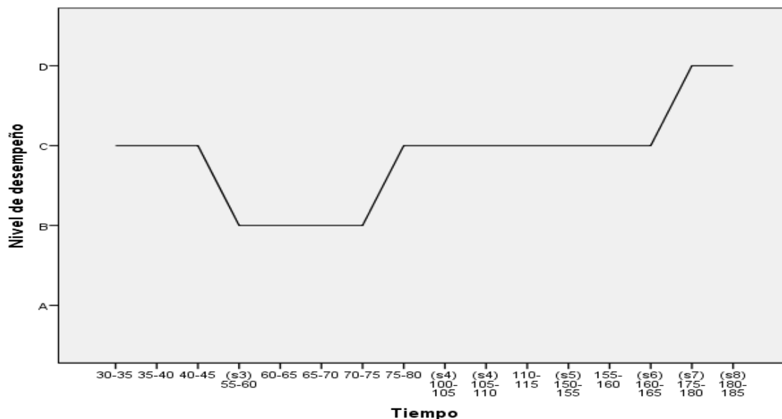
Gráfico 5.4.3. Trayectoria de desarrollo de la habilidad “Notación algebraica” durante las sesiones
