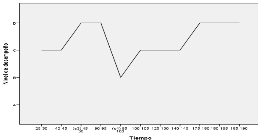
Gráfico 5.1.3. Trayectoria de desarrollo de la habilidad “Notación algebraica” durante las sesiones
