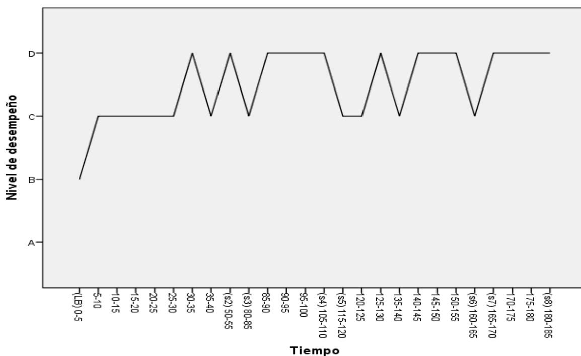
Gráfico 5.4.1. Trayectoria de desarrollo de la habilidad “Pensamiento covariativo” durante las sesiones
