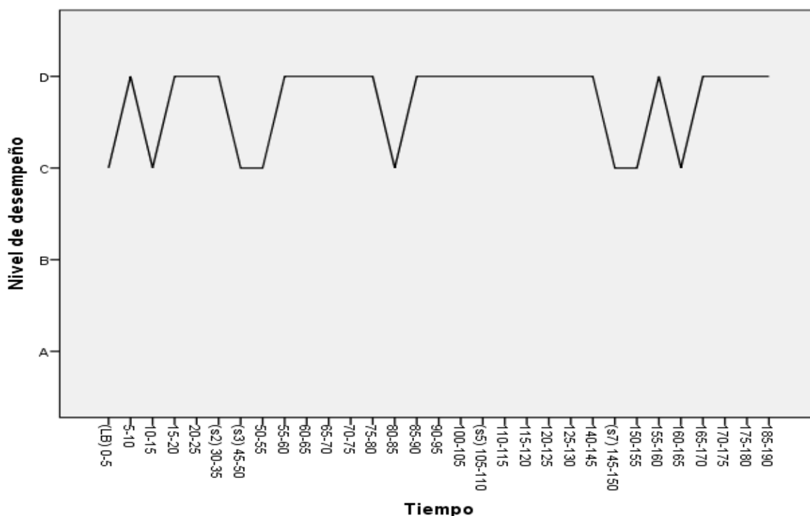
Gráfico 5.1.2 Trayectoria de desarrollo de la habilidad “Relaciones de correspondencia” durante las sesiones
