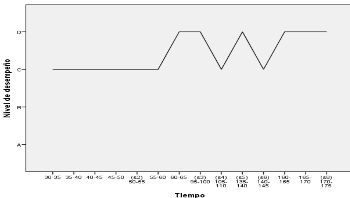
Gráfico 5.3.3. Trayectoria de desarrollo de la habilidad “Notación algebraica” durante las sesiones
