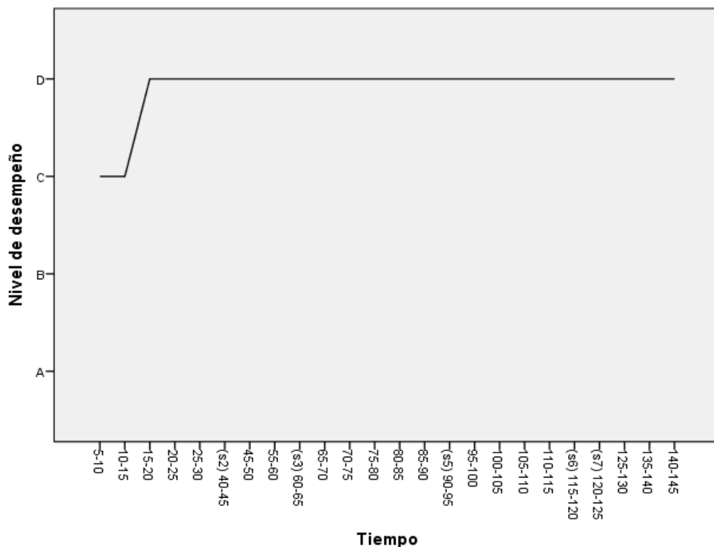
Gráfico 5.2.2. Trayectoria de desarrollo de la habilidad “Relaciones de correspondencia” durante las sesiones
