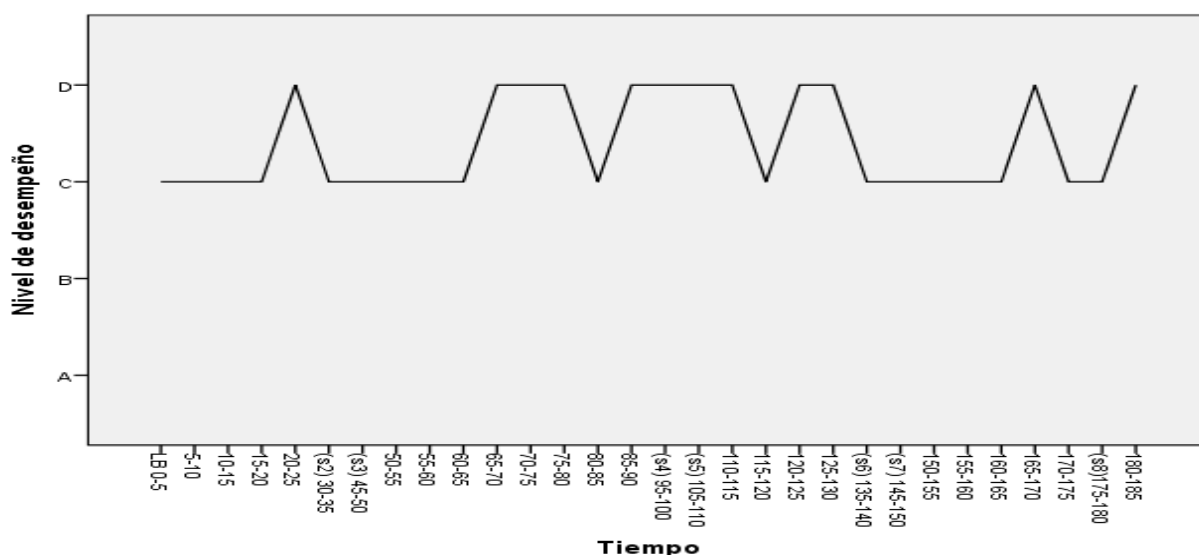
Gráfico 5.1.1 Trayectoria de desarrollo de la habilidad “Pensamiento covariativo”
