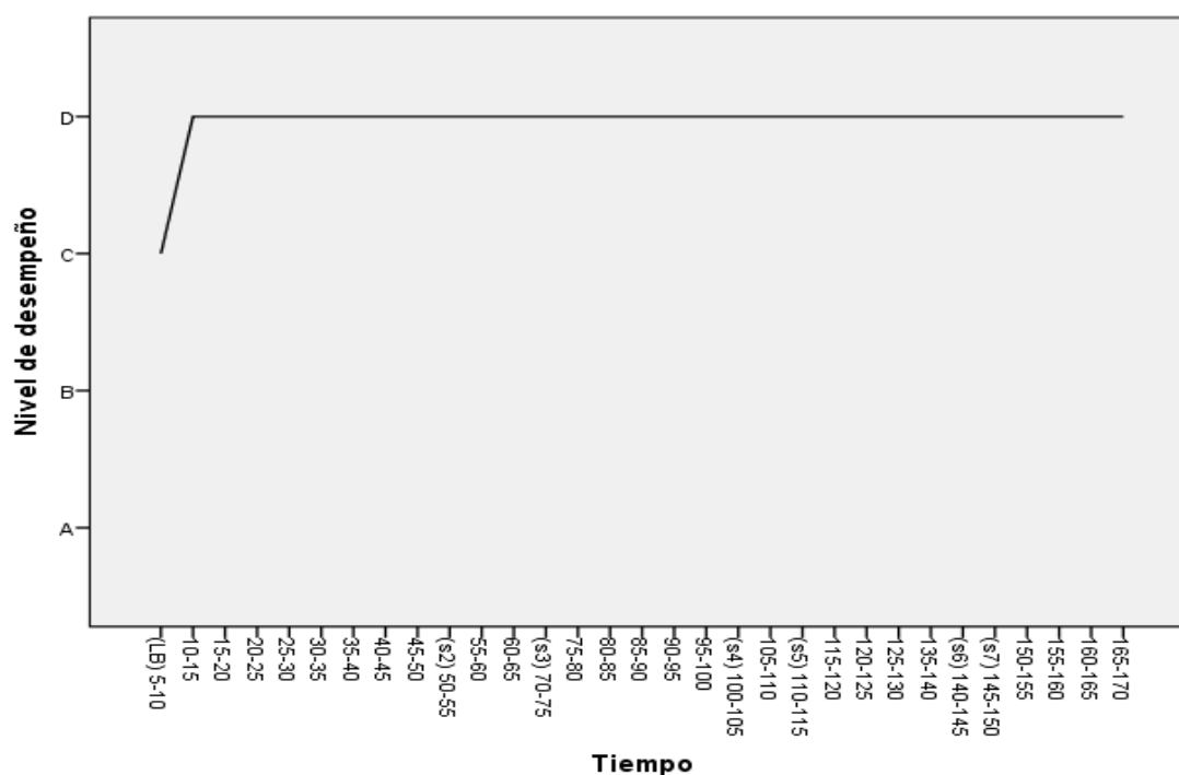
Gráfico 5.3.2. Trayectoria de desarrollo de la habilidad “Relaciones de correspondencia” durante las sesiones
