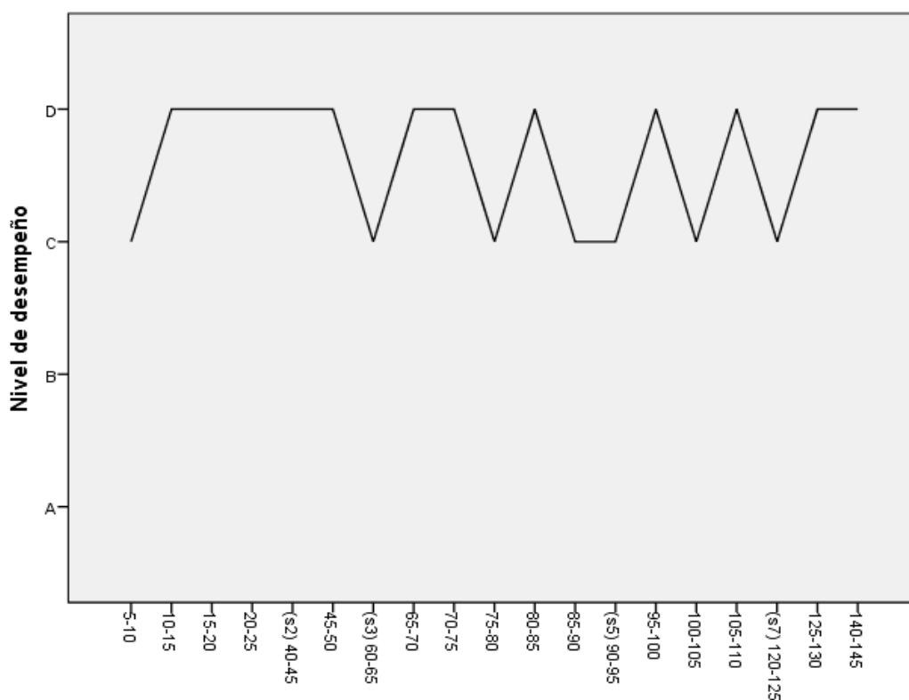
Gráfico 5.2.1. Trayectoria de desarrollo de la habilidad “Pensamiento covariativo” durante las sesiones
