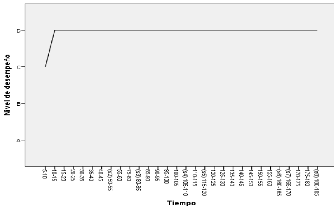
Gráfico 5.4.2. Trayectoria de desarrollo de la habilidad “Relaciones de correspondencia” durante las sesiones
