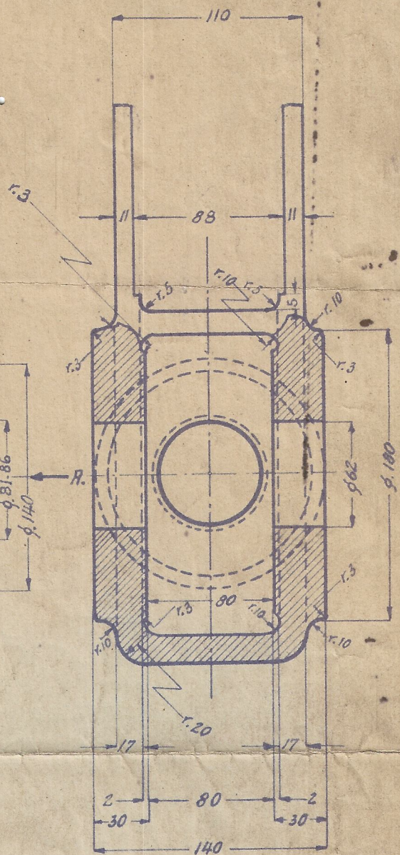
Seccion B.B.
