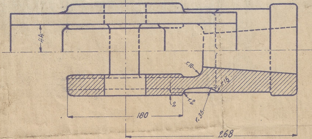
Seccion A.A.
