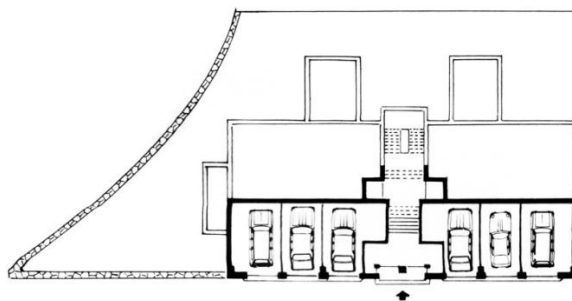
Figura 27. Plano de los parqueaderos de los apartamentos de sectores encumbrados o élite. En el edificio Carrera Quinta, construido en Bogotá en 1930 (Escala, 1983: 92).
