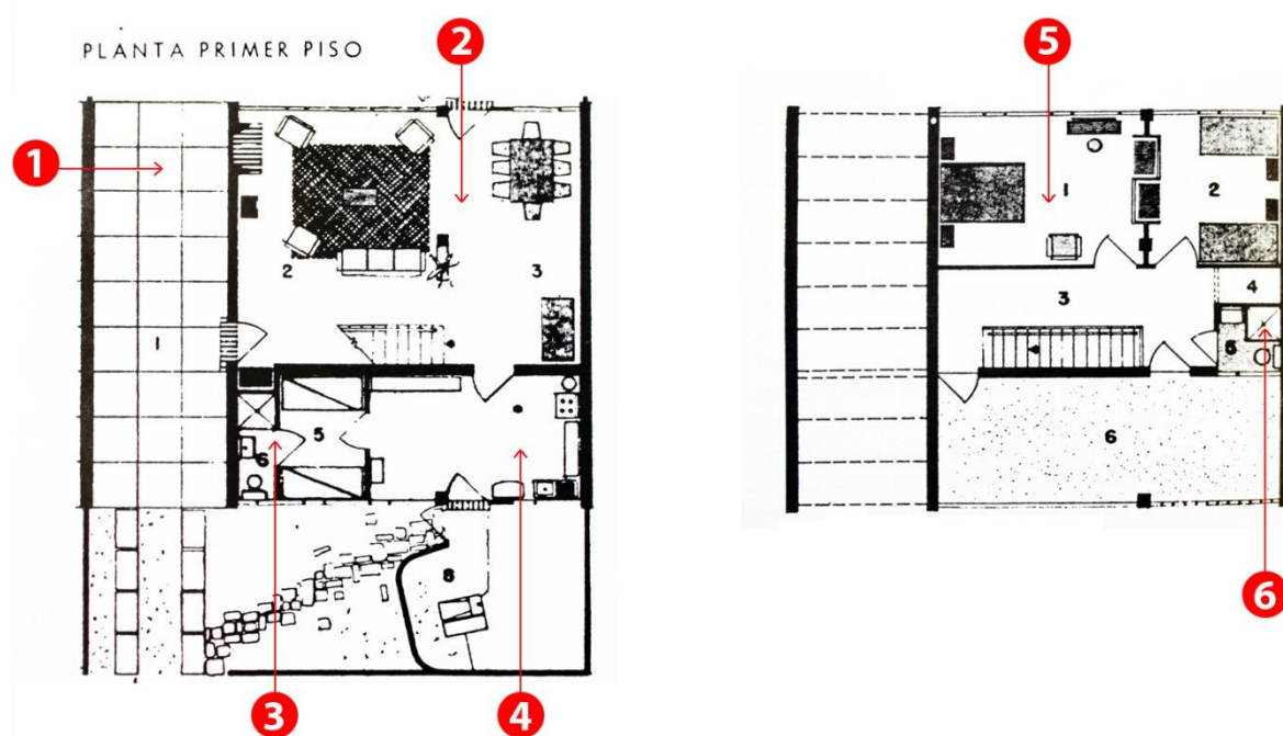
Figura 37. Plano de las viviendas construidas en el barrio Los Alcázares en Bogotá. 1949. Conformación espacial de un sector popular. Zona social: (1) garaje y zona de ampliación en el segundo piso, (2) sala-comedor. Zona de servicios: (3) baño social, (4) cocina. Zona privada: (5) alcoba, (6) baño de alcobas (Arango, 1989: 226).
