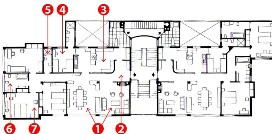
Figura 39. Plano de los apartamentos Avenida Caracas construidos en Bogotá. 1949. Conformación espacial de sectores entre acomodados y élite. Zona social: (1) sala-comedor y (2) hall de distribución. Zona de servicios: (3) cocina y (4) alcoba del servicio. Zona privada: (5) baño de alcobas y social, (6) baño de alcobas y (7) alcoba. (Escala, 1983: 88).
