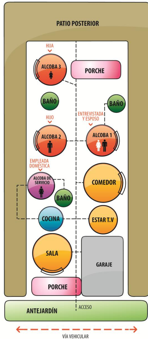
ESQUEMA No. 6.4 Casa urbana en la ciudad de Barranquilla, Atlántico (1970 - 1975)
