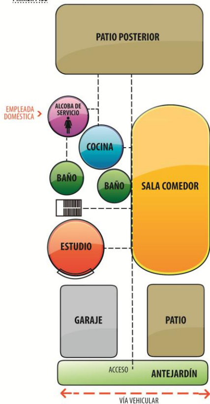
ESQUEMA No. 8.7 Casa urbana en el barrio Los Chorros de Cali (1974 - 1976)
