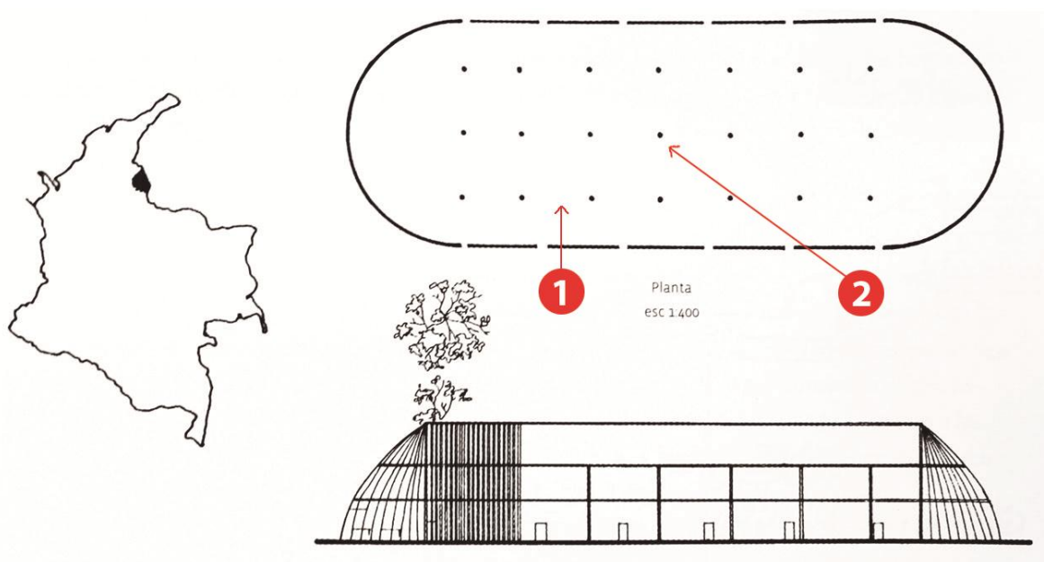
Figura 9. Bohío Barí Motilón, Catatumbo. (1) zona de hornos y (2) área para colgar hamacas (Saldarriaga, 2009: 56).
