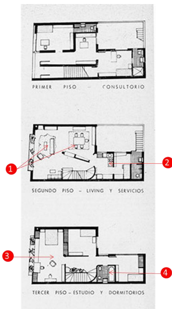
Figura 26. Plano de la vivienda de sectores acomodados de la casa Gabriel Serrano construida en Bogotá.1939. (1) zona social: sala-comedor unidos, (2) zona de servicios: cocina y ropas, (3) zona privada: alcobas y (4) baño para alcobas (Arango, 1989: 198).
