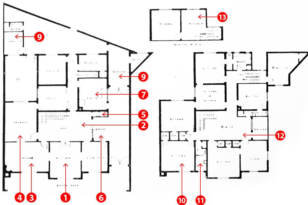
Figura 25. Plano de una vivienda de sectores encumbrados o élite en Bogotá. 1942. Primer piso. Zona social: (1) vestíbulo o recibo, (2) hall de repartición de área social, (3) sala, (4) comedor, (5) baño social, (6) porche o estar exterior y (9) garaje. Zona de servicio: (7) cocina y (8) alcoba de servicio. Segundo piso. Zona privada: (10) alcobas, (11) baño de las alcobas y (12) hall de repartición de área privada. Tercer piso: (13) estudio (Arango, 1989: 178).
