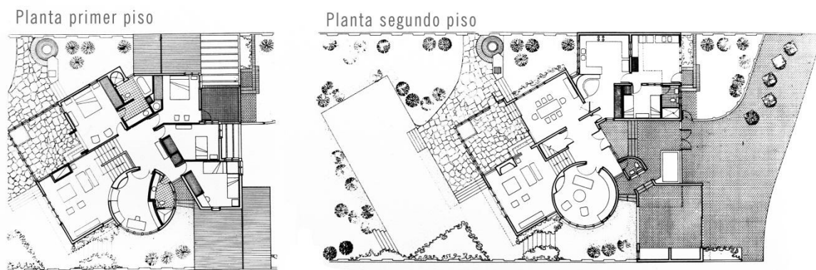
Figura 41. Plano de la casa para el arquitecto Ignacio Gómez Carrasco. Bogotá. 1970. (Sociedad Colombiana de Arquitectos, 1970: 96).
