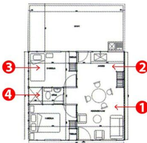
Figura 50. Plano de las viviendas de interés social construidas en Cauca, Antioquia. 2012. (Escallón, 2012: 264).
