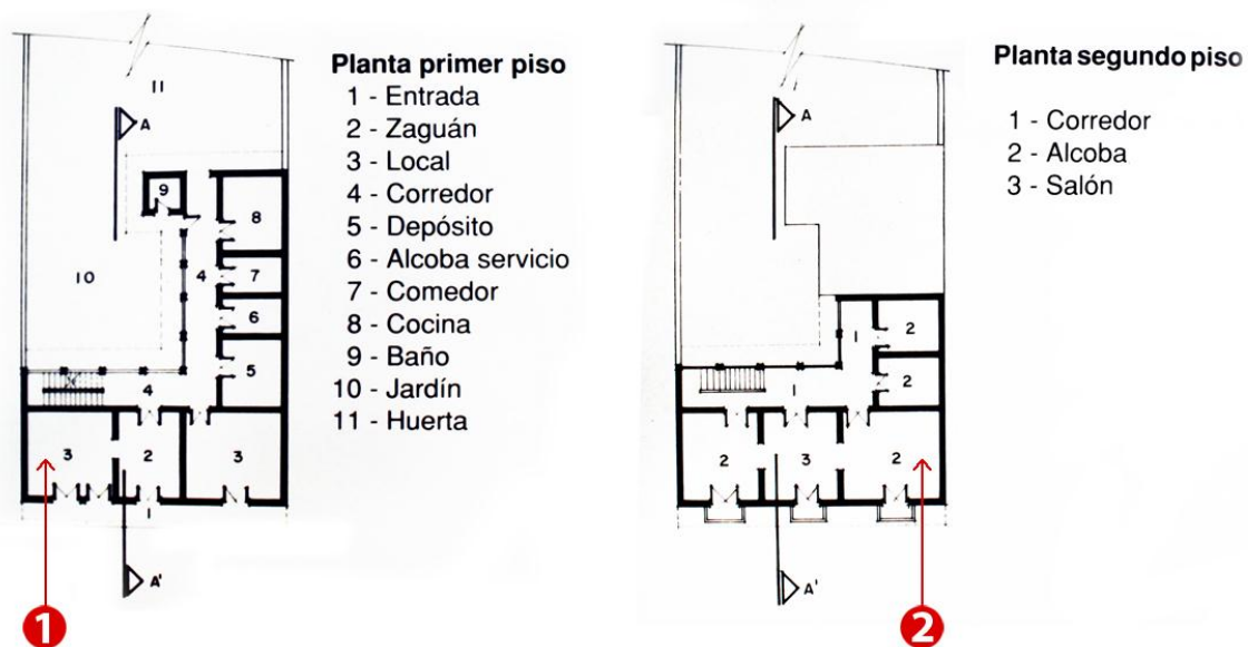
Figura 21. Plano de una casa construida en Murillo, Tolima. 1871. Localizada cerca a la plaza de Bolívar. (1) zona de vivienda y (2) zona de depósito (Tobón, 1989: 50).
