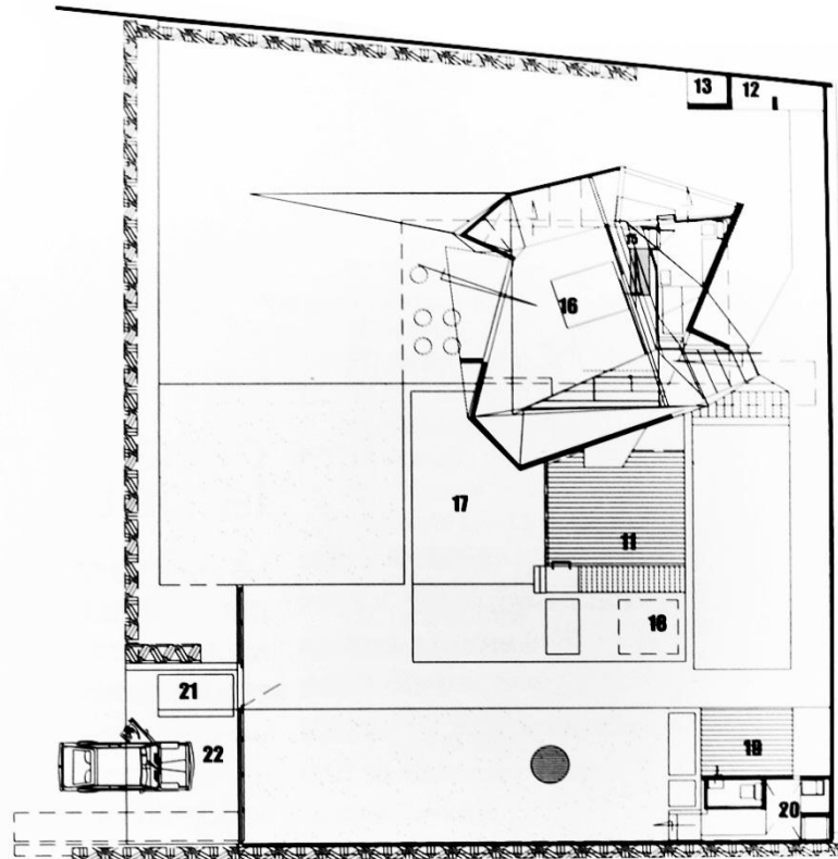
Figura 47. Plano de la casa Samanes Villa del Rosario. Norte de Santander. 2010 (Sociedad Colombiana de Arquitectos, 2010: 132).
