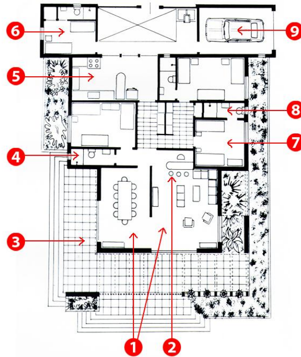
Figura 29. Plano de la Quinta Jaramillo Arango, Fusagasuga, 1935. (1) sala-comedor, (2) bar, (3) terraza-corredor, (4) baño social, (5) cocina, (6) alcoba de servicio, (7) alcoba, (8) baño privado y (9) garaje (Escala, 1983: 38).
