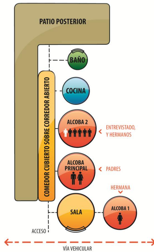
ESQUEMA No. 7.7 Casa urbana en la ciudad de Pereira, Risaralda (1955 - 1959)
