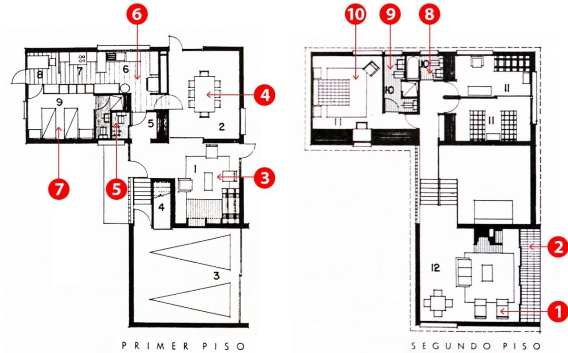
Figura 35. Plano de la casa de Francisco Pizano construida en Bogotá. 1950. Conformación espacial de sectores entre acomodados y élite. Zonificación agrupada. Zona social: (1) sala, (2) balcón, (3) estar, (4) comedor, (5) baño social. Zona de servicios: (6) cocina, (7) alcoba de servicio. Zona privada: (8) baño de alcobas, (9) baño privado y (10) alcoba principal (Arango, 1989: 222).
