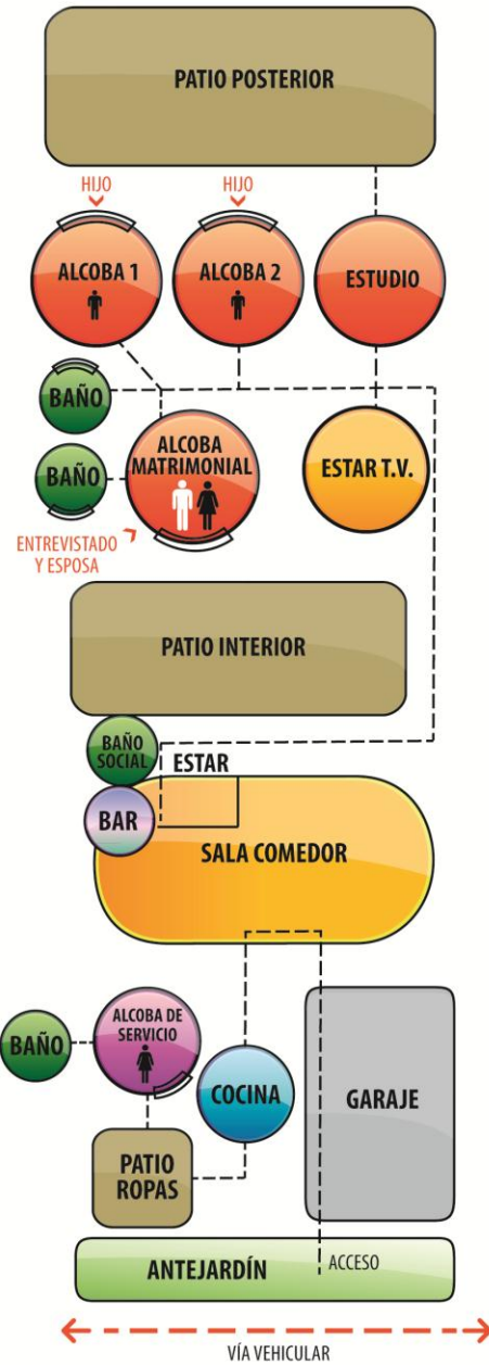
ESQUEMA No. 9.5 Casa urbana en el barrio Cuarto de Legua de Cali (1977 - 2004)
