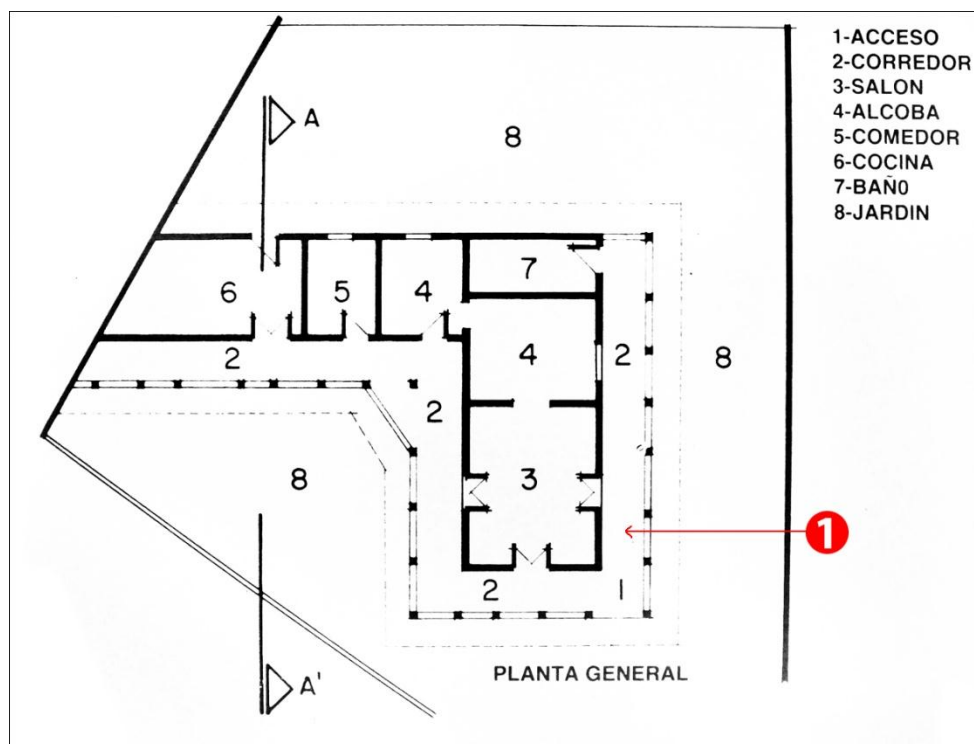
Figura 22. Plano de una casa construida en Villa Quindío, Montenegro. 1910. (1) corredor (Tobón, 1989: 122).
