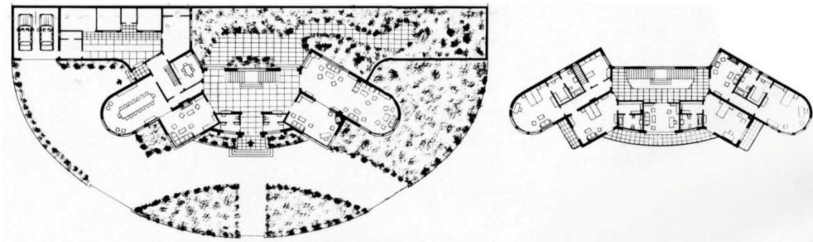
Figura 44. Plano de la casa Olaya Herrera. Bogotá. 1931. (Escala, 1983: 35).
