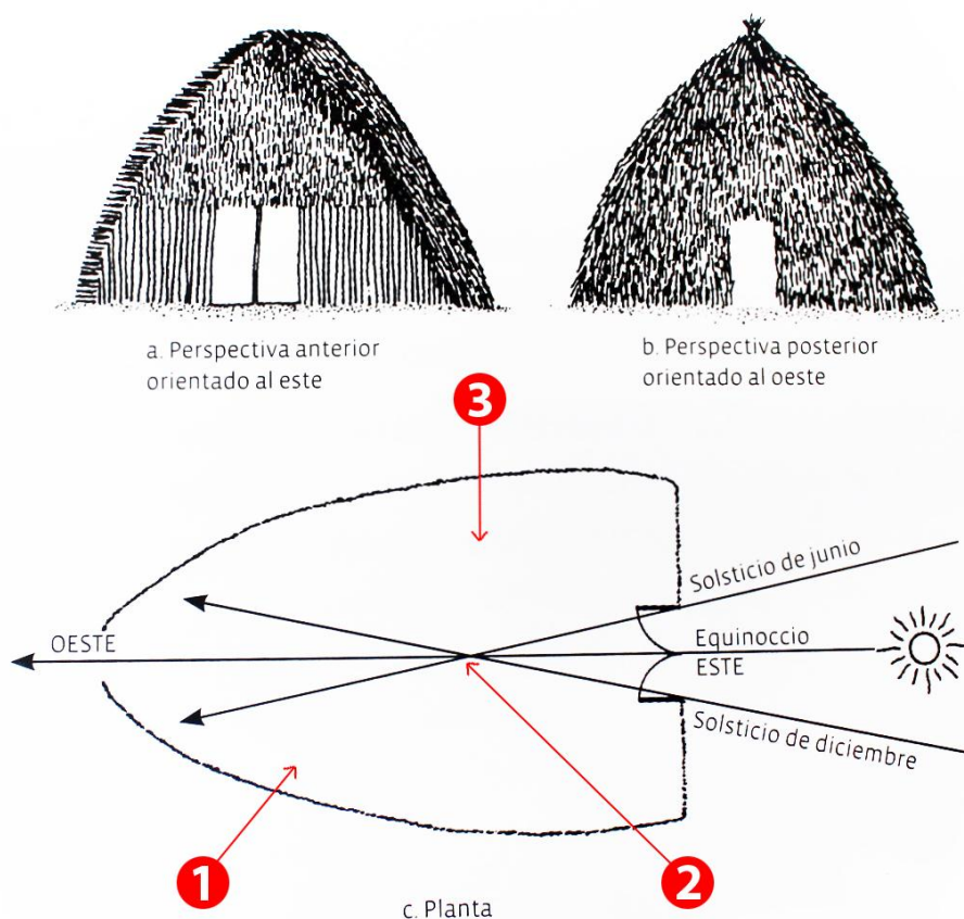
Figura 12. Plano de una vivienda Uwá. 1995. (1) fogón de los alimentos, (2) dormitorio y (3) fogón donde se tuestan hojas (Saldarriaga, 2009: 48).
