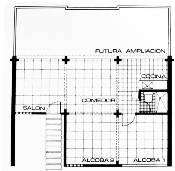
Figura 46. Plano del (conjunto) plan 400 s.m. Cartagena. 1972. Vivienda para personas de bajos ingresos (Sociedad Colombiana de Arquitectos, 1971: 17).
