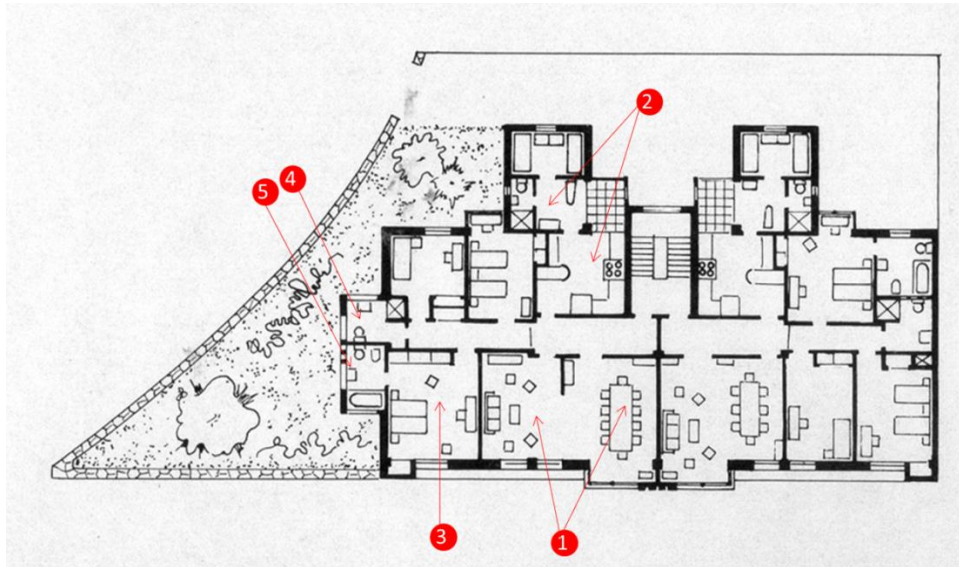
Figura 28. Plano de los apartamentos de sectores encumbrados o élite. En el edificio Carrera Quinta, construido en Bogotá en 1930. (1) zona social: sala-comedor, (2) zona de servicios: cocina, ropas y alcoba de servicio, (3) zona privada: alcobas, (4) baño de las alcobas y (5) baño privado de la alcoba (Escala, 1983: 92).
