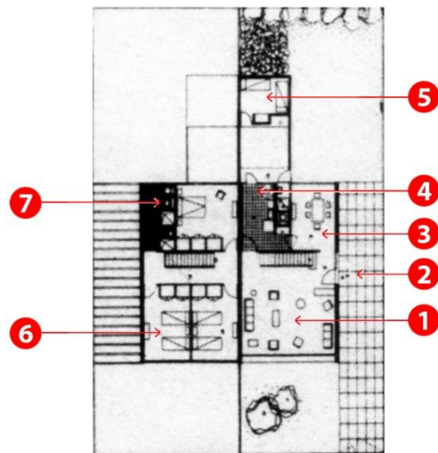
Figura 36. Plano de las viviendas construidas para el barrio El Polo en Bogotá. 1957. Conformación espacial de un sector acomodado. Zona social: (1) sala, (2) garaje y (3) comedor. Zona de servicios: (4) cocina y (5) alcoba del servicio. Zona privada: (6) alcoba y (7) baño de alcobas (universidad de los Andes, 2004: 81).
