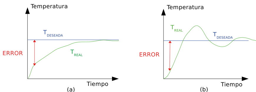
Figura 7. Evolución en el tiempo de una realimentación negativa (a) subamortiguada y (b) sobreamortiguada
