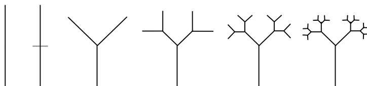
Figura 25. Fractal arbóreo (híbrido)
