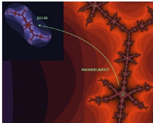
Figura 47. Localmente, Julia y Mandelbrot se parecen
