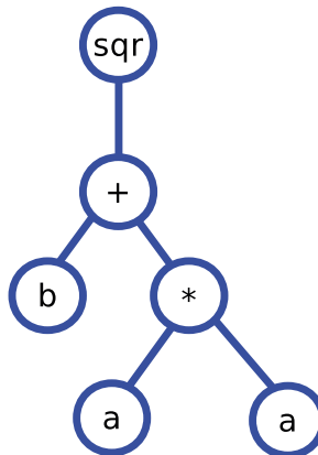
Figura 165. Árbol sintáctico
