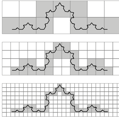
Figura 33. Cálculo de la dimensión dMB del fractal de Koch por conteo de cajas
