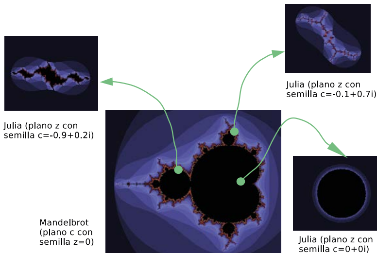
Figura 44. Mandelbrot como catálogo de Julias
