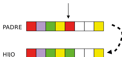
Figura 113. Mutación
