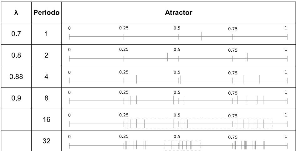
Figura 76. Duplicación de periodo en la curva logística
