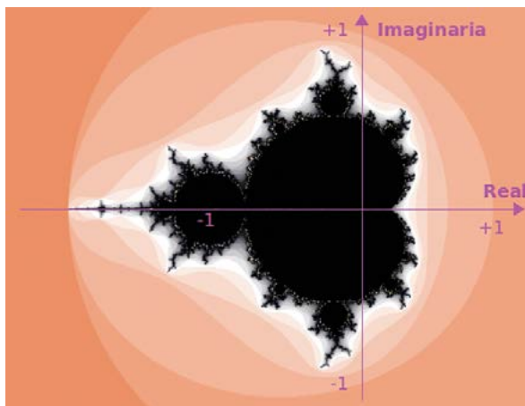
Figura 42. Fractal de Mandelbrot
