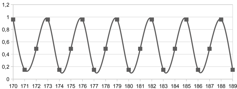
Figura 78. Curva logística con periodo 3 para \lambda=0.96
