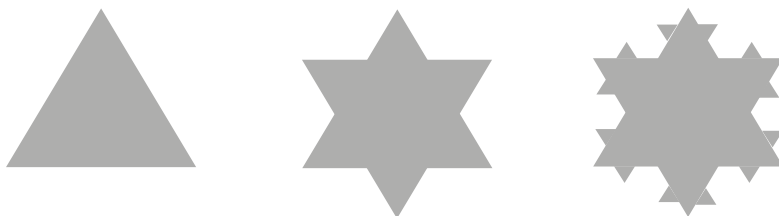
Figura 27. Fractal copo de nieve
