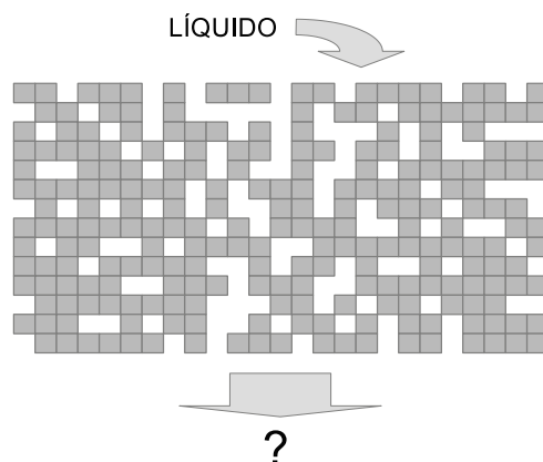
Figura 52. Retícula como modelo para estudiar la percolación
