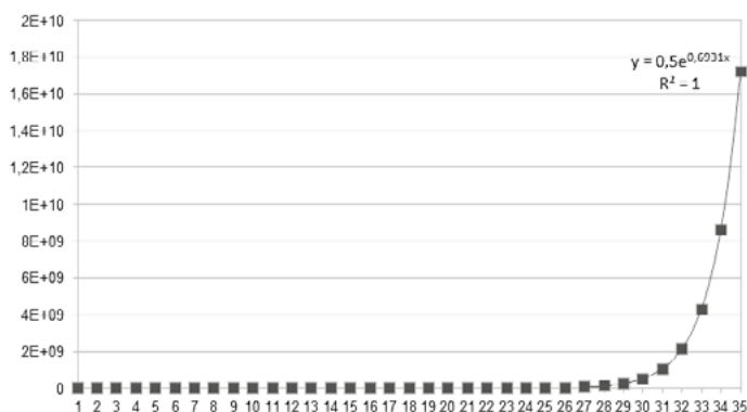
Figura 17. Reproducción exponencial
