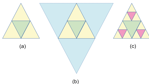
Figura 51. Demostración geométrica
