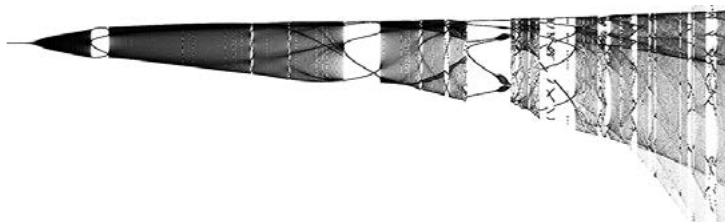
Figura 86. Diagrama de bifurcaciones de Tinkerbell
