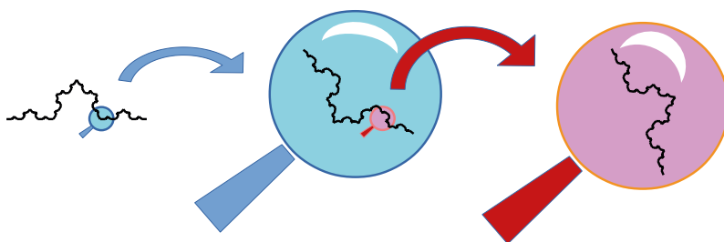
Figura 35. Invariancia frente a cambios de escala
