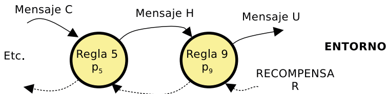
Figura 140. Reparto de recompensas con algoritmo brigada de baldes
