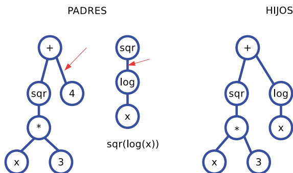
Figura 157. Cruce. Las flechas indican los puntos de corte elegidos al azar
