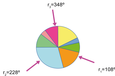
Figura 112. Ejemplo de selección de 3 cromosomas por ruleta
