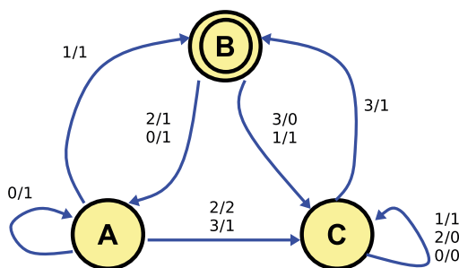
Figura 141. Máquina de estados finitos
