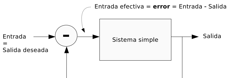
Figura 5. Realimentación negativa
