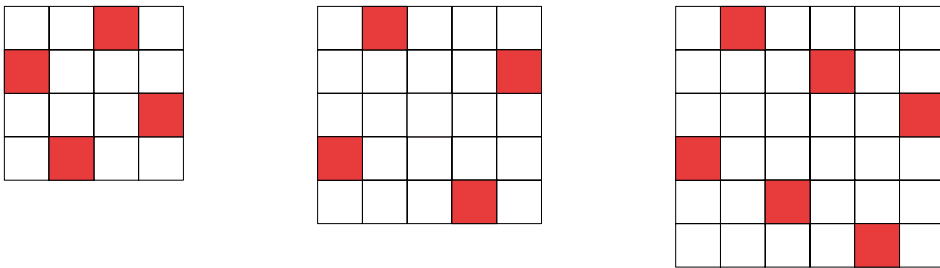
Figura 117. Solución a las N -Damas para N=\{4, 5, 6\}
