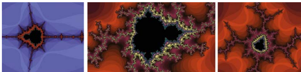
Figura 43. En los interiores de Mandelbrot
