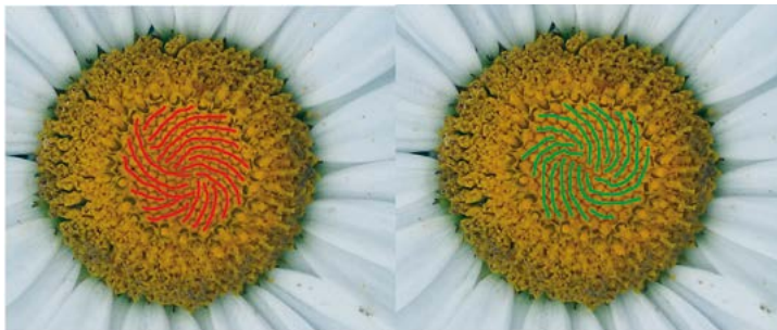
Figura 20. Margarita con 18 espirales dextrógiros (en rojo) y 16 levógiros (en verde)
