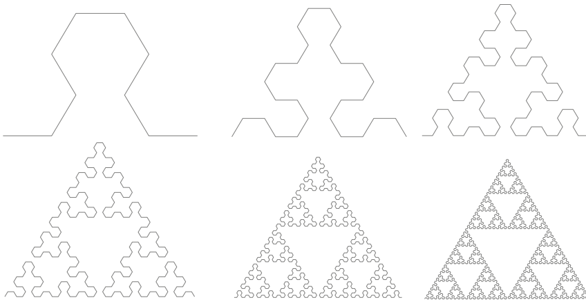
Figura 38. Sucesivas aproximaciones al triángulo de Sierpinski, usando una gramática de Lindenmayer
