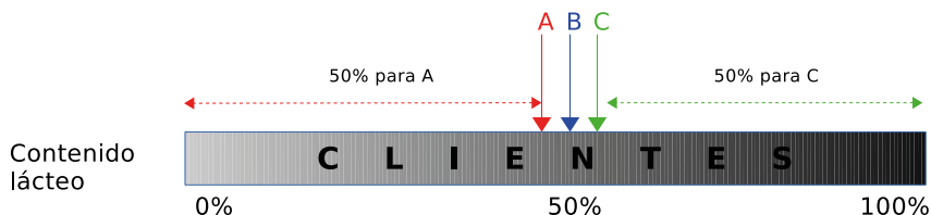
Figura 174. Aparece una tercera empresa
