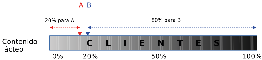
Figura 172. Dos marcas de helados
