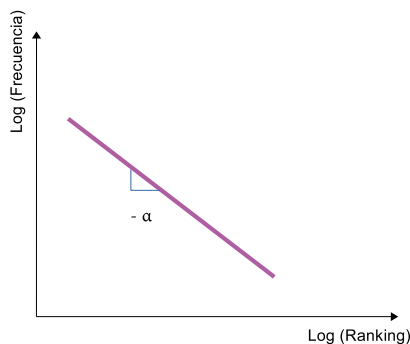
Figura 99. Distribución de Zipf (univariada)
