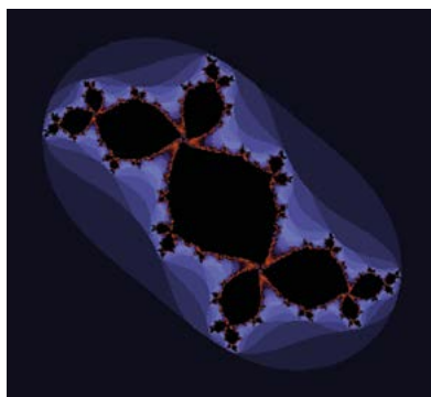
Figura 45. Conejito de Douady
