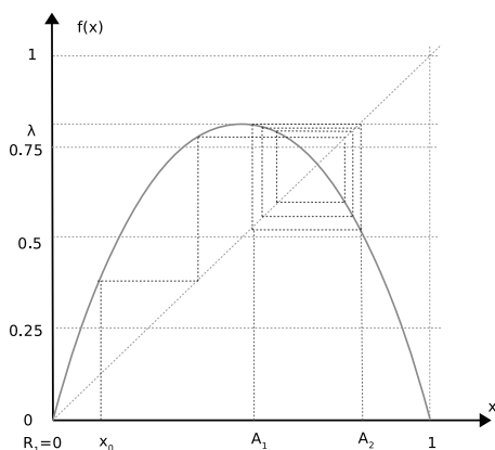
Figura 68. Curva logística para x_0=0.2 y \lambda=0.8
