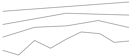
Figura 49. Fractal por desplazamiento del punto medio (se muestran 4 iteraciones, en sentido hacia abajo)
