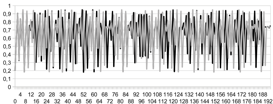
Figura 73. Curva logística en caos, con \lambda=0.95 para x_0=0.2 (en negro) y x_0=0.2001 (en gris)
