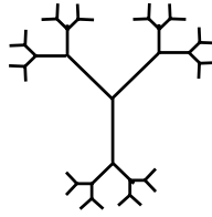
Figura 32. Fractal arbóreo
