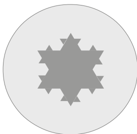
Figura 34. El área del fractal copo de nieve está acotada
