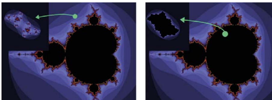
Figura 46. Julia inconexo y Julia conexo
