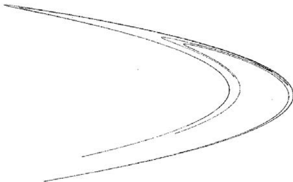
Figura 83. Uno de los atractores de Hénon para a=1.4 , b=0.3
