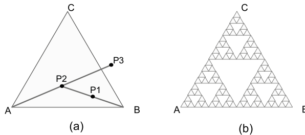
Figura 50. (a) Juego del caos; (b) estrategia ganadora
