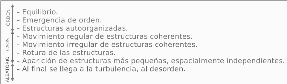
Figura 57. Transiciones del orden a la aleatoriedad pasando por el caos
