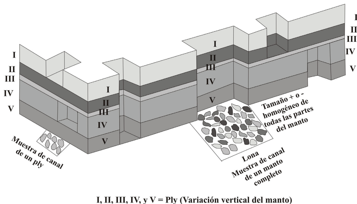
Figura 1. Esquema de muestreo de canal en un manto de carbón. Por cada 20 a 30 cm de espesor del manto, se toman de 2 a 3 kg de muestra.
