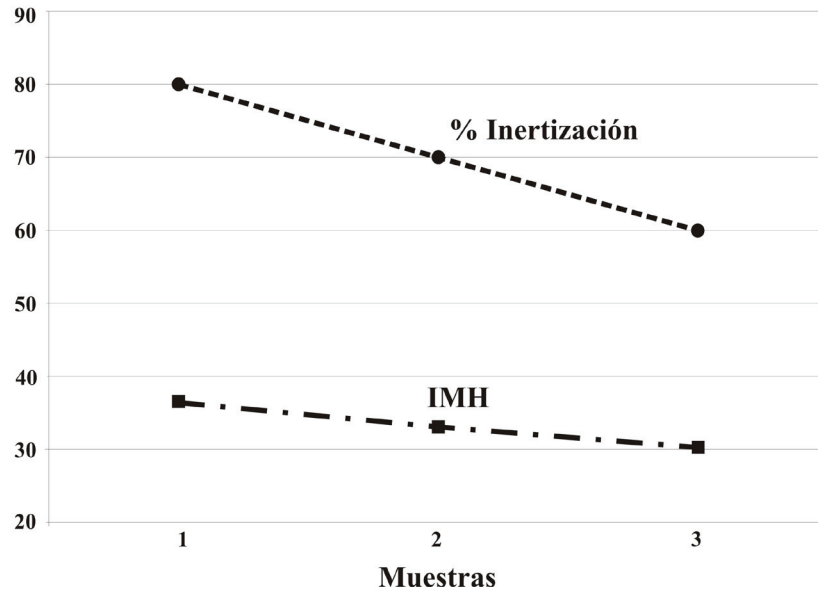
Figura 4. Relación del índice de molienda hardgrove con el porcentaje de inertización del polvo de carbón de un Manto de una Mina en Amagá.
