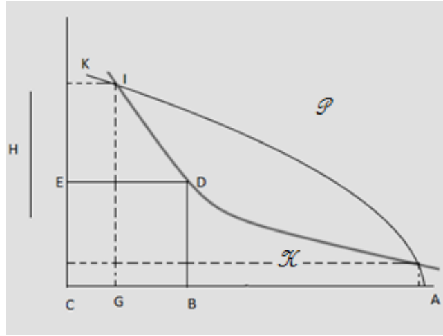
Figura 16. Representación de la intersección de la hipérbola y la parábola según al-Khayyām.
