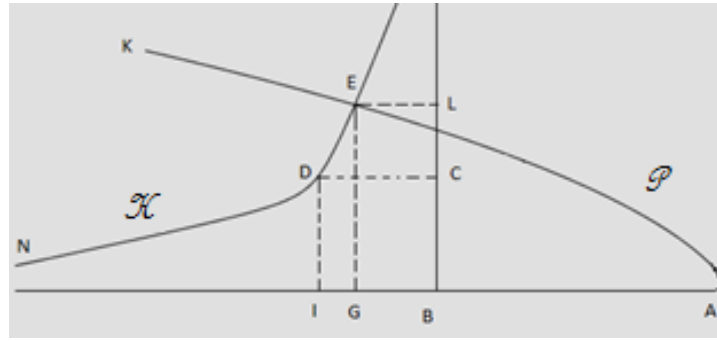
Figura 13. Representación de la intersección de la hipérbola y la parábola según al-Khayyām.
