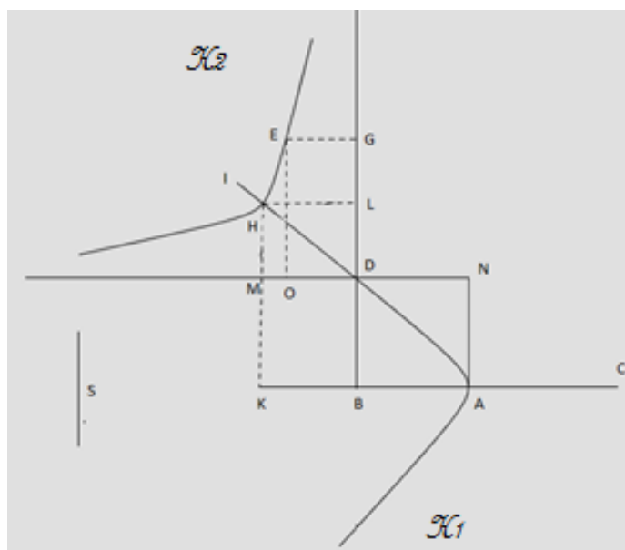
Figura 22. Representación de la intersección de las dos hipérbolas según al-Khayyām.
