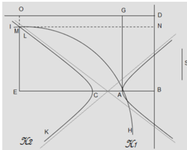
Figura 26. Representación de la intersección de las dos hipérbolas según al-Khayyām.
