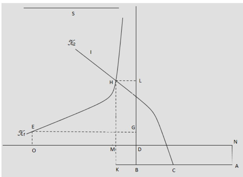
Figura 23. Representación de la intersección de las dos hipérbolas según al-Khayyām.
