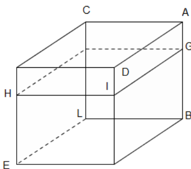
Figura 4. Representación del sólido en la ecuación 10 según al-Khayyām.
