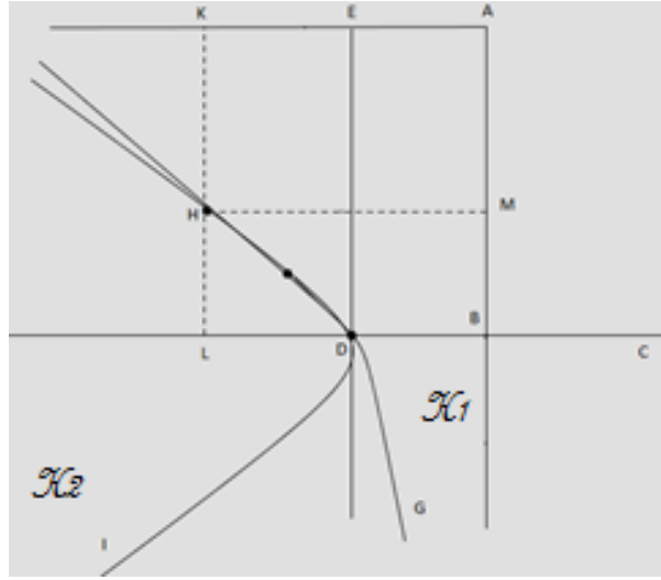
Figura 19. Representación de la intersección de las dos hipérbolas según al-Khayyām.
