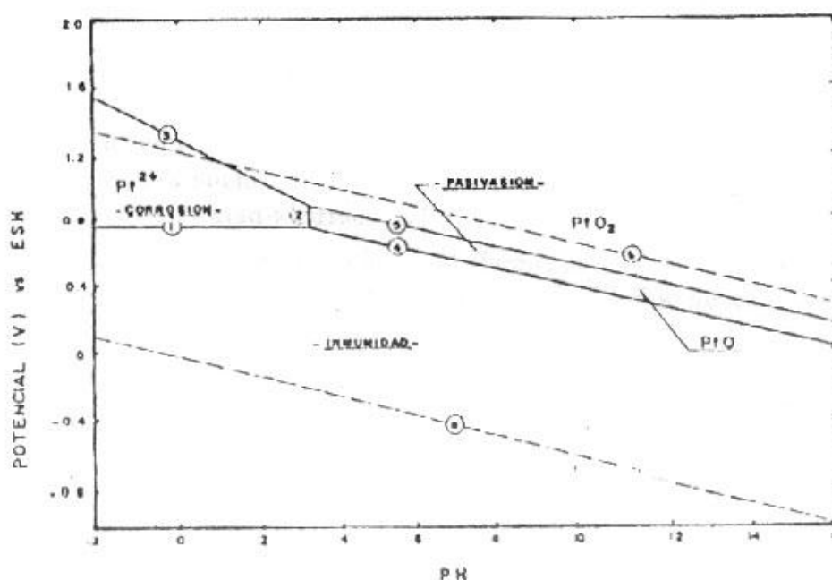
Figura 2. Diagrama de equilibrio potencial- pH para el sistema platino-agua a 25^{\circ}C
