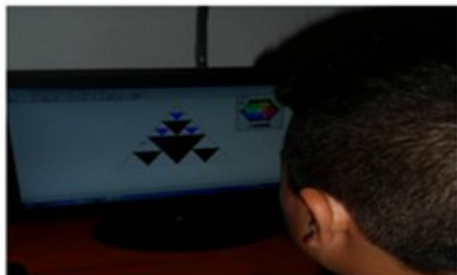
Ilustración 55: Construcción de fractal construido por etapas utilizando Cabri Geometry II Plus en el aula de sistemas según guía de la situación 4 Secuencia Aplicada.
