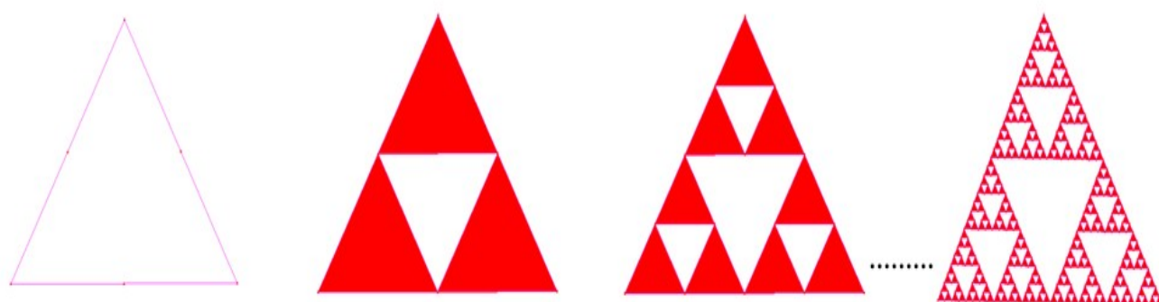
Ilustración 29: Construcción del Tapete Triangular.
