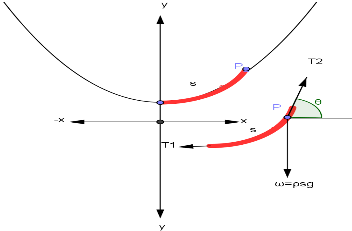
Ilustración 28: Diagrama de fuerzas en la catenaria
