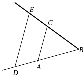
Ilustración 11: Producto de segmentos
