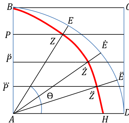
Ilustración 4: Trisección del ángulo con la trisectriz.
