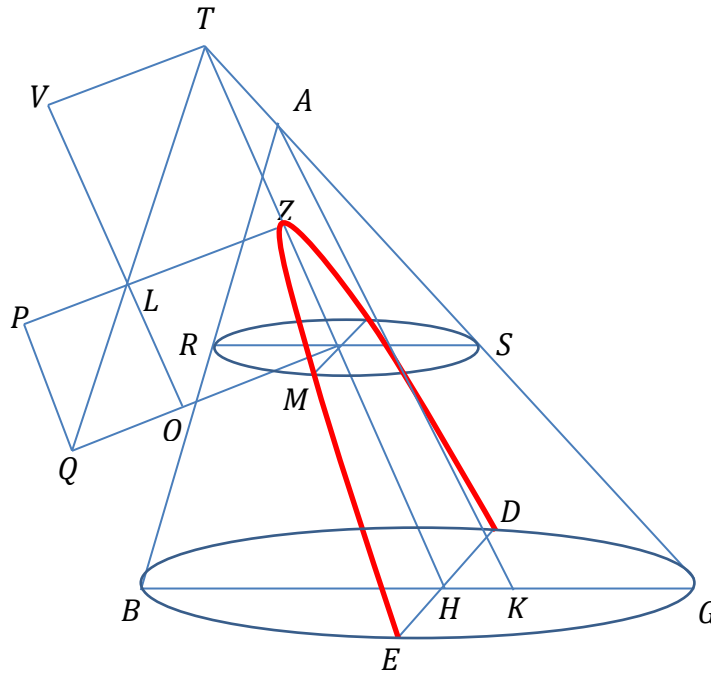
Ilustración 10: Síntoma de la hipérbola
