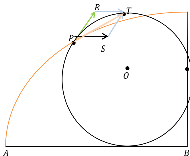
Ilustración 32: Tangente a la cicloide
