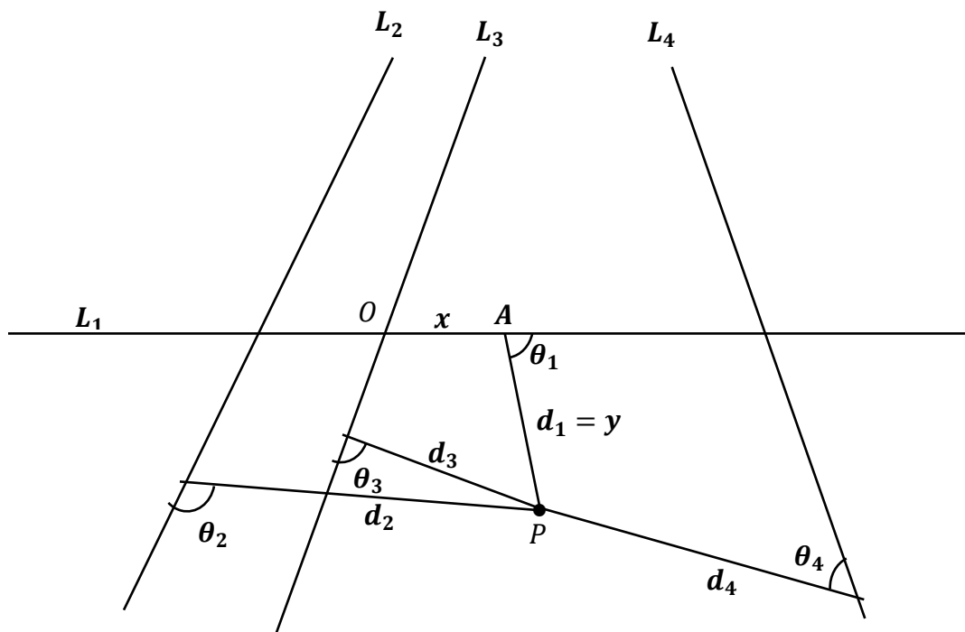
Ilustración 13: Generalización del problema de Pappus
