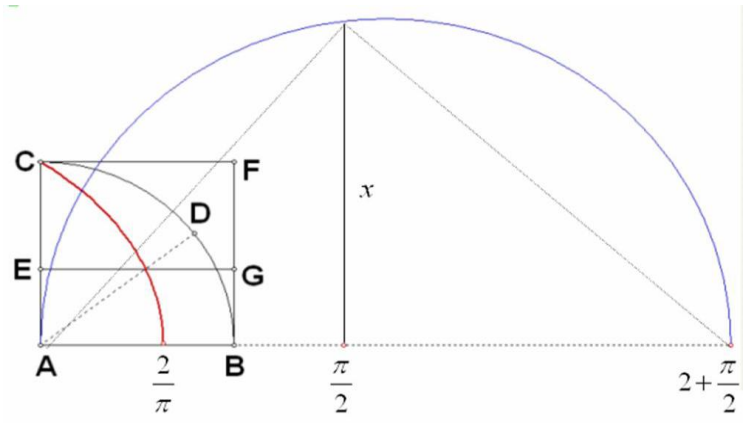
Ilustración 20: Cuadratura del círculo
