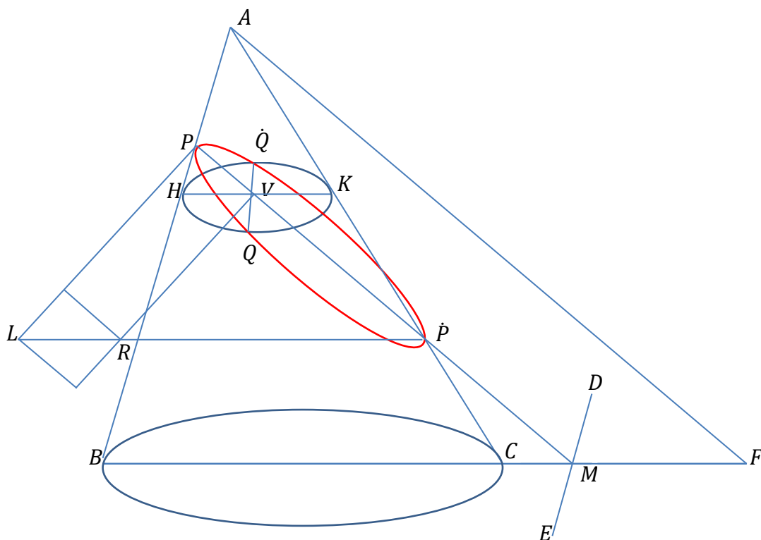
Ilustración 9: Síntoma para la elipse
