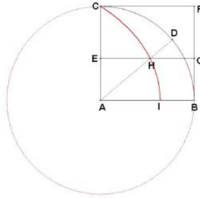
Ilustración 18: Cuadratura del círculo
