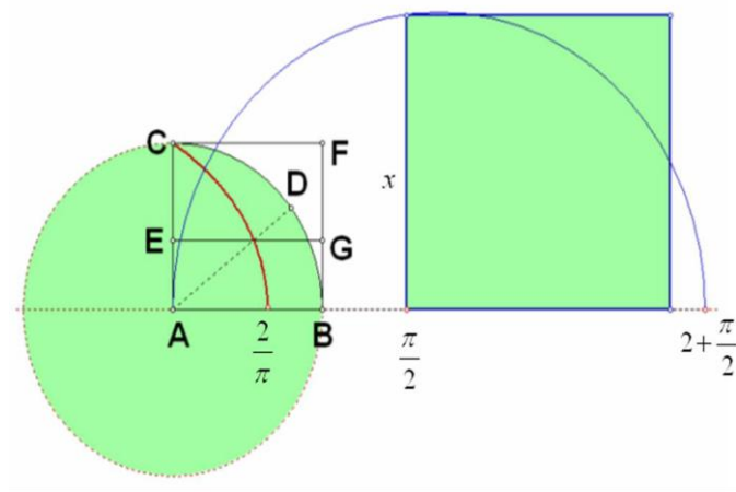
Ilustración 21: Cuadratura del círculo
