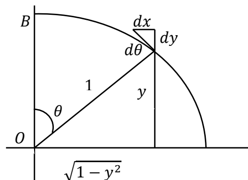
Ilustración 16: Desarrollo del seno
