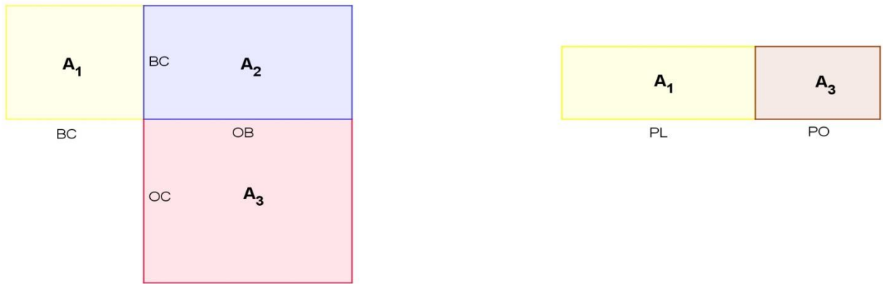
Ilustración 8: Rectángulos de igual altura
