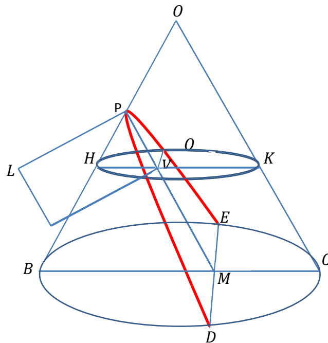
Ilustración 7: Obtención del síntoma de la parábola
