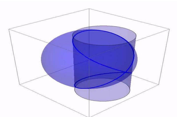
Ilustración 5: hipopede de Eudoxo
