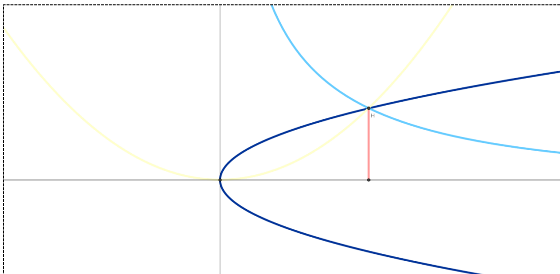
Ilustración 23: Duplicación del cubo
