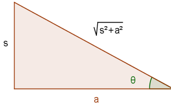
Ilustración 29: Triángulo para la sustitución trigonométrica
