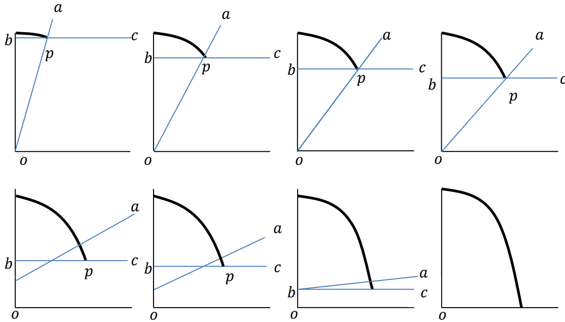
Ilustración 3: trisectriz o Cuadratriz
