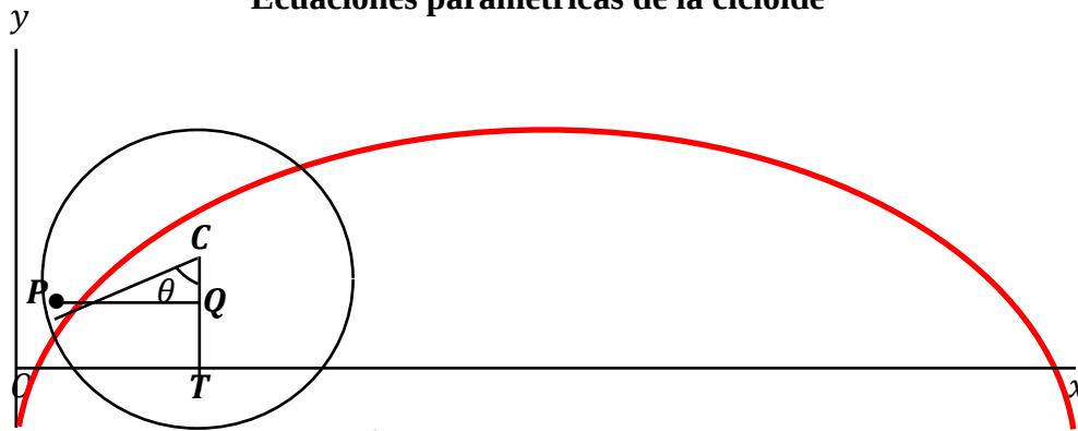
Ilustración 31: Ecuaciones de la cicloide
