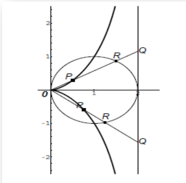
Ilustración 25: Cisoide de Diocles
