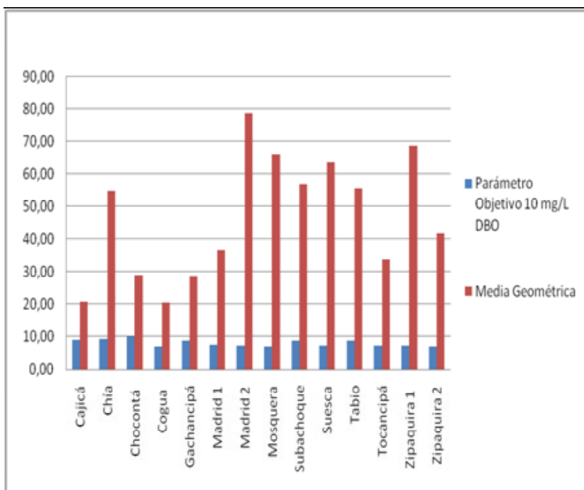
Figura 3. Parámetro Objetivo DBO para 10 mg/L Vs Media Geométrica
