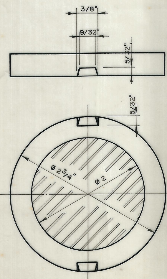
Detalle "A"
