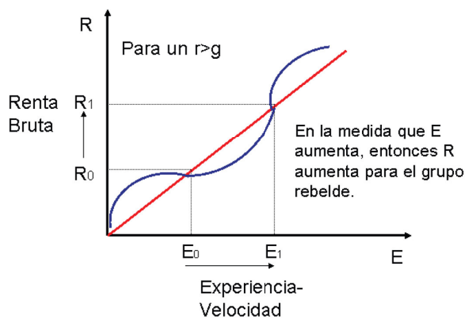
Grafica 1: Modelo de probabilidad de éxito de la fuerza rebelde.
