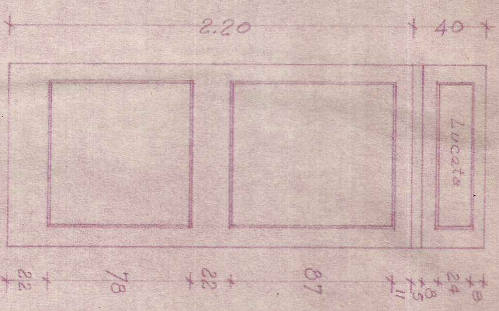
PUERTA TIPO 3
