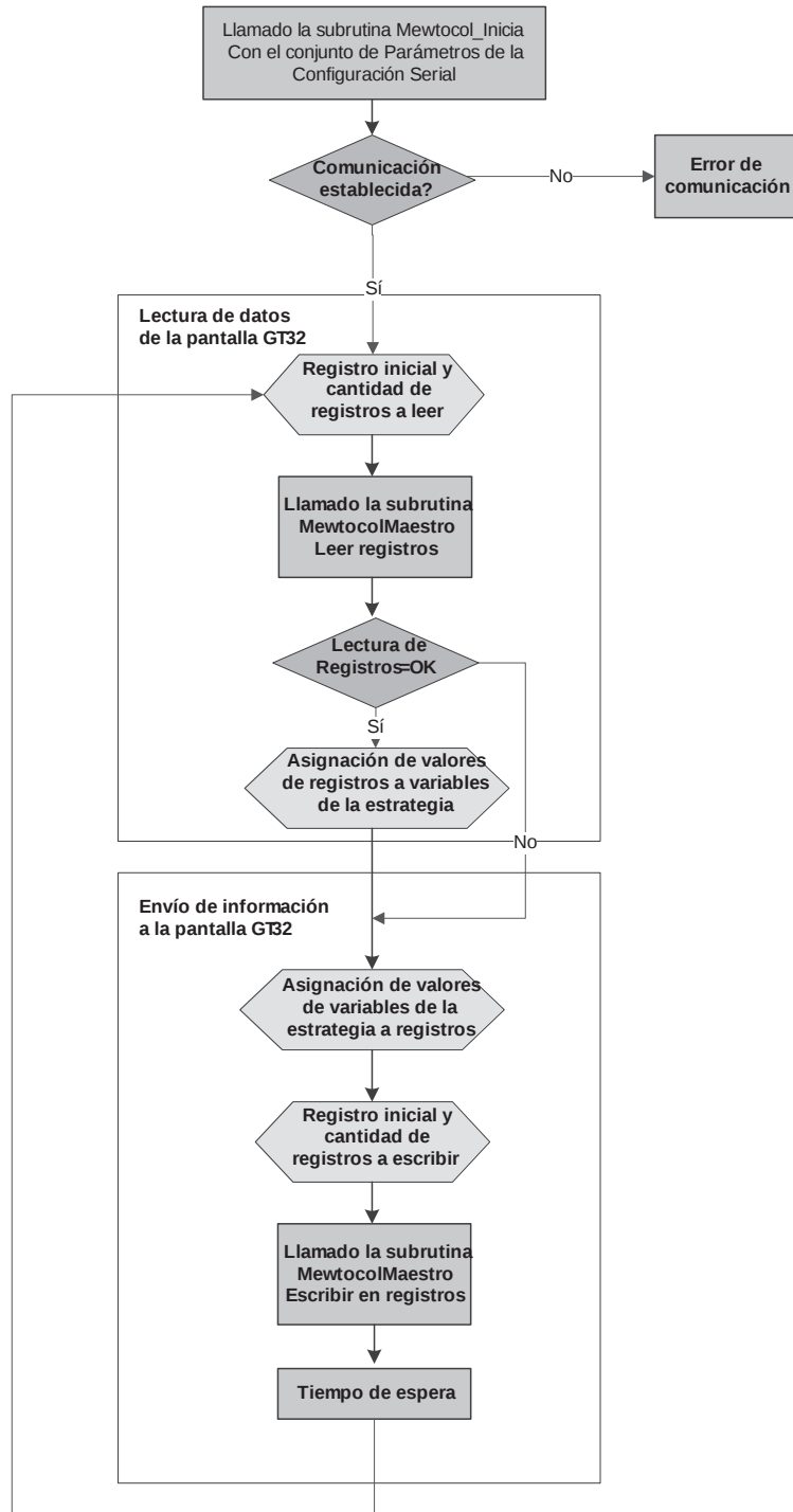
Figura 4.21 Diagrama MewtocolSerial
