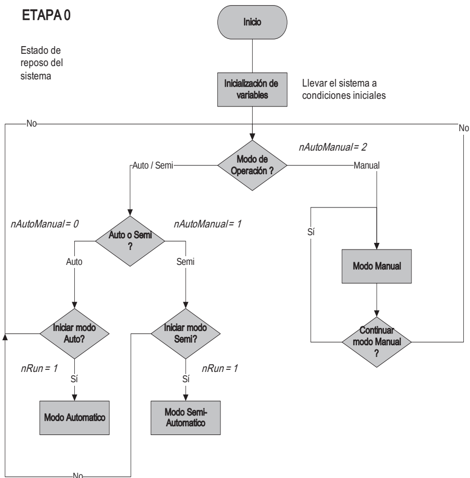
Figura 4.24 Diagrama inicio_secuencias
