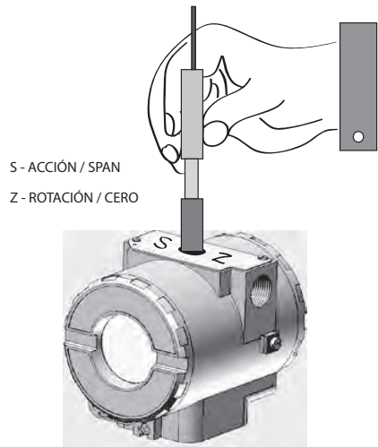
Figura 3.19 Ajuste local de cero y span [29]
