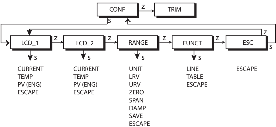
Figura 3.20 Rama CONF con las opciones para el ajuste [36]
