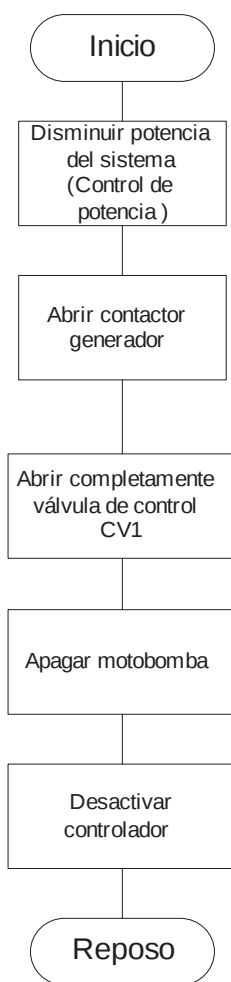
Figura 3.6 Secuencia de control para parada del SGEH
