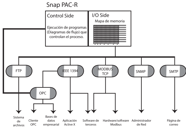
Figura 4.3 Opciones de comunicación con el Opto 22
