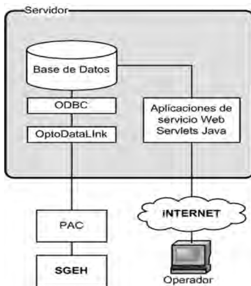
Figura 6.1 Esquema de la interfaz de comunicación
