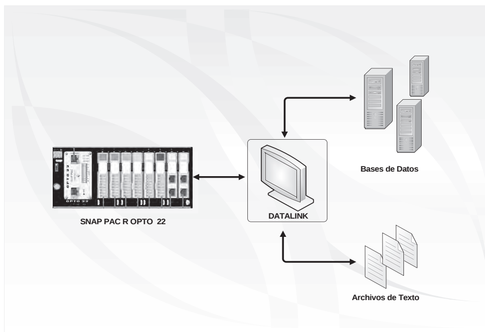
Figura 4.15 Posibilidades de comunicación utilizando OptoDataLink
