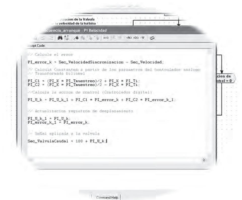
Figura 5.21 Implementación controlador PI usando OptoScript
