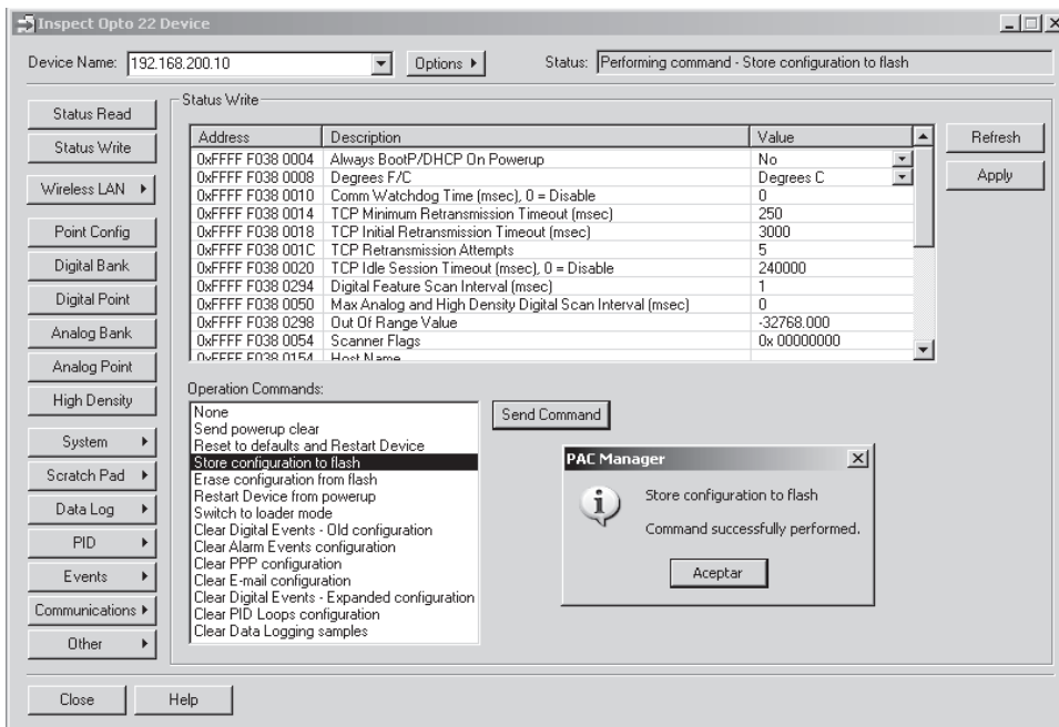
Figura 4.8. Grabar configuración en memoria flash
