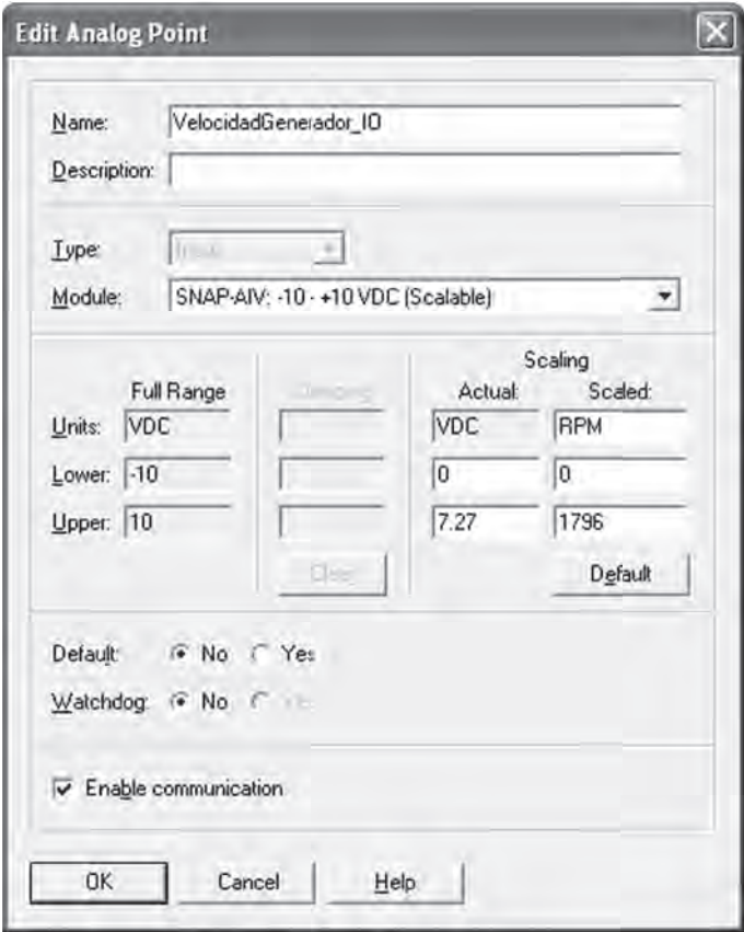
Figura 5.3 Escalado en la medición de velocidad usando el PAC Control para el Módulo SNAP-AIV -10/10V
