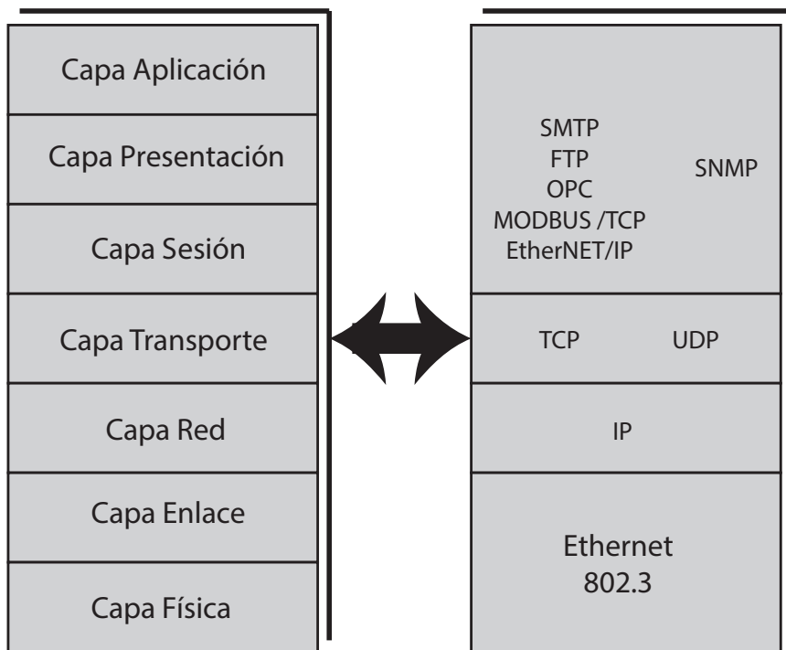
Figura 4.2. Opto 22. Protocolos
