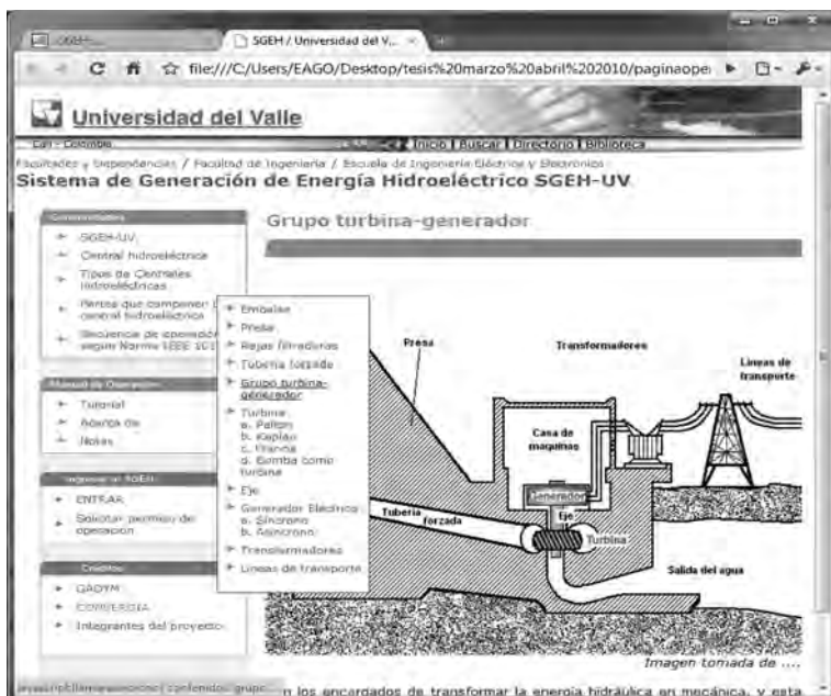
Figura 7.11 Partes que componen una central hidroeléctrica, grupo turbina-generator
