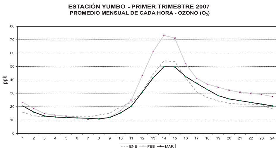
Gráfica 3.22. Promedio mensual de cada hora - Ozono (O 3 ) Estación Yumbo - primer trimestre 2007.
