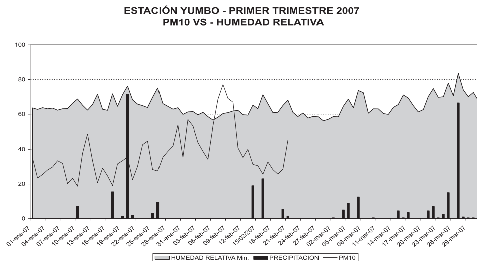
Gráfica 3.21. PM10 vs. humedad relativa Estación Yumbo - primer trimestre 2007
