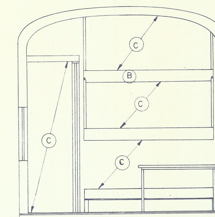
CORTE B-B
