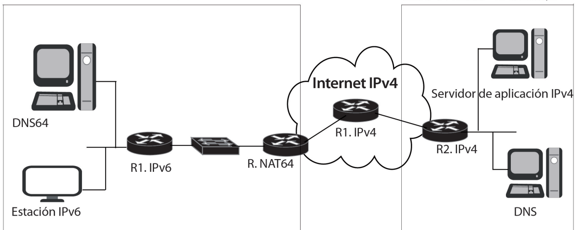
Figura 2. Funcionamiento del mecanismo NAT64 + DNS64.
