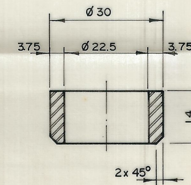
BUJE PARA PASADOR TIJERA
