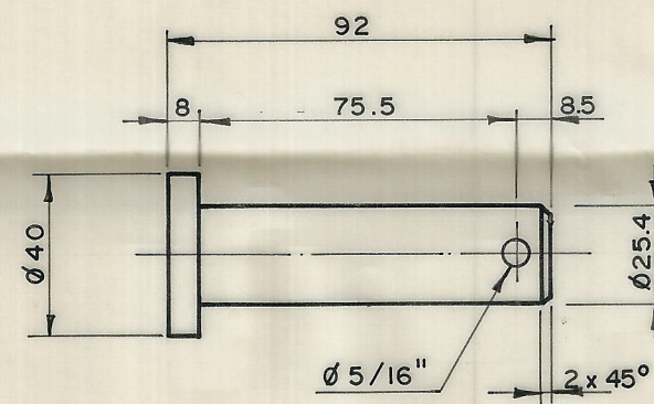
PASADOR PARA BIELA
