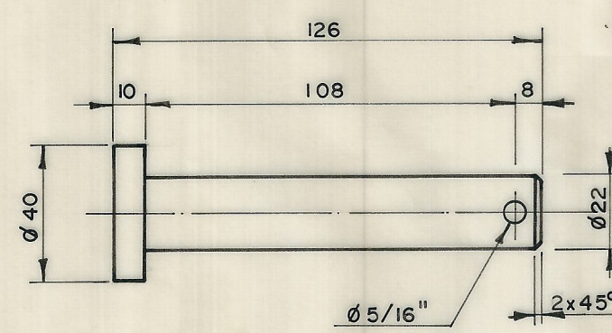
PASADOR PARA EJE DE BOGA CILINDRO FRENOS
