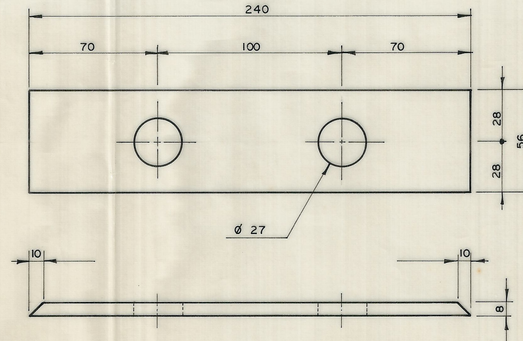
PLATINA PARA ZAPATA
