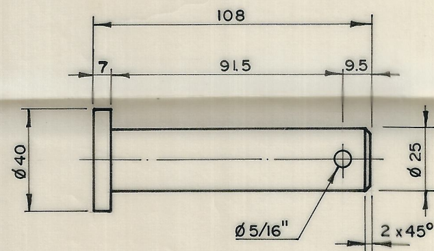
PASADOR TORNILLO TENSOR
