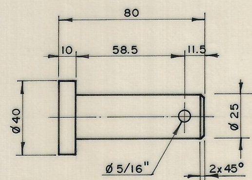
PASADOR PARA COLGANTE PORTAZAPATA
