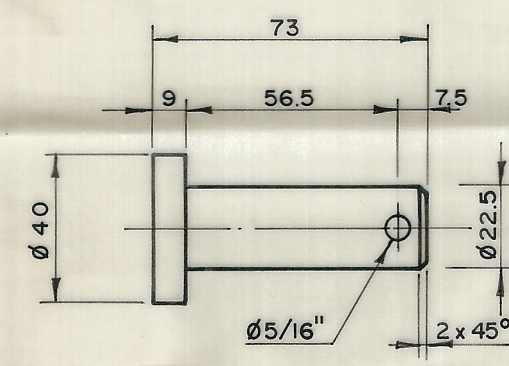
PASADOR PARA TIJERA
