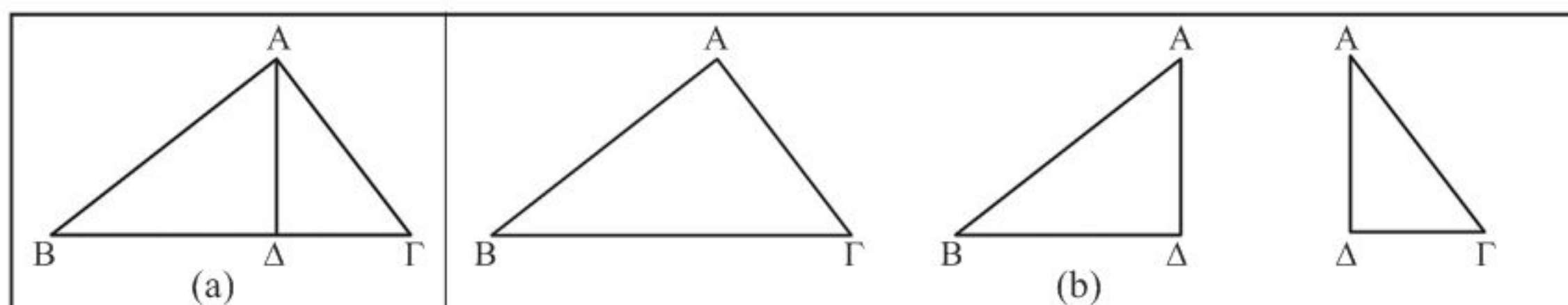
Ilustración 2. Tres triángulos semejantes
