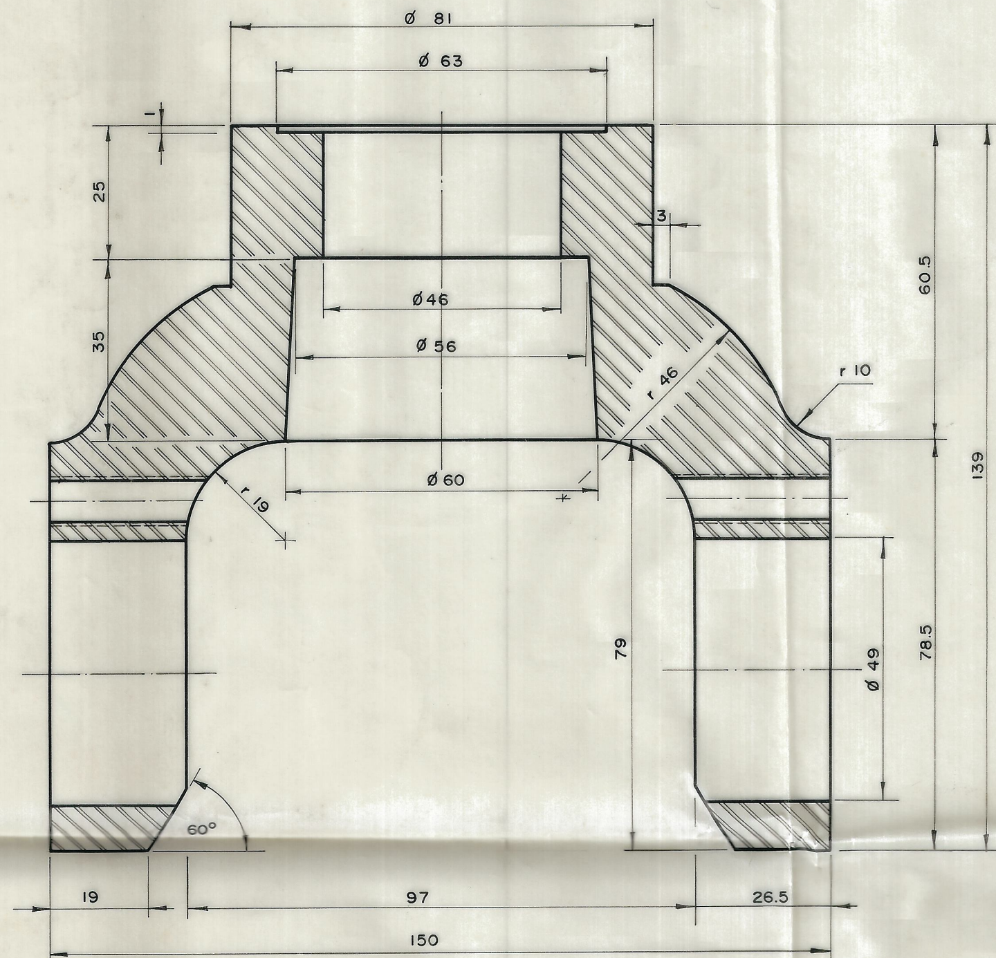
SECCION A-A'
