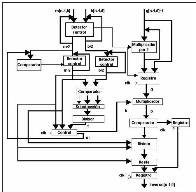
Figura 7. Arquitectura para el algoritmo binario
