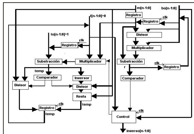
Figura 6. Arquitectura para el Algoritmo de Euclides
