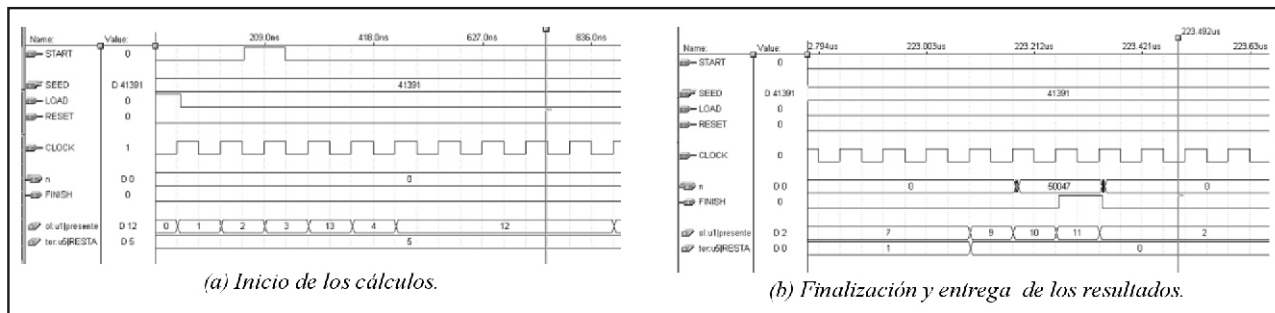
Figura 10. Resultados de la simulación del generador de números primos
