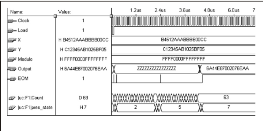
Figura 2. Simulación obtenida para el multiplicador de 65 Bits
