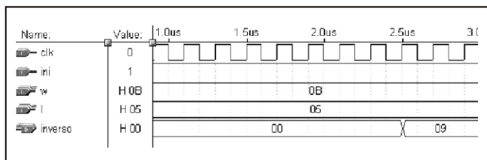
Figura 8. Resultados de la simulación para la arquitectura basada en el algoritmo de Euclides.
