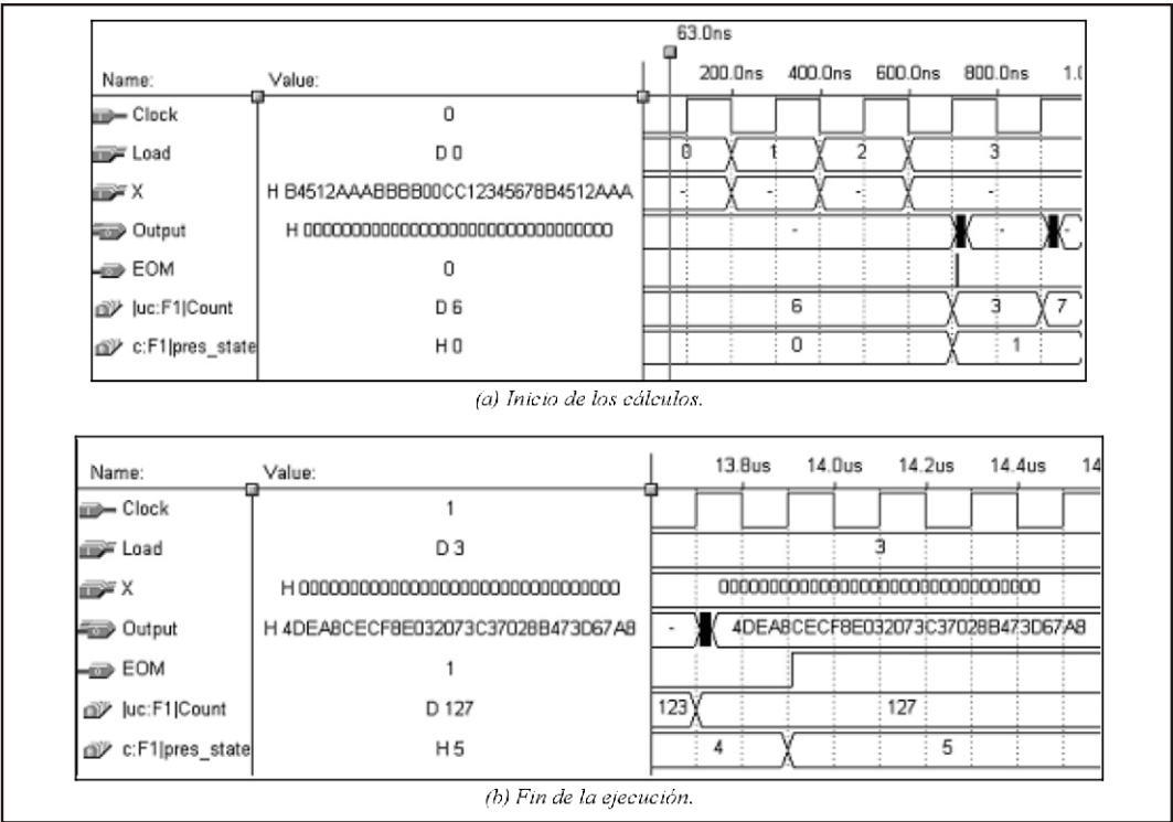
Figura 3. Simulación obtenida para el multiplicador de 128 Bits
