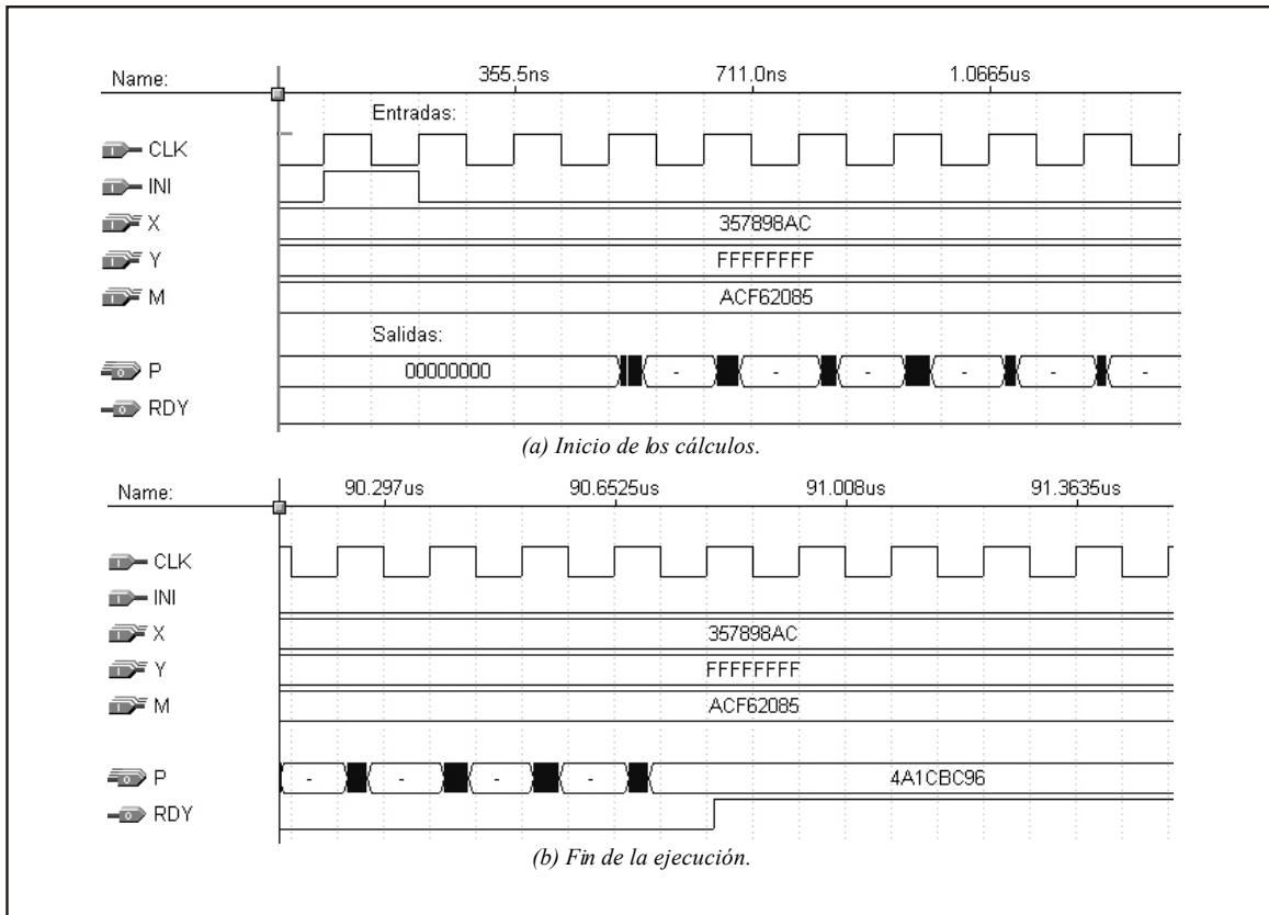
Figura 5. Simulación obtenida para el diseño final de la exponenciación modular
