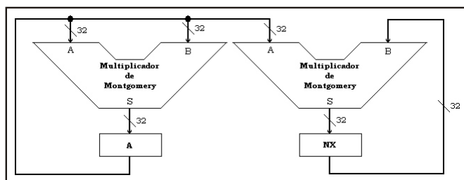
Figura 4. Ruta de datos simplificada del diseño POT3
