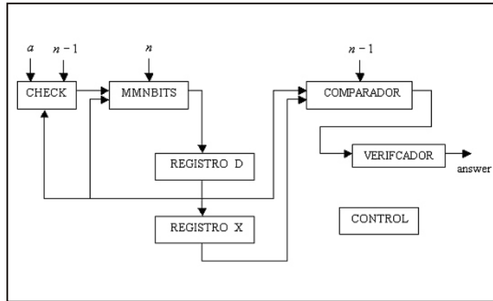
Figura 9. Diagrama de bloques para probador de primalidad
