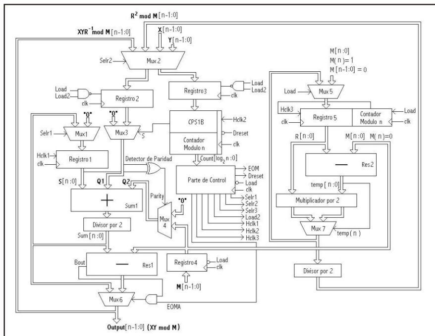
Figura 1. Diagrama Esquemático del Multiplicador de Montgomery para calcular x \cdot y \bmod M
