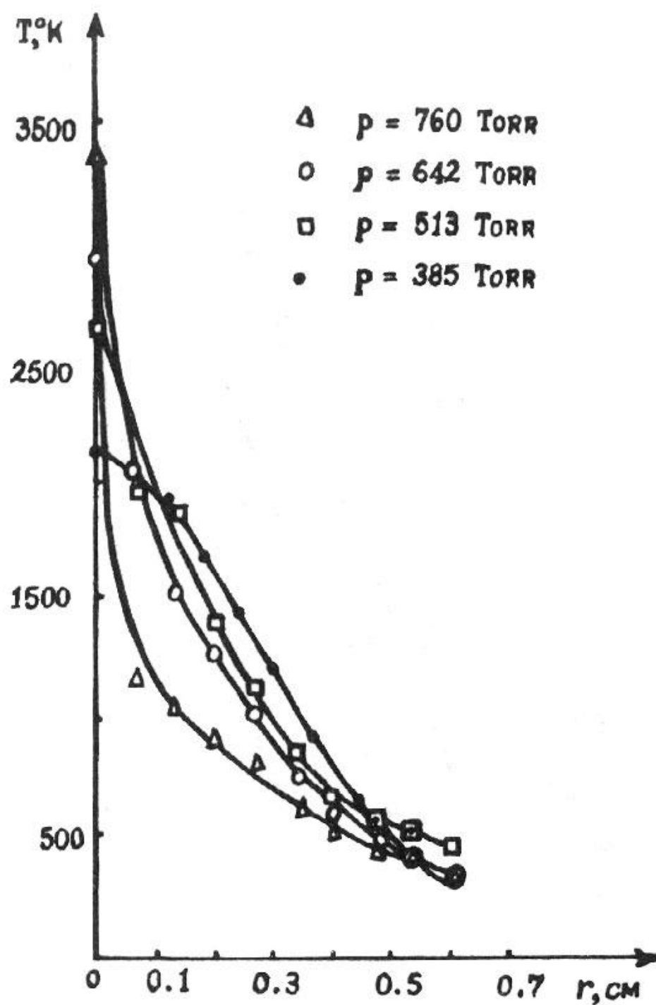
Fig. 4: Distribución de la temperatura cinética ( T_o ) en el canal de la descarga en dependencia de la presión gas: N_2 , \ell \simeq 1 CM.
