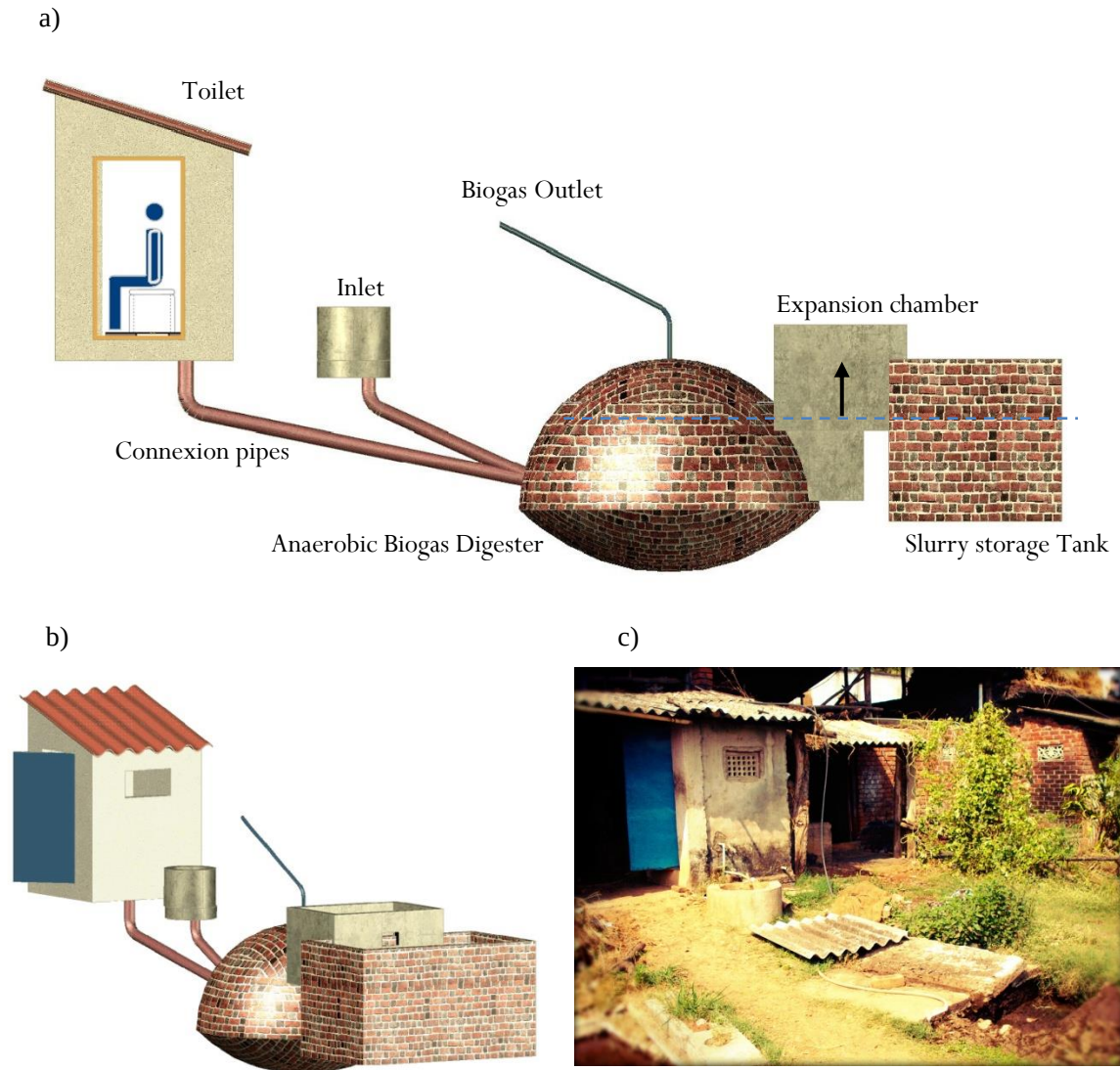
Figure ¡Error! No hay texto con el estilo especificado en el documento.-1 a) TLBP profile view. b) TLBP 3D view. c) TLBP selected
