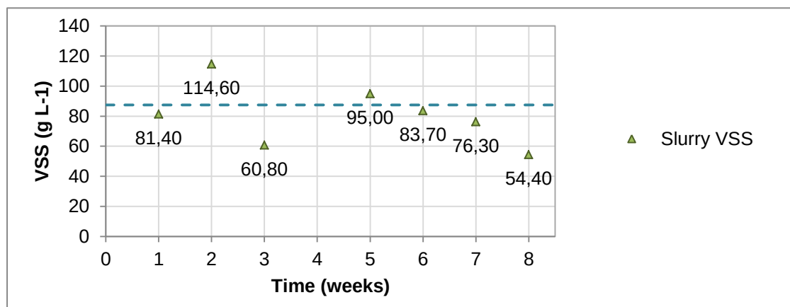
Figure ¡Error! No hay texto con el estilo especificado en el documento.-18 TLBP effluent's VSS and typical anaerobically digested sludge's VSS
