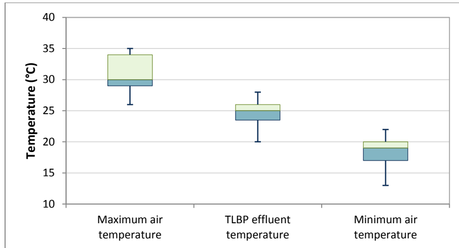
Figure ¡Error! No hay texto con el estilo especificado en el documento.-15 TLBP effluent temperature, maximum and minimum air temperatures
