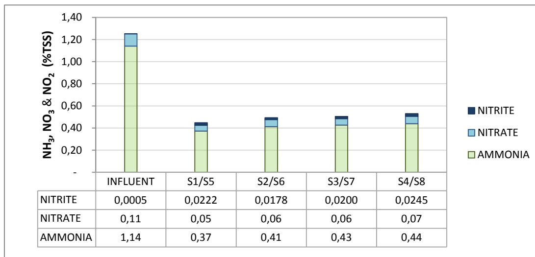
Figure ¡Error! No hay texto con el estilo especificado en el documento.-26 Influent and sludge treatment wetlands inorganic nitrogen composition
