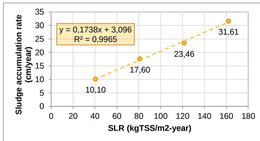
Figure ¡Error! No hay texto con el estilo especificado en el documento.-31 Sludge accumulation rates (cm/year)
