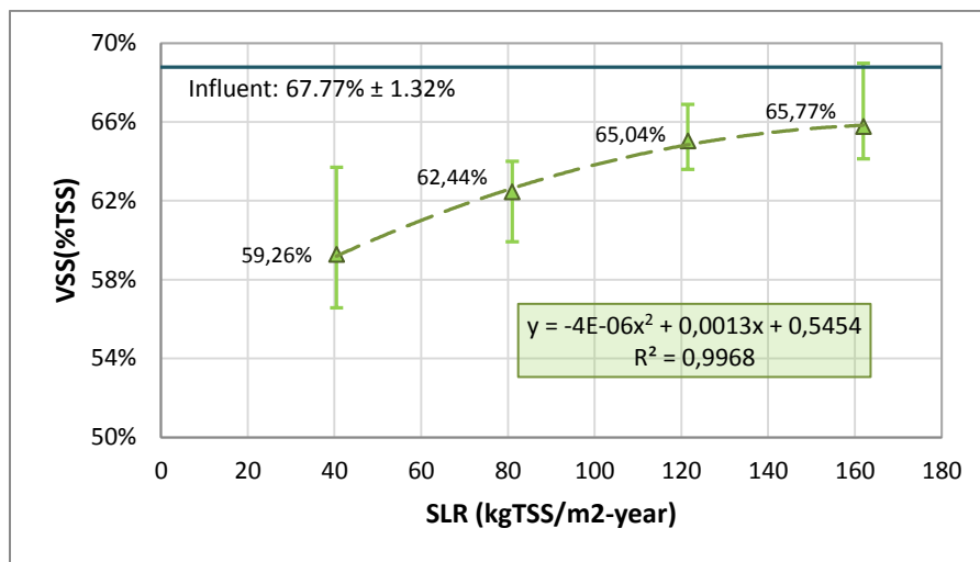
Figure ¡Error! No hay texto con el estilo especificado en el documento.-25 Sludge VSS (%TSS) reduction at different STWs
