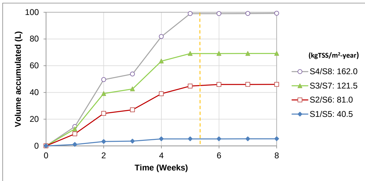
Figure ¡Error! No hay texto con el estilo especificado en el documento.-33 Water leachate accumulated volume at different loading rates
