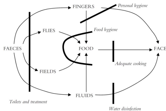
Figure ¡Error! No hay texto con el estilo especificado en el documento.-2 The F-diagram, showing the faecal disease transmission routes to a new host and the possible sanitation barriers
