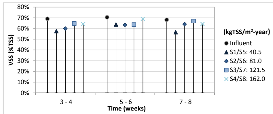
Figure ¡Error! No hay texto con el estilo especificado en el documento.-24 VSS concentration at the influent and its reduction at different loading rates
