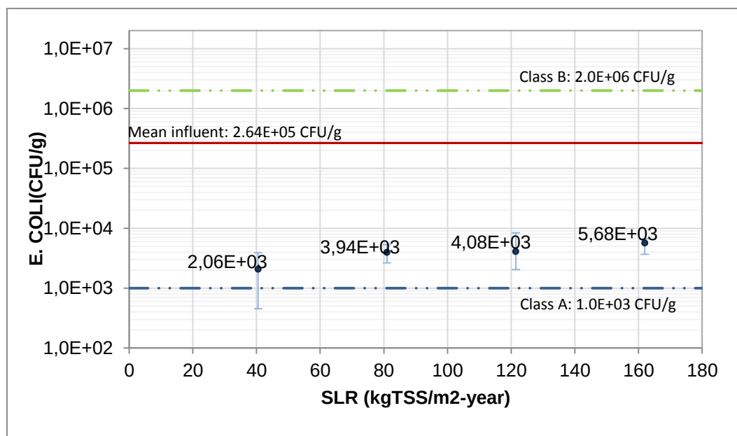
Figure ¡Error! No hay texto con el estilo especificado en el documento. -29 E. Coli concentration at different STWs and EPA limits for class A and B
