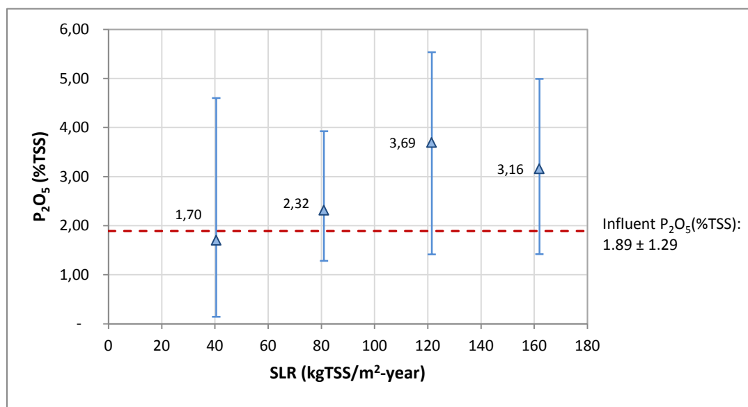
Figure ¡Error! No hay texto con el estilo especificado en el documento.-27 Influent and STWs phosphate concentrations
