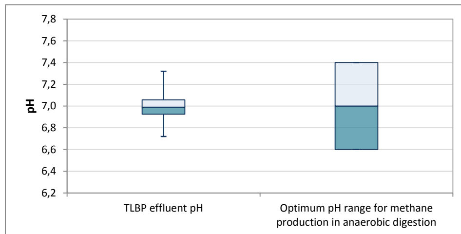
Figure ¡Error! No hay texto con el estilo especificado en el documento.-16 TLBP effluent pH and its recommended range for optimum growth of methane-producing microorganisms
