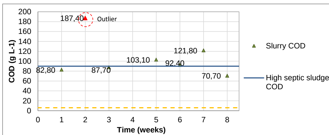
Figure ¡Error! No hay texto con el estilo especificado en el documento.-19 TLBP effluent's COD, high and low septic sludge COD concentrations
