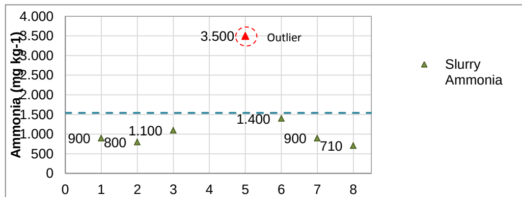
Figure ¡Error! No hay texto con el estilo especificado en el documento.-20 TLBP effluent ammonia and maximum ammonia concentration to avoid inhibition of methanogenesis
