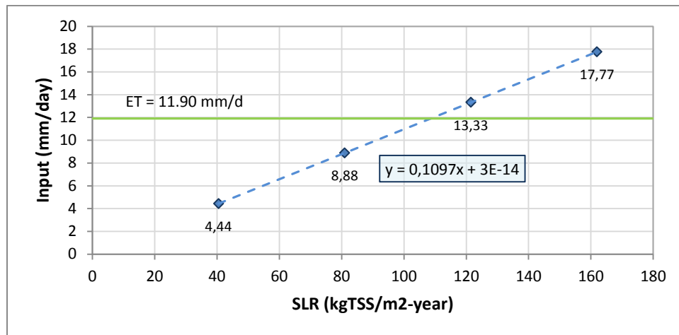
Figure ¡Error! No hay texto con el estilo especificado en el documento.-34 Volume of water fed daily at different SLRs
