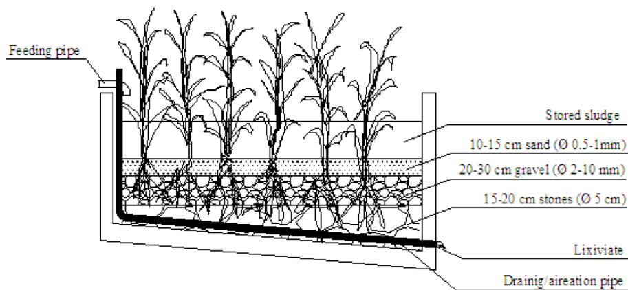
Figure ¡Error! No hay texto con el estilo especificado en el documento.-5 Schematic diagram of a sludge treatment wetland Source: Uggetti et al. (2010)
