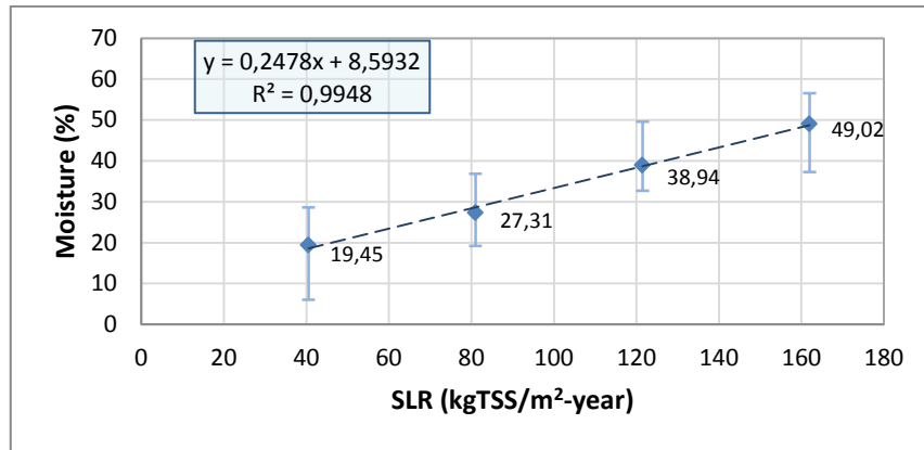
Figure ¡Error! No hay texto con el estilo especificado en el documento.-23 STW dried sludge moisture content under different loading rates
