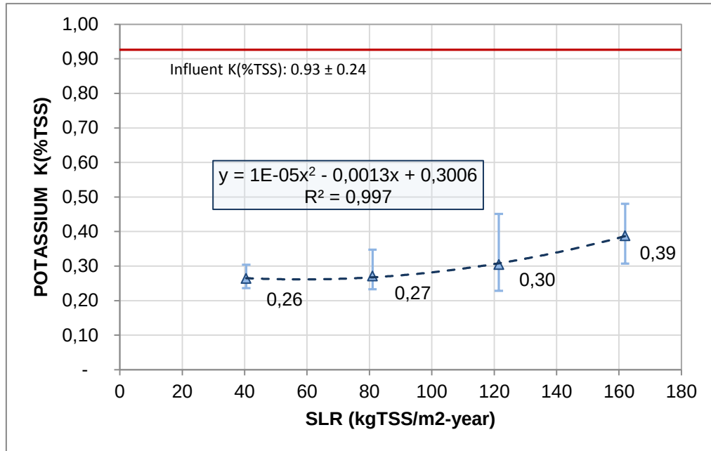
Figure ¡Error! No hay texto con el estilo especificado en el documento.-28 Influent and STWs potassium concentrations
