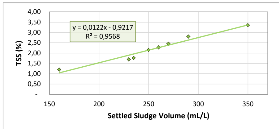
Figure ¡Error! No hay texto con el estilo especificado en el documento.-22 Correlation TLBP effluent TSS (%) vs. Settled Sludge Volume (mL/L)
