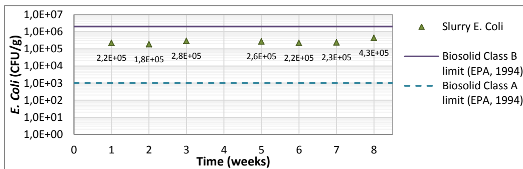
Figure ¡Error! No hay texto con el estilo especificado en el documento.-21 TLBP effluent E. Coli CFU/g (dry-weight basis) & biosolid class A and B limits (EPA, 1994)
