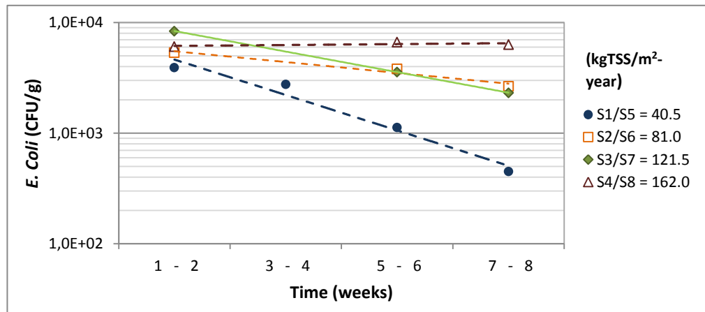
Figure ¡Error! No hay texto con el estilo especificado en el documento.-30 Pathogen reduction during the first two months of system implementation
