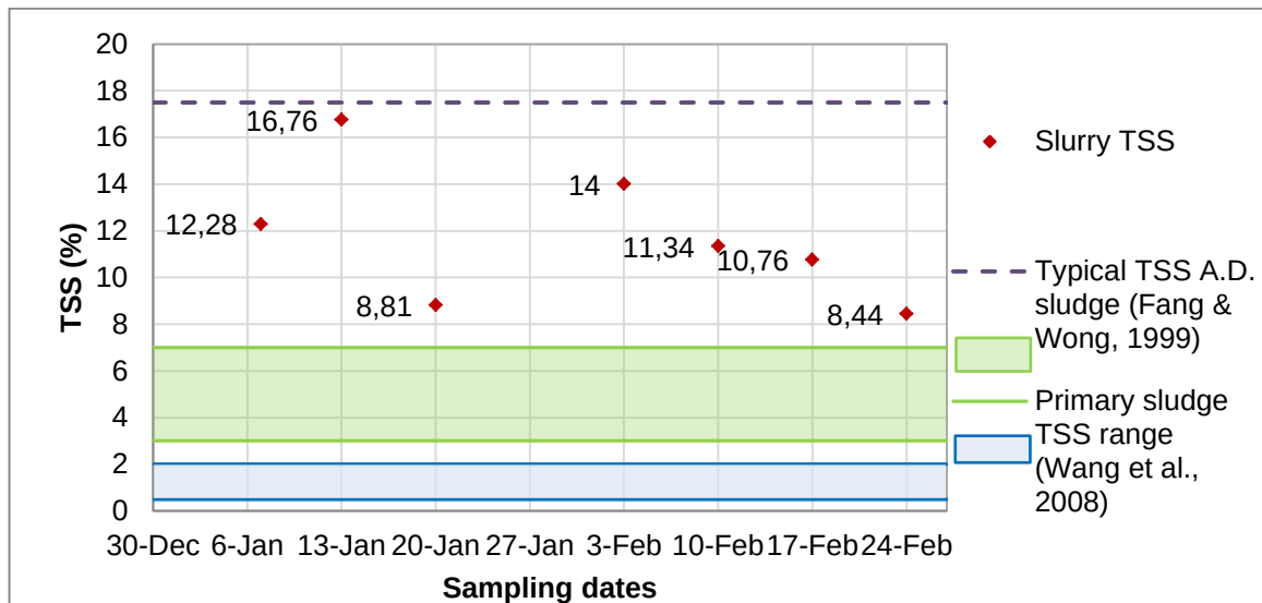
Figure ¡Error! No hay texto con el estilo especificado en el documento.-17 TLBP effluent's TSS, primary and secondary TSS ranges and typical anaerobically digested sludge TSS
